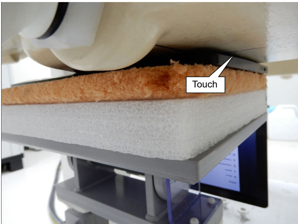
EUT Bottom_WWAN_0mm
