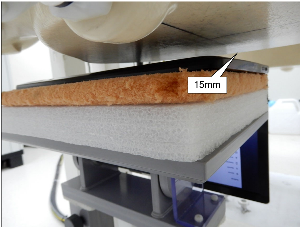
EUT Bottom_WWAN_15mm
