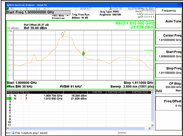
Band2 / 1.4MHz / High CH / QPSK / 1 RB
