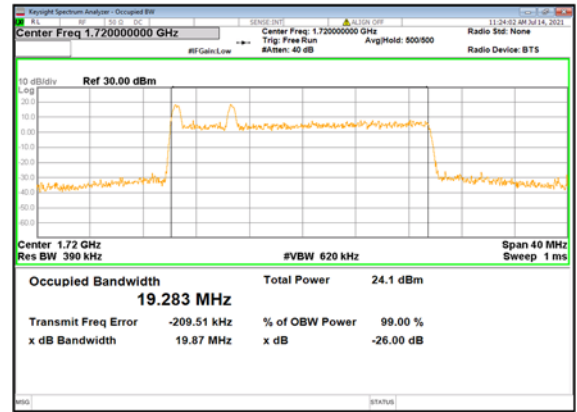
n66(20M)_CP-OFDM_ QPSK_Outer_Full_Low_CH
