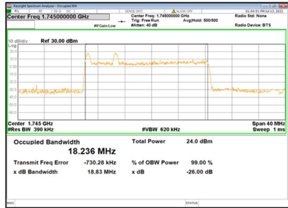
n66(20M)_CP-OFDM_ QPSK_Outer_Full_Mid_CH
