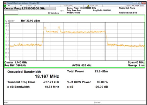
n66(20M)_DFT-s-OFDM_ QPSK_Outer_Full_Mid_CH
