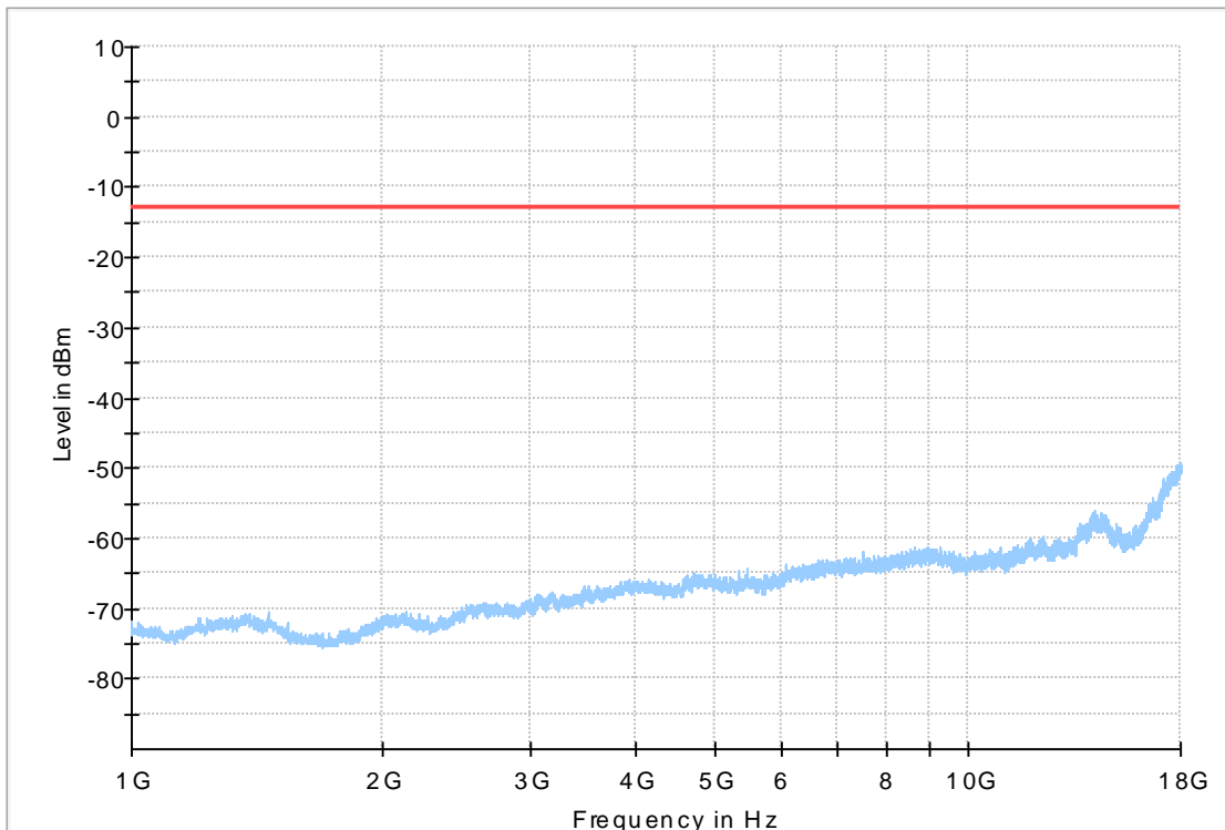
1GHz-18GHz
