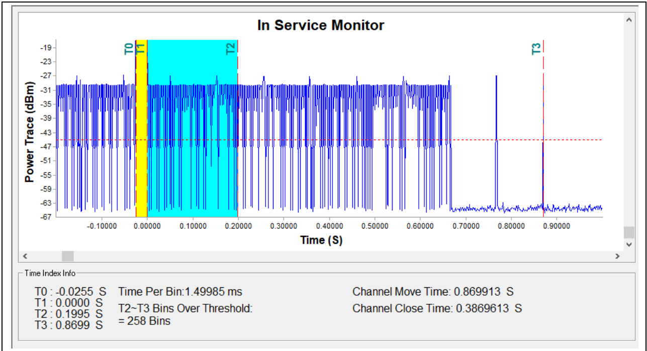
(5600MHz, 802.11a)
