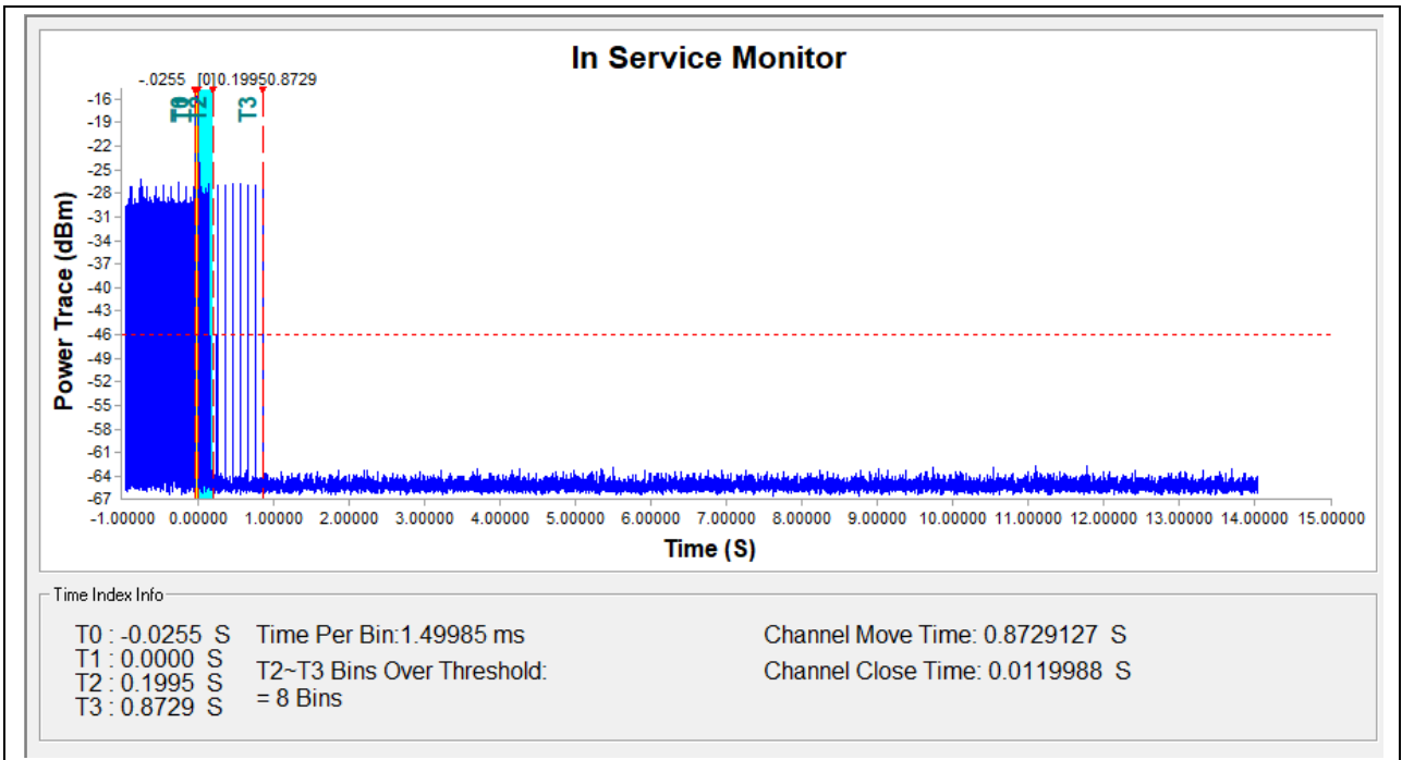
(5320MHz, 802.11a)
