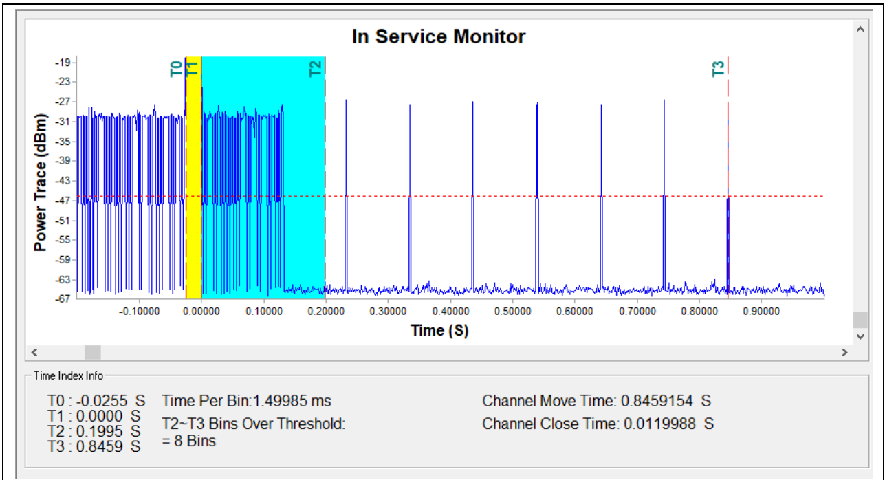
(5300MHz, 802.11a)
