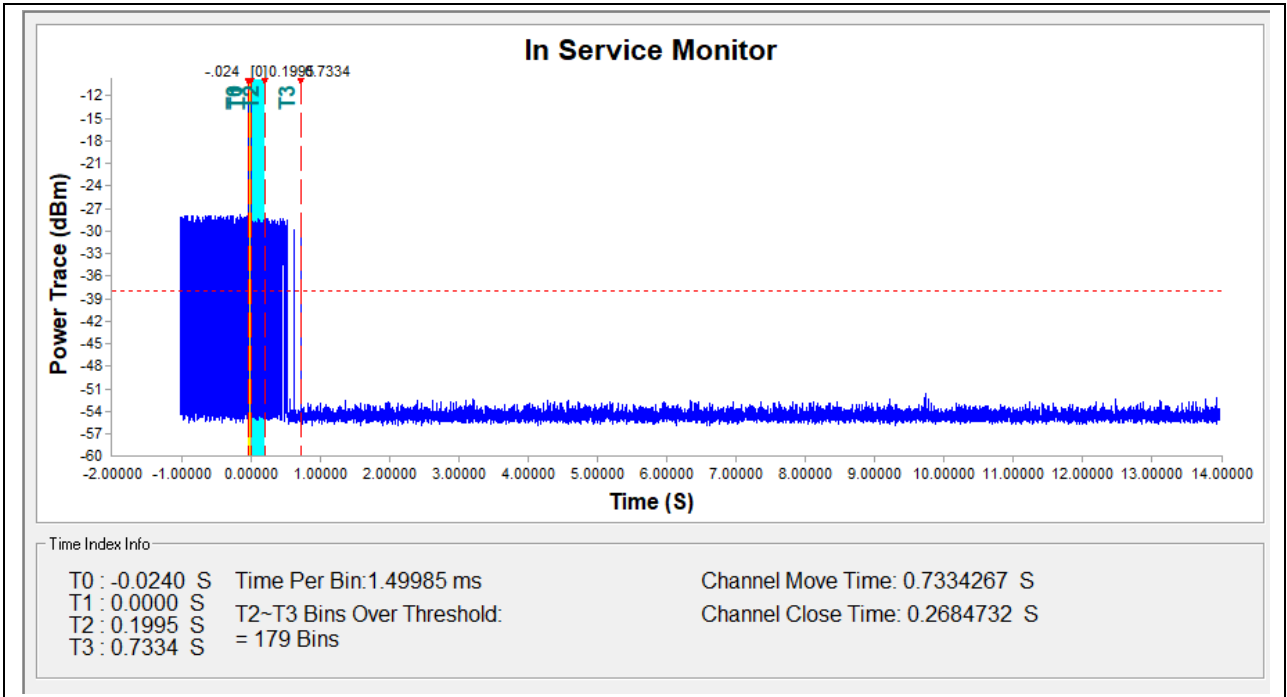
(5620MHz, 802.11a)
