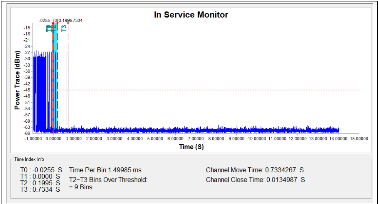
(5580MHz, 802.11a)
