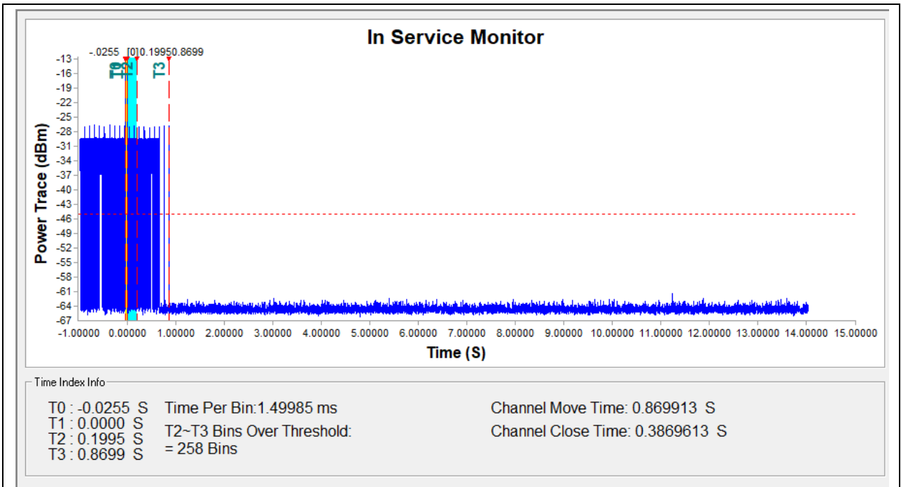
(5600MHz, 802.11a)
