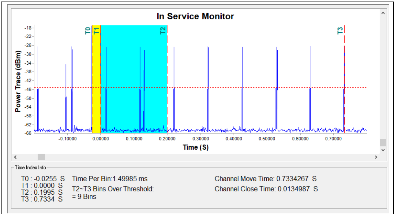
(5580MHz, 802.11a)
