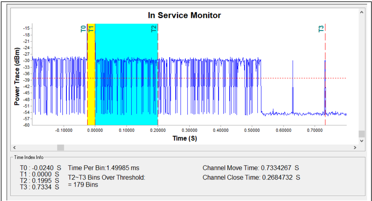
(5620MHz, 802.11a)
