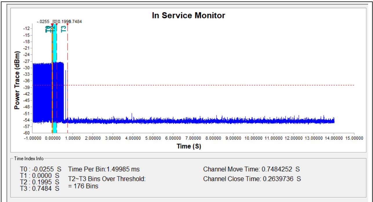
(5640MHz, 802.11a)
