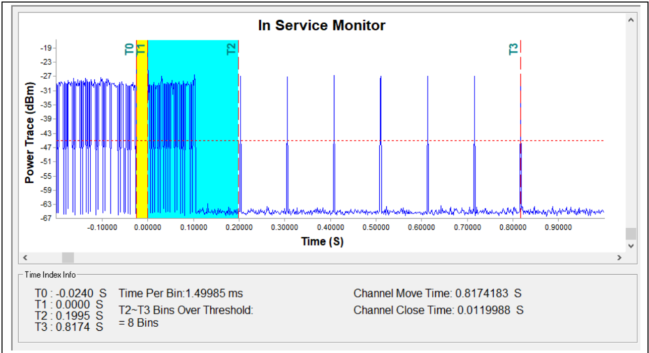
(5280MHz, 802.11a)
