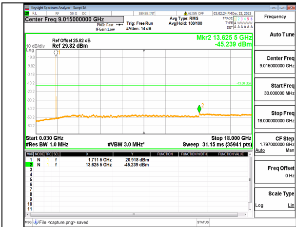
n66 (30MHz-18GHz) 15M DFT-s-OFDM BPSK Inner_1RB_Left Low
