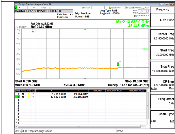
n66 (30MHz-18GHz) 15M DFT-s-OFDM QPSK Inner_1RB_Left Low
