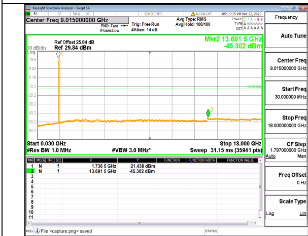
n66 (30MHz-18GHz) 20M DFT-s-OFDM BPSK Inner_1RB_Left Mid
