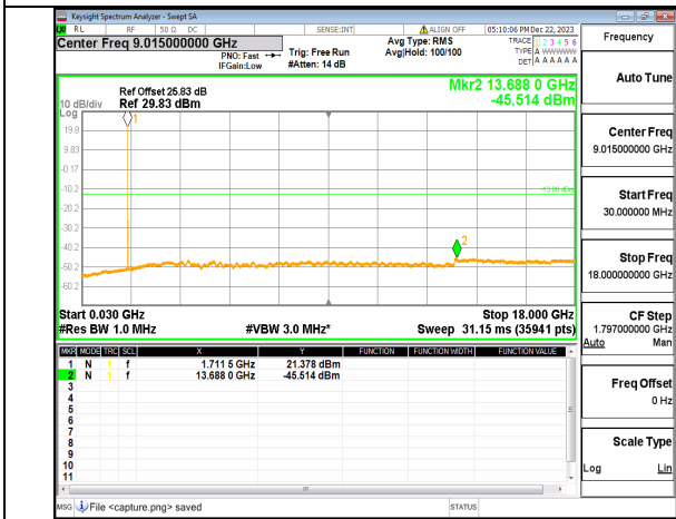
n66 (30MHz-18GHz) 20M DFT-s-OFDM QPSK Inner_1RB_Left Low
