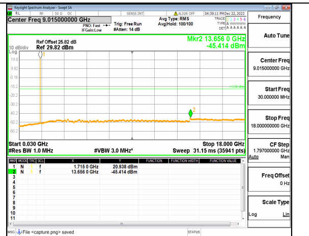
n66 (30MHz-18GHz) 5M DFT-s-OFDM QPSK Inner_1RB_Right Low
