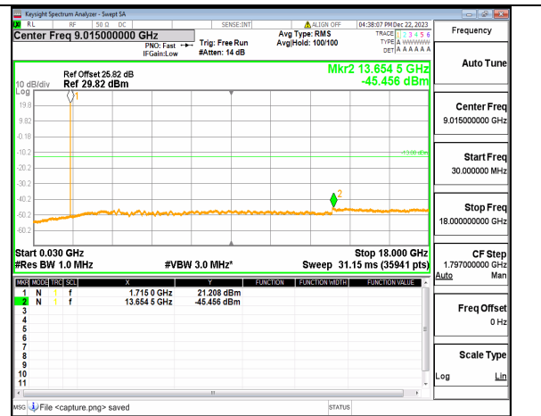
n66 (30MHz-18GHz) 5M DFT-s-OFDM BPSK Inner_1RB_Right Low
