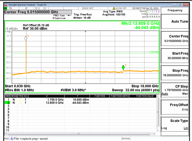
66B / 10+5MHz / QPSK / Mid CH / 50@0-25@
