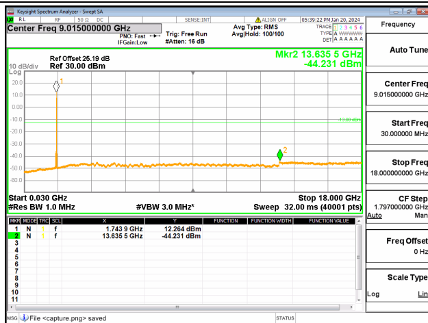
66C / 15+10MHz / QPSK / Mid CH / 1@0-1@49
