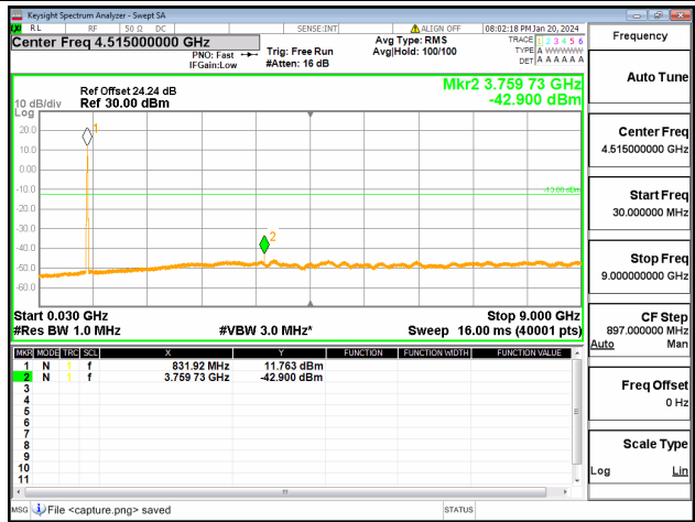
5B / 10+10MHz / QPSK / Mid CH / 50@0-50@0
