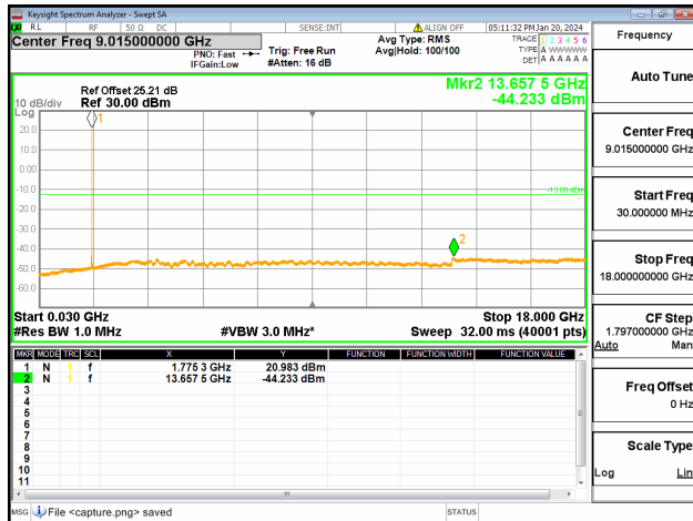
66B / 10+5MHz / QPSK / High CH / 1@49-1@0
