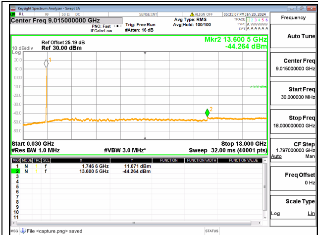
66C / 10+20MHz / QPSK / Mid CH / 50@0-100@0
