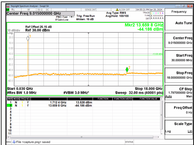
66B / 5+15MHz / QPSK / Low CH / 25@0-75@0
