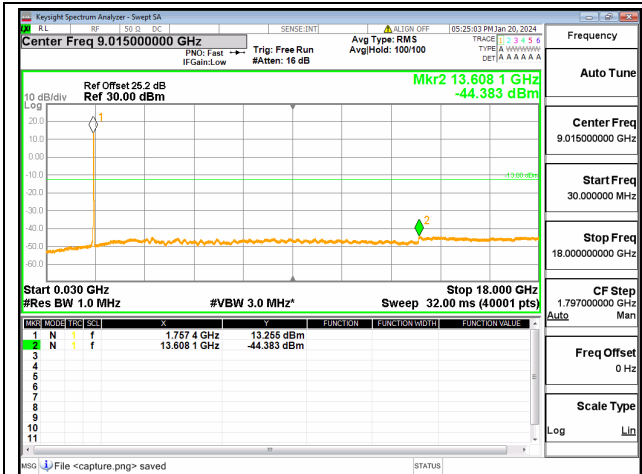
66C / 5+20MHz / QPSK / High CH / 25@0-100@0
