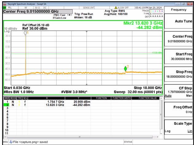
66C / 15+15MHz / QPSK / Mid CH / 1@74-1@0
