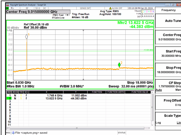
66B / 10+10MHz / QPSK / Mid CH / 50@0-50@
