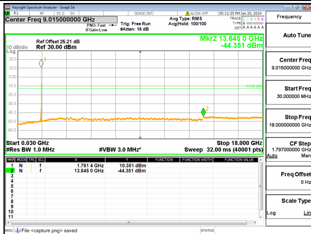
66B / 10+10MHz / QPSK / High CH / 1@0-1@49
