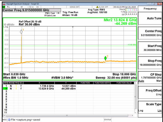
66C / 15+20MHz / QPSK / Mid CH / 1@0-1@99
