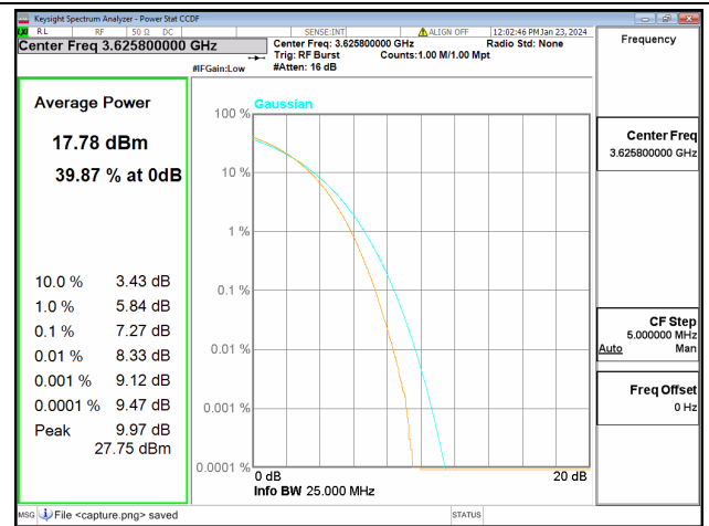
48C / 5+20MHz / Mid CH / 256QAM
