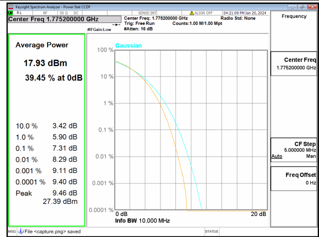
66B / 5+5MHz / High CH / 256QAM
