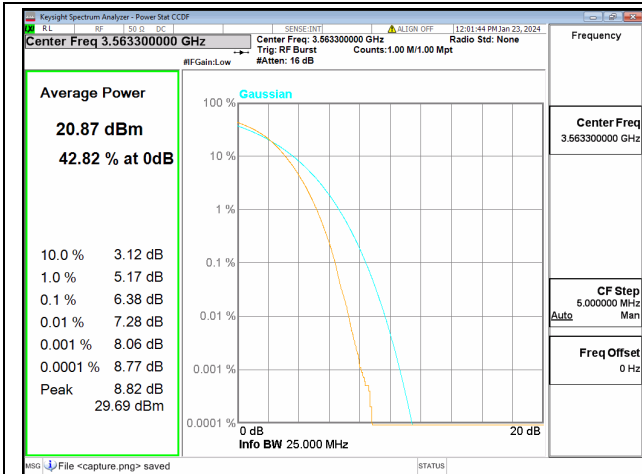
48C / 5+20MHz / Low CH / QPSK
