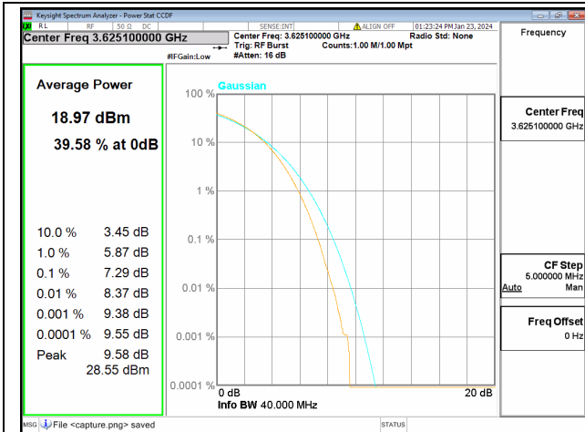
48C / 20+20MHz / Mid CH / 64QAM
