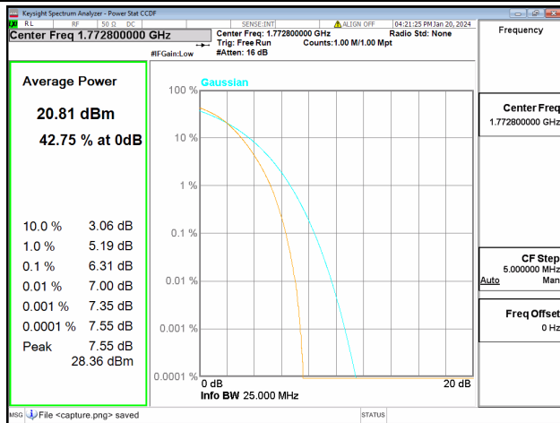
66B / 5+10MHz / High CH / QPSK
