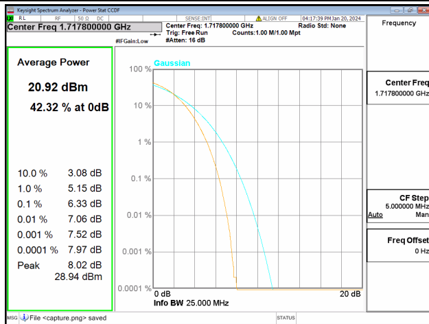
66B / 5+10MHz / Low CH / QPSK
