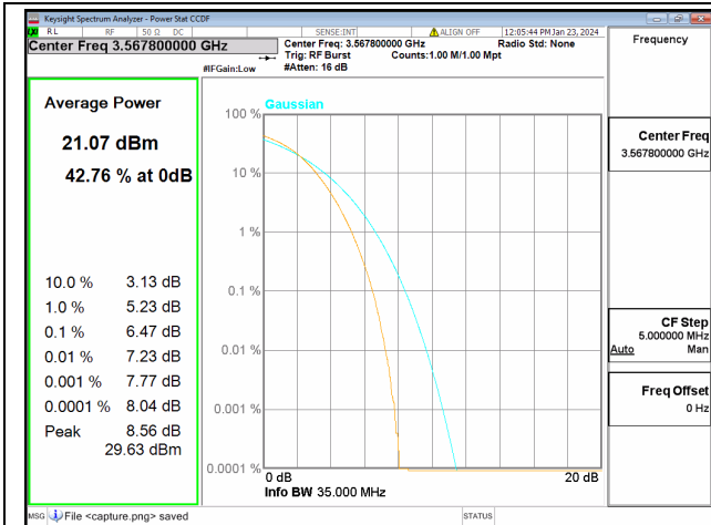
48C / 15+20MHz / Low CH / QPSK
