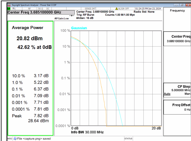
48C / 20+10MHz / High CH / QPSK
