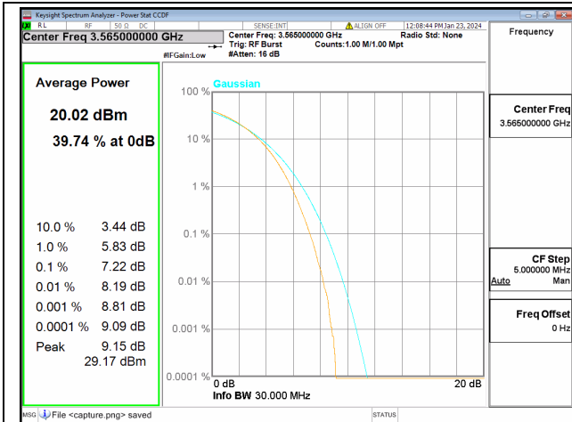
48C / 20+10MHz / Low CH / 64QAM
