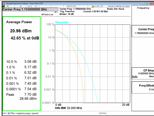
66B / 5+15MHz / Mid CH / QPSK
