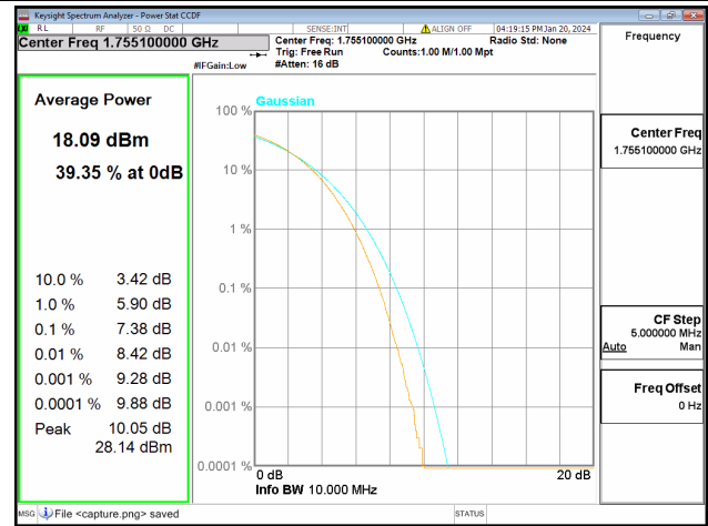
66B / 5+5MHz / Mid CH / 256QAM
