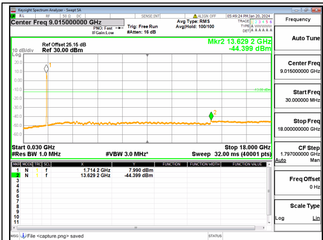
66C / 20+10MHz / QPSK / Low CH / 100@0-50@0
