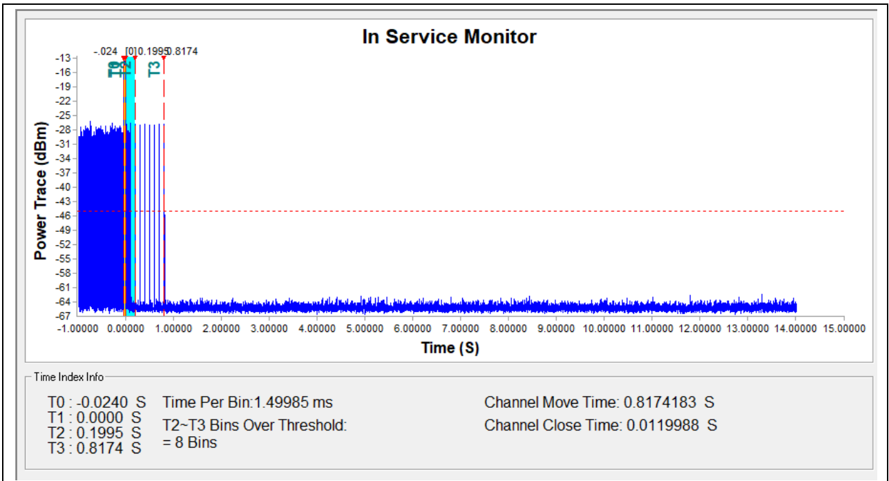
(5280MHz, 802.11a)
