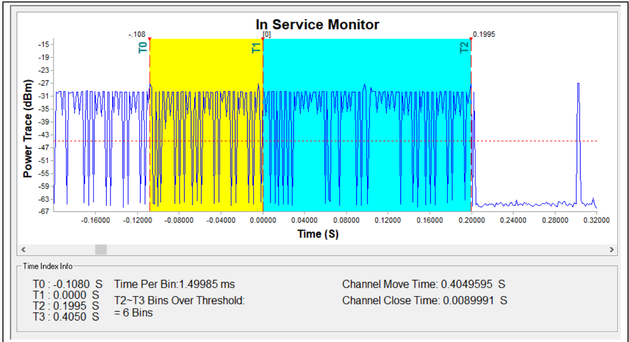
(5600MHz, 802.11a)
