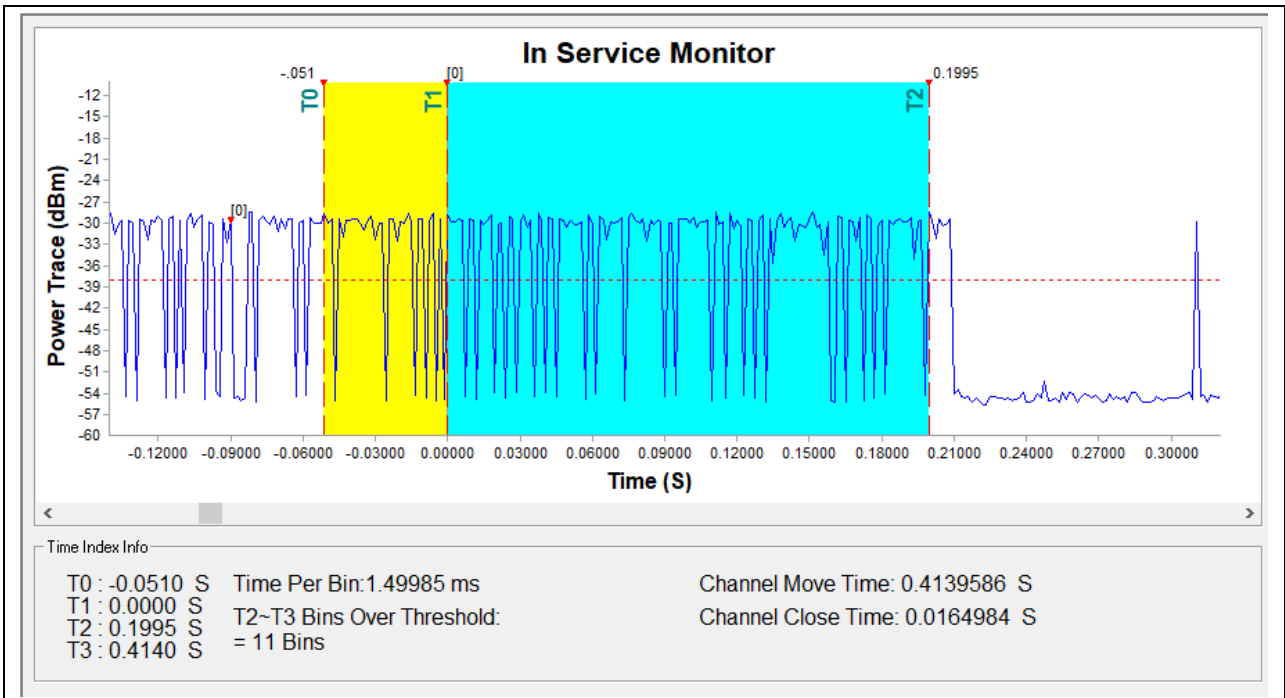
(5620MHz, 802.11a)
