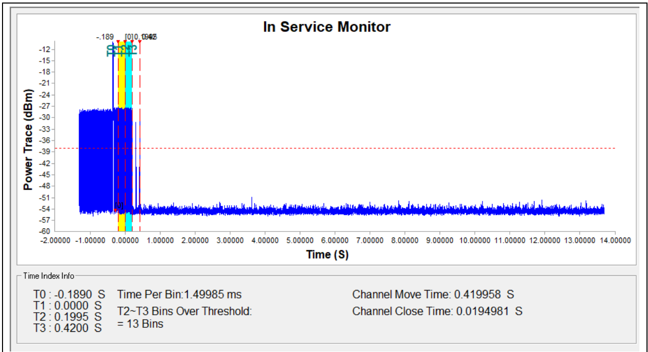
(5640MHz, 802.11a)
