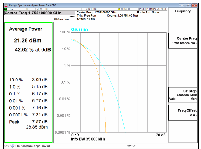
66C / 20+15MHz / Mid CH / QPSK
