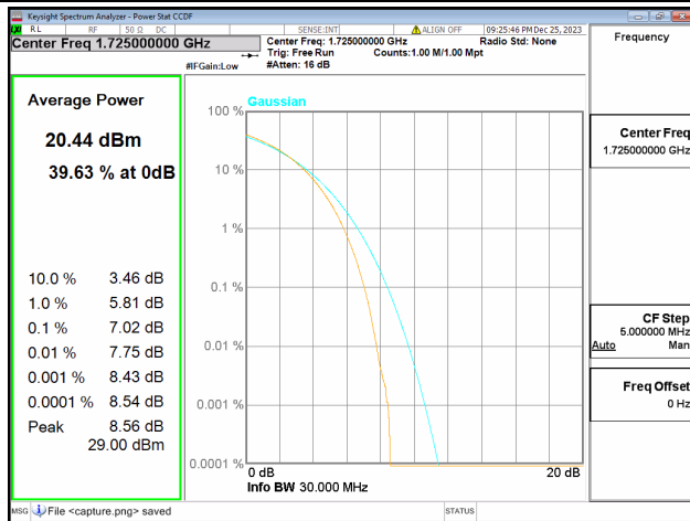
66C / 20+10MHz / Low CH / QPSK
