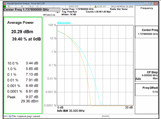
66C / 15+20MHz / Low CH / 64QAM
