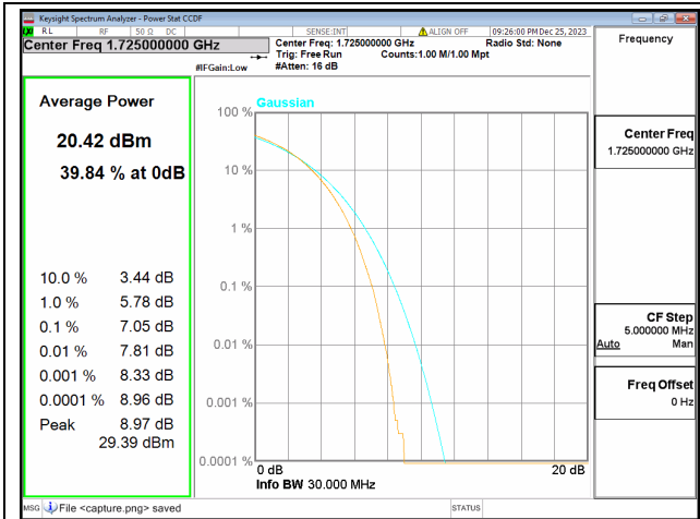
66C / 20+10MHz / Low CH / 64QAM
