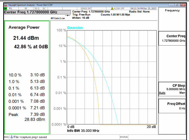
66C / 15+20MHz / Low CH / QPSK
