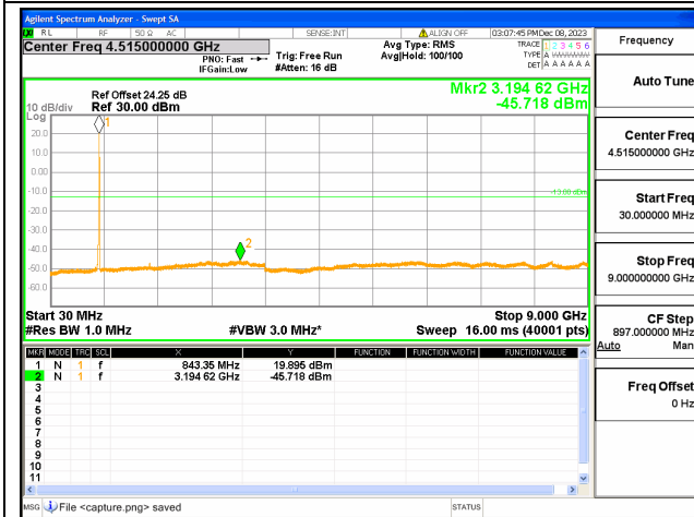
5B / 3+5MHz / QPSK / High CH / 15@0-25@0
