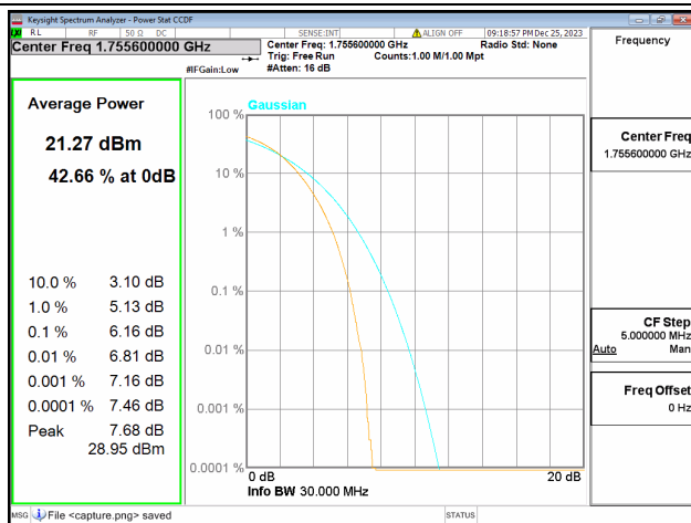
66C / 10+20MHz / Mid CH / QPSK
