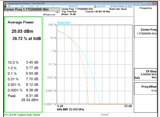
66B / 15+5MHz / High CH / 64QAM
