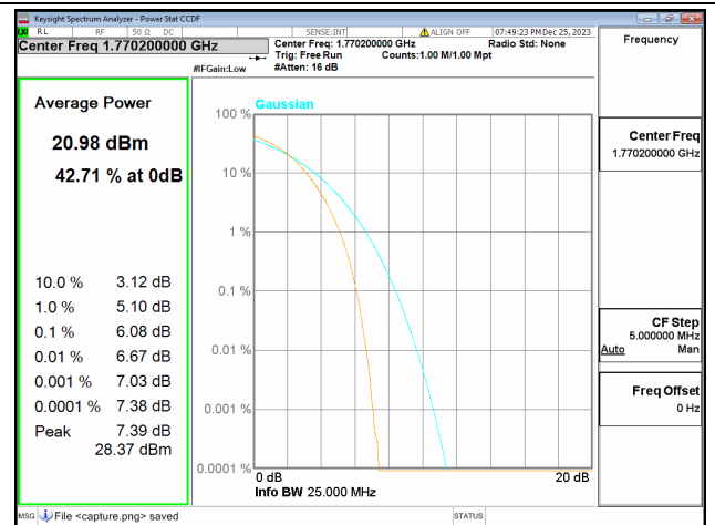
66B / 15+5MHz / High CH / QPSK
