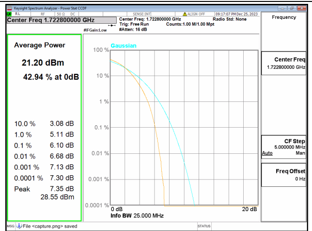
66C / 10+15MHz / Low CH / QPSK
