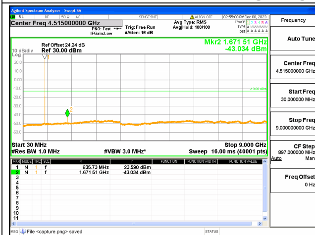
5B / 3+5MHz / QPSK / Mid CH / 1@14-1@0
