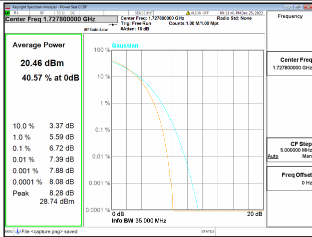
66C / 15+20MHz / Low CH / 16QAM
