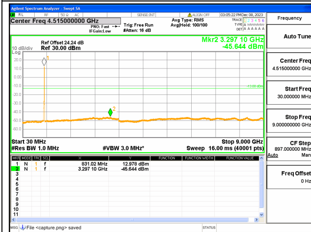
5B / 10+5MHz / QPSK / Mid CH / 50@0-25@0
