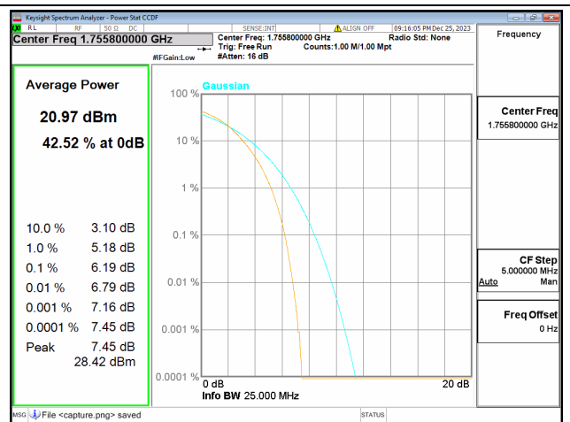
66C / 5+20MHz / Mid CH / QPSK
