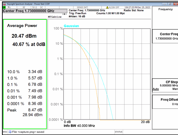
66C / 20+20MHz / Low CH / 16QAM
