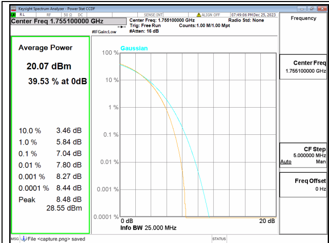
66B / 15+5MHz / Mid CH / 64QAM
