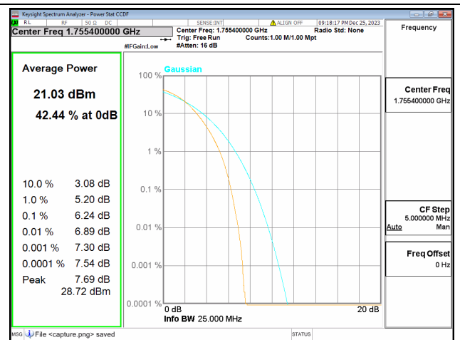
66C / 10+15MHz / Mid CH / QPSK
