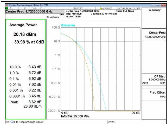
66C / 5+20MHz / Low CH / 64QAM
