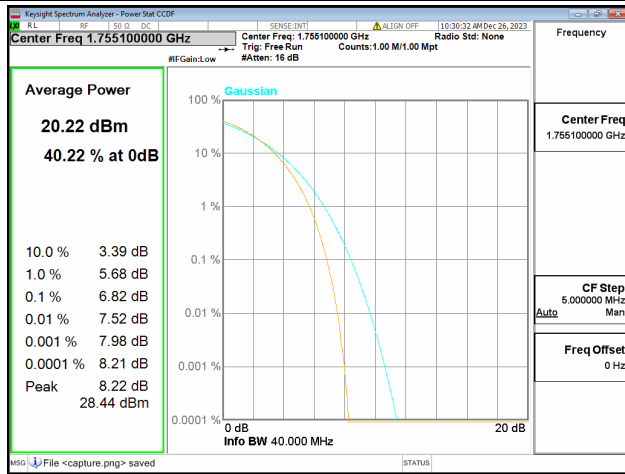
66C / 20+20MHz / Mid CH / 16QAM
