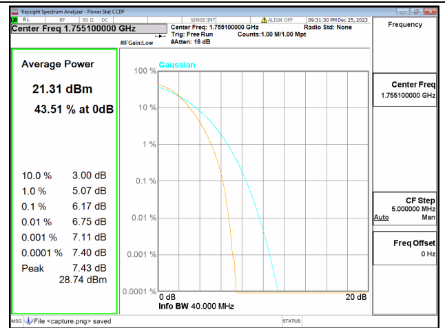
66C / 20+20MHz / Mid CH / QPSK
