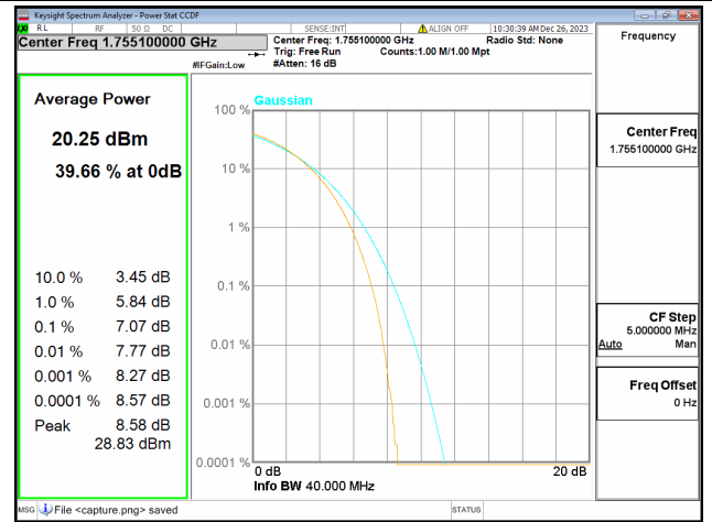
66C / 20+20MHz / Mid CH / 64QAM
