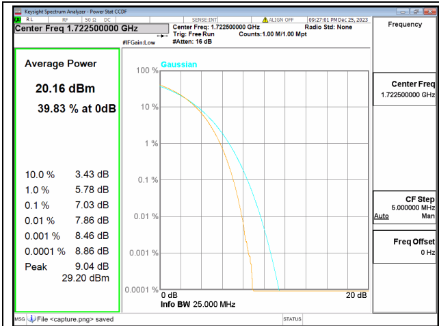
66C / 20+5MHz / Low CH / 64QAM
