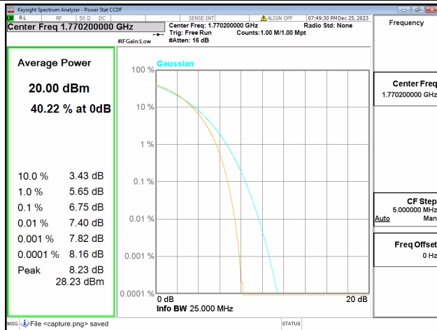
66B / 15+5MHz / High CH / 16QAM
