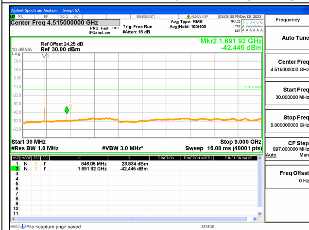
5B / 5+3MHz / QPSK / High CH / 1@24-1@0
