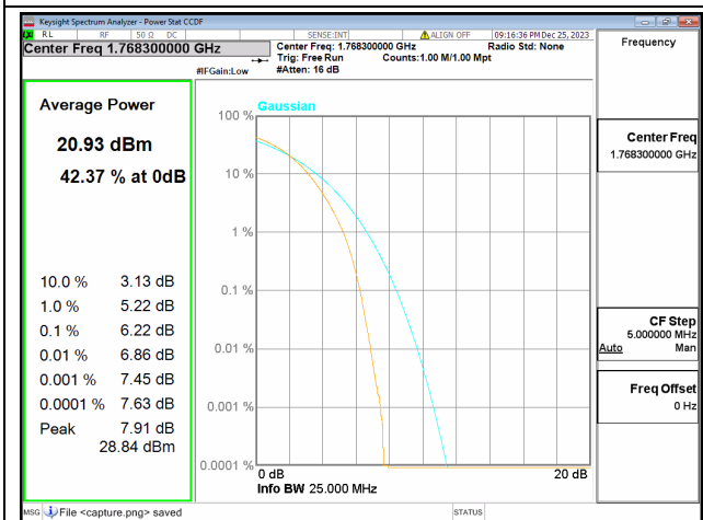
66C / 5+20MHz / High CH / QPSK
