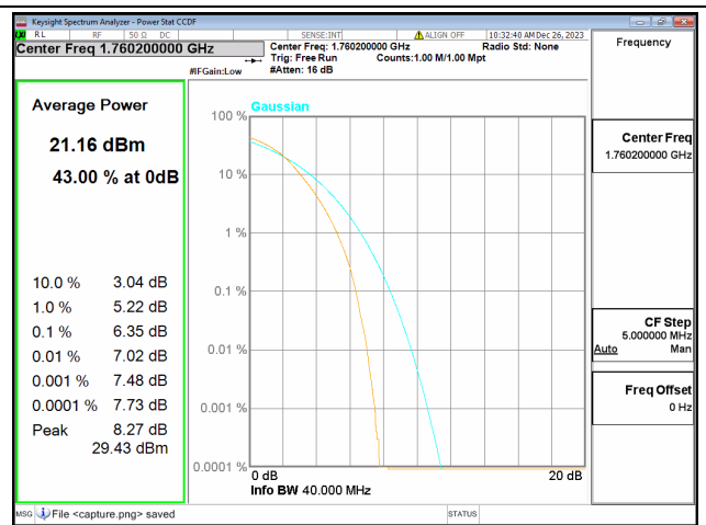
66C / 20+20MHz / High CH / QPSK
