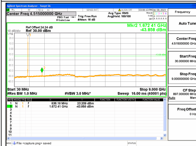
5B / 10+10MHz / QPSK / Mid CH / 1@49-1@0
