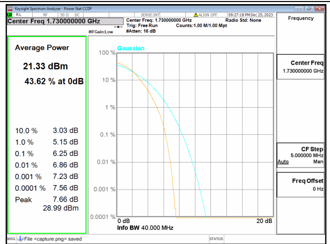
66C / 20+20MHz / Low CH / QPSK
