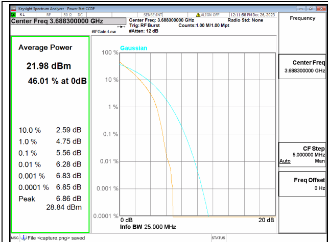
48C / 5+20MHz / High CH / QPSK
