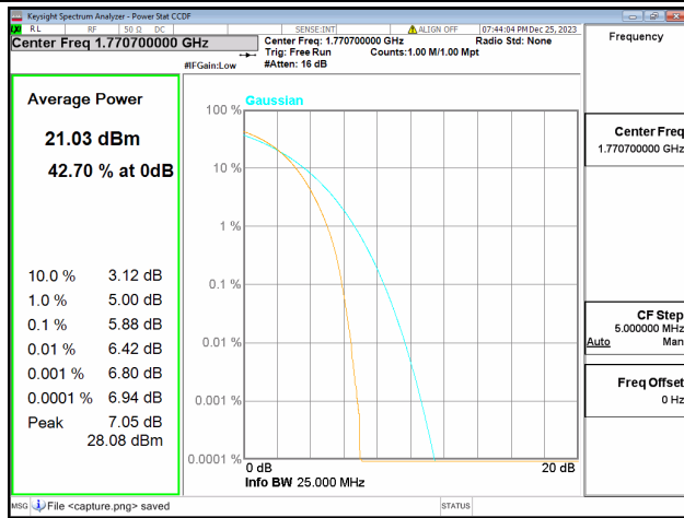
66B / 5+15MHz / High CH / QPSK
