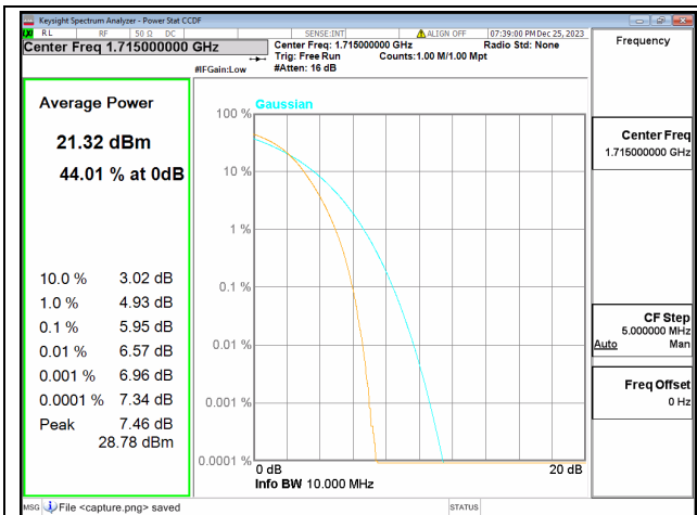
66B / 5+5MHz / Low CH / QPSK
