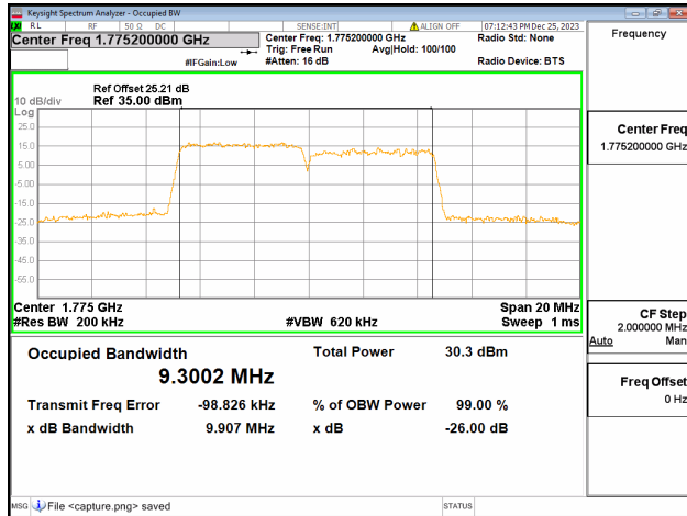
66B / 5+5MHz / QPSK/ High CH
