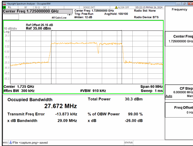
66C / 20+10MHz / QPSK/ Low CH
