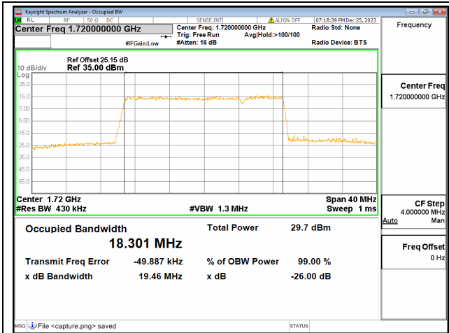
66B / 15+5MHz / 16QAM/ Low CH
