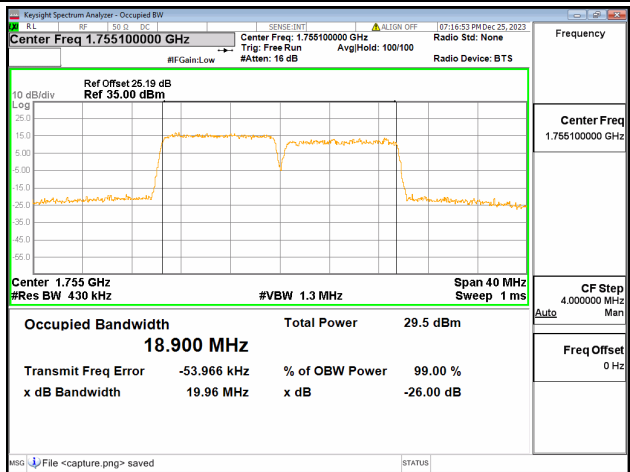
66B / 10+10MHz / 64QAM/ Mid CH
