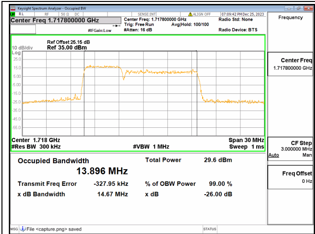
66B / 5+10MHz / 16QAM/ Low CH
