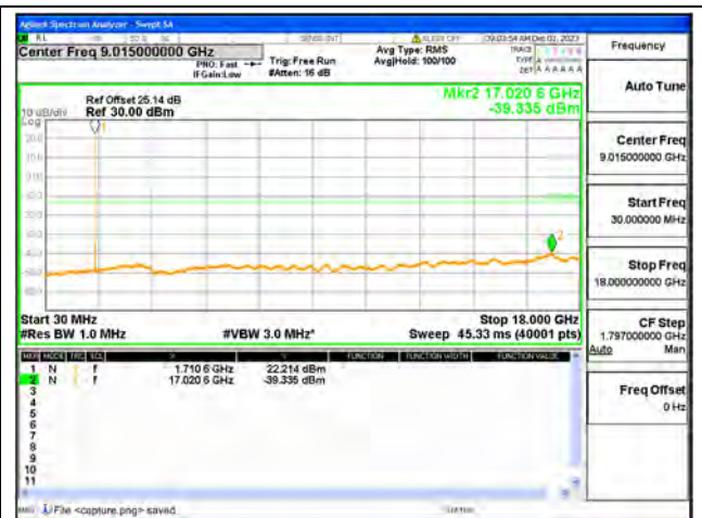
B4 / 5MHz / Low CH / QPSK
