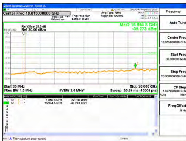
B2 / 10MHz / Low CH / QPSK
