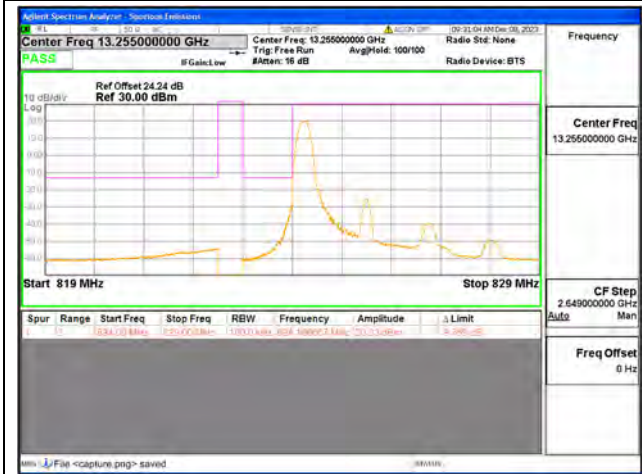
B5 / 3MHz / Low CH / QPSK / 1 RB
