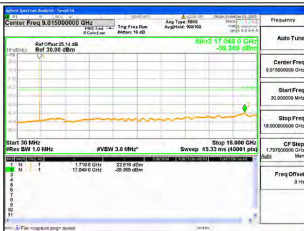
B4 / 10MHz / Low CH / QPSK
