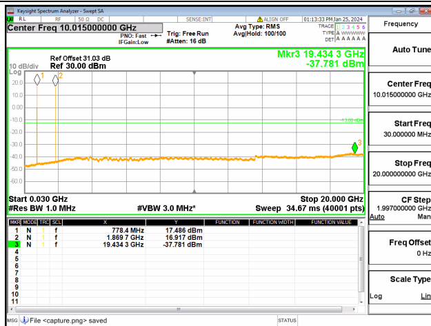
2A-13A / 20+10MHz / QPSK / Low+Mid CH / 1@99-1@0
