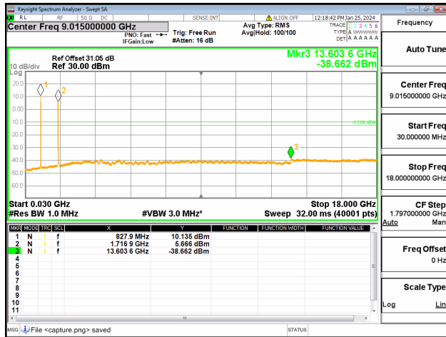
4A-5A / 20+10MHz / QPSK / Low+Low CH / 100@0-50@0
