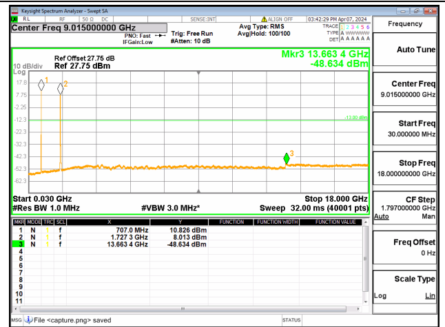
4A-12A / 20+10MHz / QPSK / Low+Mid CH / 100@0-50@0
