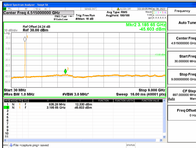
5B / 10+10MHz / QPSK / High CH / 50@0-50@
