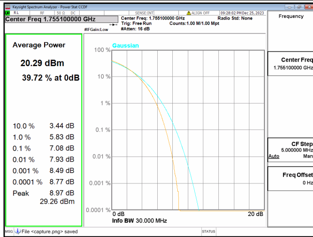
66C / 20+10MHz / Mid CH / 64QAM
