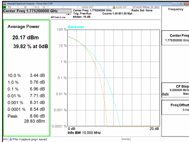
66B / 5+5MHz / High CH / 64QAM
