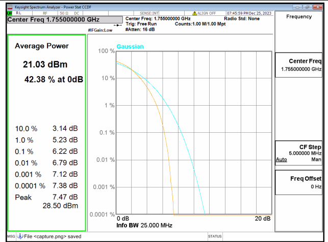
66B / 10+5MHz / Mid CH / QPSK
