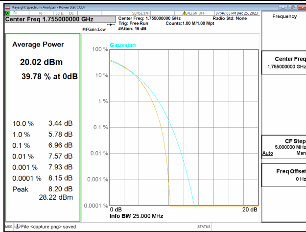
66B / 10+5MHz / Mid CH / 16QAM
