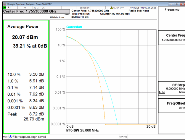
66B / 5+10MHz / Mid CH / 64QAM
