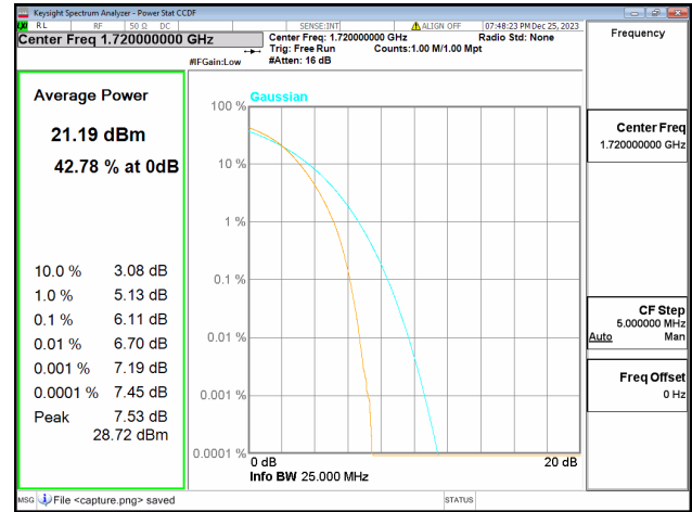
66B / 15+5MHz / Low CH / QPSK
