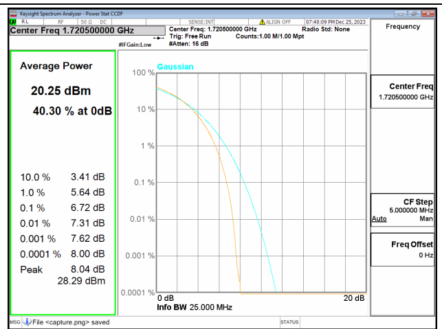
66B / 5+15MHz / Low CH / 16QAM
