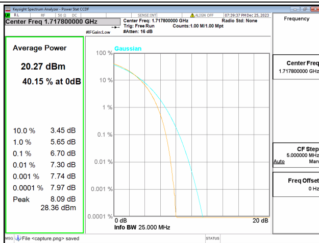
66B / 5+10MHz / Low CH / 16QAM
