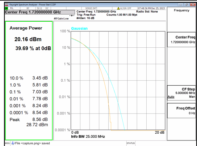
66B / 15+5MHz / Low CH / 64QAM
