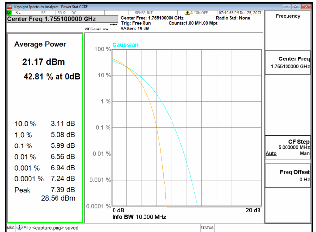
66B / 5+5MHz / Mid CH / QPSK
