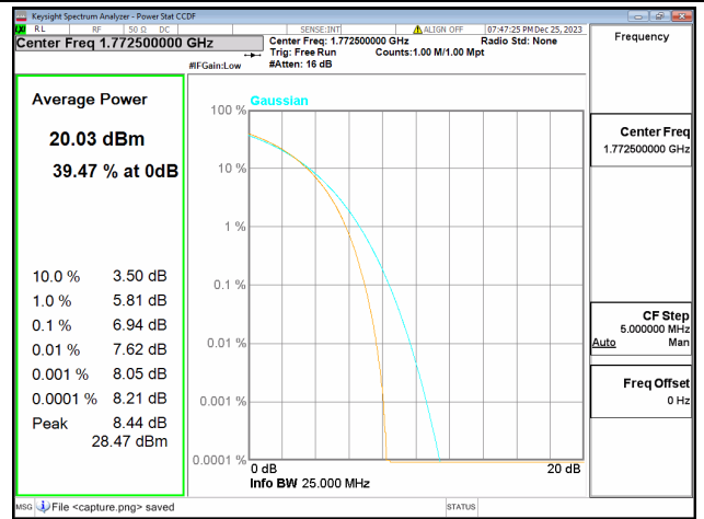
66B / 10+5MHz / High CH / 64QAM
