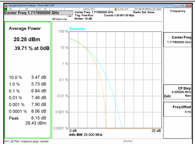
66B / 5+10MHz / Low CH / 64QAM
