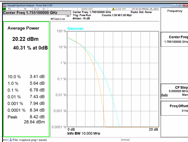
66B / 5+5MHz / Mid CH / 16QAM
