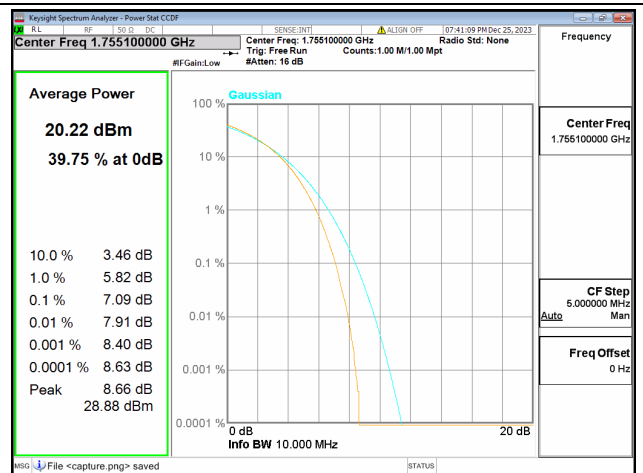
66B / 5+5MHz / Mid CH / 64QAM
