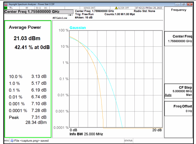
66B / 5+15MHz / Mid CH / QPSK
