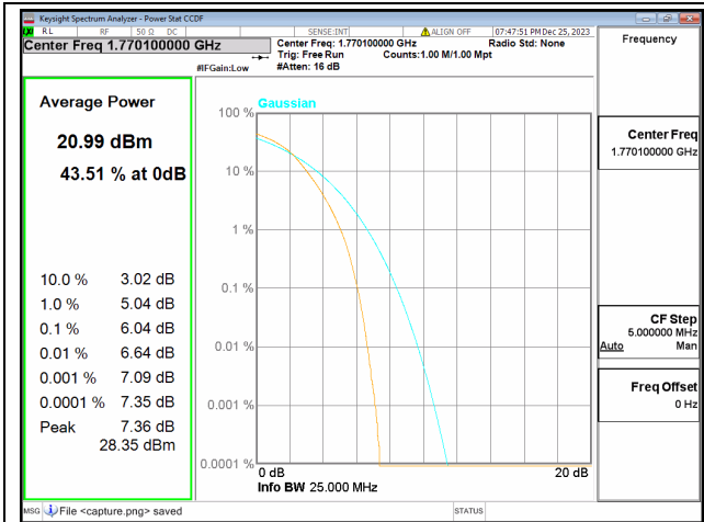
66B / 10+10MHz / High CH / QPSK
