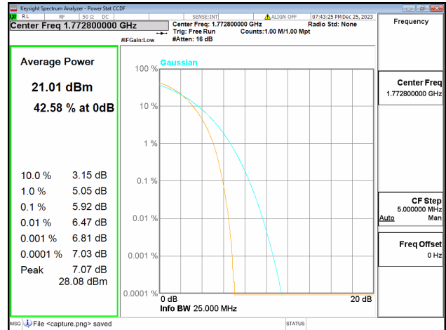
66B / 5+10MHz / High CH / QPSK
