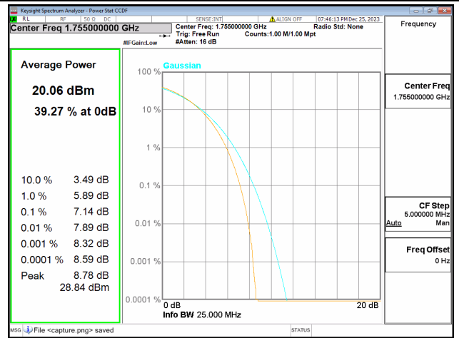
66B / 10+5MHz / Mid CH / 64QAM
