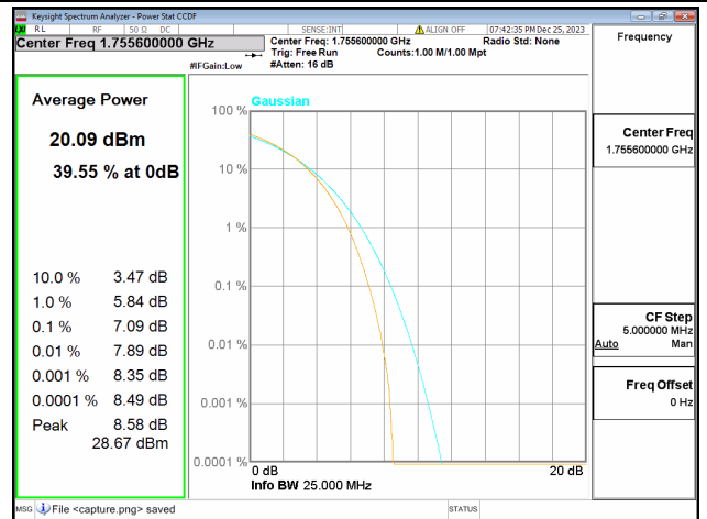
66B / 5+15MHz / Mid CH / 64QAM
