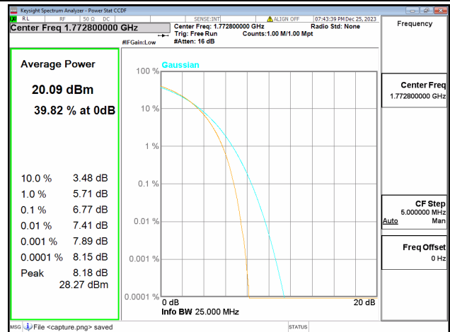
66B / 5+10MHz / High CH / 64QAM
