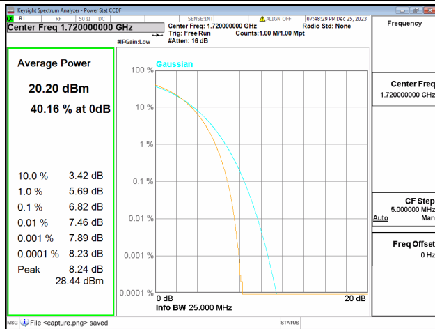
66B / 15+5MHz / Low CH / 16QAM
