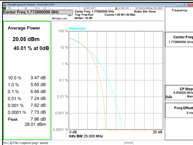
66B / 5+10MHz / High CH / 16QAM
