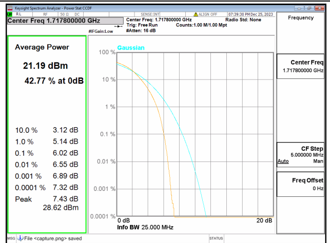
66B / 5+10MHz / Low CH / QPSK
