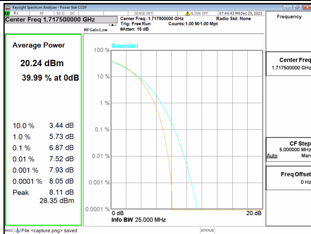
66B / 10+5MHz / Low CH / 16QAM
