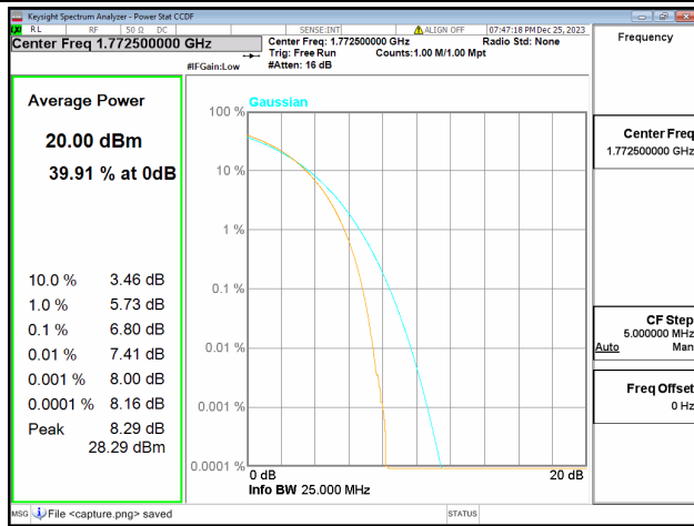
66B / 10+5MHz / High CH / 16QAM
