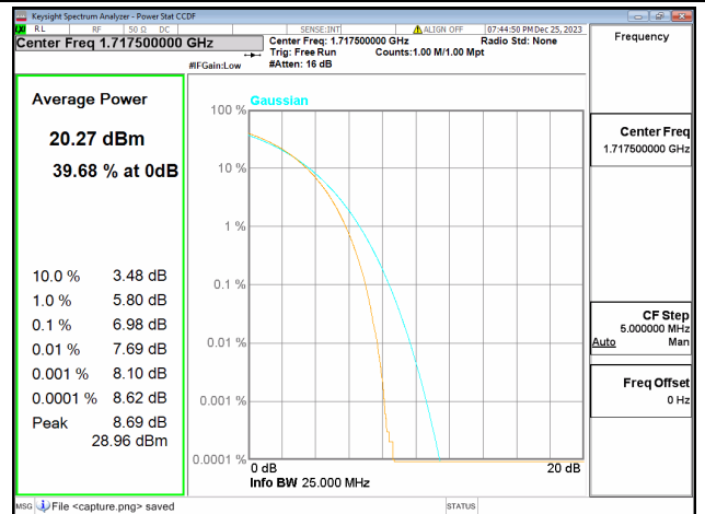
66B / 10+5MHz / Low CH / 64QAM
