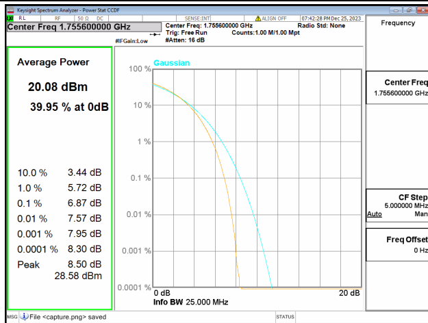
66B / 5+15MHz / Mid CH / 16QAM
