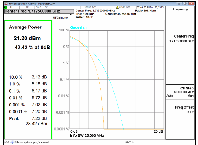
66B / 10+5MHz / Low CH / QPSK
