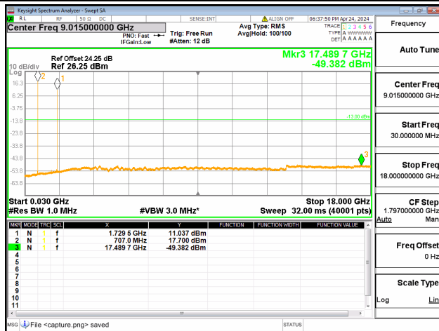
12A-66A / 10+20MHz / QPSK / High+Low CH / 1@0-1@99
