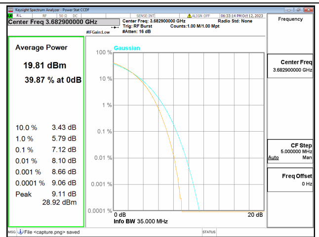
48C / 15+20MHz / High CH / 16QAM
