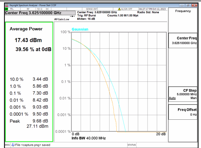
48C / 20+20MHz / Mid CH / 256QAM
