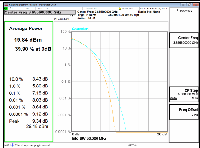
48C / 10+20MHz / High CH / 16QAM
