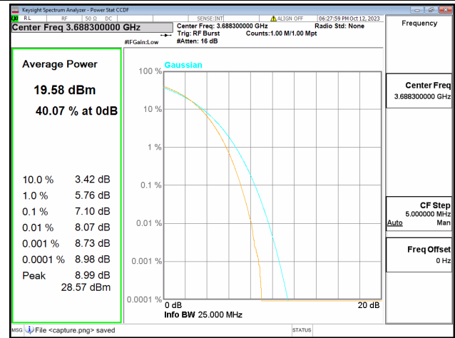
48C / 5+20MHz / High CH / 16QAM
