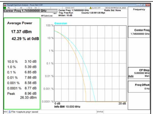
B66 / 10MHz / Mid CH / 256QAM
