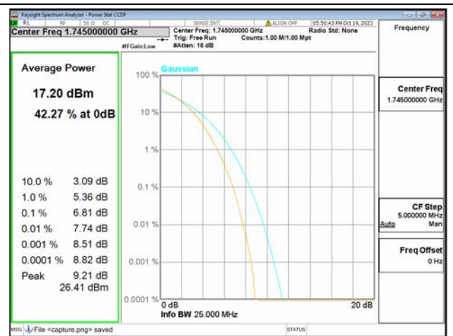
B66 / 20MHz / Mid CH / 256QAM
