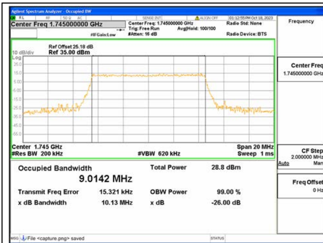
B66 / 10MHz / 64QAM/ Mid CH
