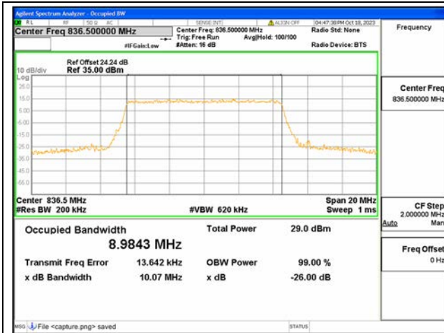
B5 / 10MHz / 64QAM/ Mid CH
