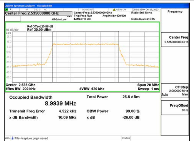
B7 / 10MHz / 256QAM/ Mid CH
