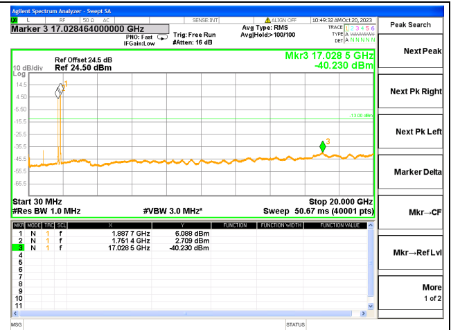
2A-66A/20M+20M /QPSK/Mid CH
