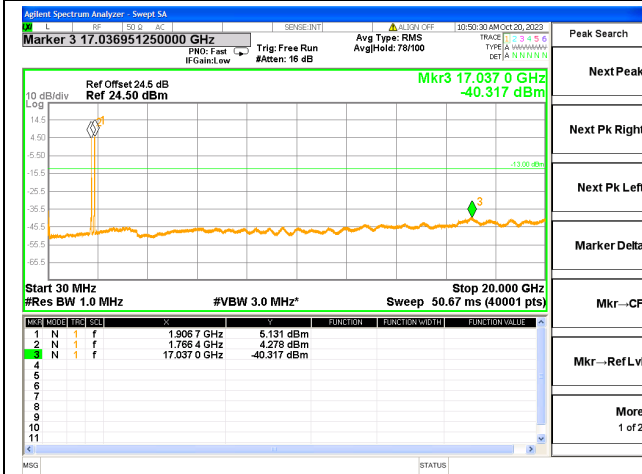
2A-66A/20M+20M/QPSK/ High CH
