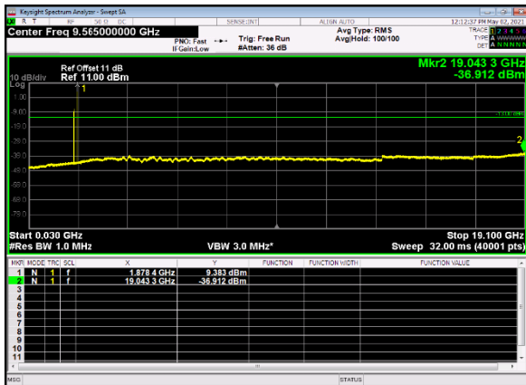
B66_n2(5M)_DFT-s-OFDM_BPSK_Edge_ 1RB_Left_Mid_CH
