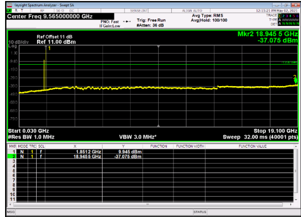
B66_n2(10M)_DFT-s-OFDM_QPSK_Edge_1RB_Left_Low_CH
