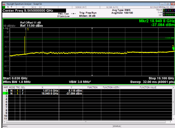
B66_n2(15M)_DFT-s-OFDM_BPSK_Edge_ 1RB_Left_Mid_CH
