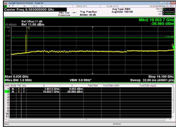
B66_n2(20M)_DFT-s-OFDM_QPSK_Edge_ 1RB_Left_Low_CH
