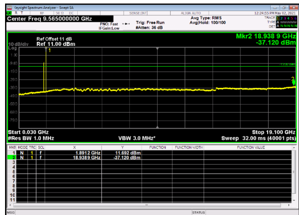
B66_n2(20M)_DFT-s-OFDM_QPSK_Edge_ 1RB_Left_High_CH
