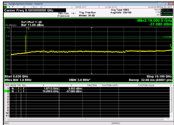
B66_n2(20M)_DFT-s-OFDM_QPSK_Edge_ 1RB_Left_Mid_CH
