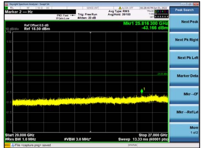
B41-20G-27G / 10MHz+15MHz /1RB+1RB/ QPSK / LOW CH
