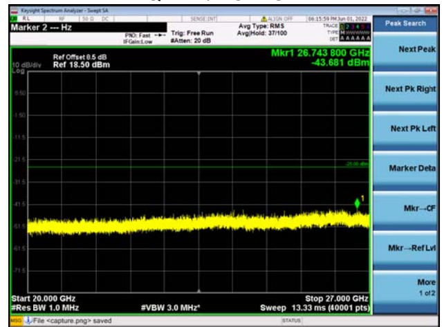
B41-20G-27G / 20MHz+5MHz /1RB+1RB/ QPSK / LOW CH
