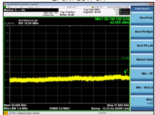
B41-20G-27G / 5MHz+20MHz /25RB+100RB/ QPSK / LOW CH
