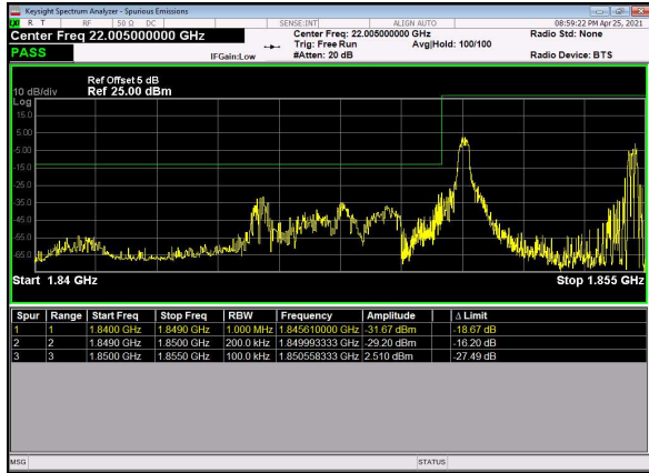
N2(20M)_DFT-s-OFDM_BPSK_Edge_1RB_Lef t_Low_CH
