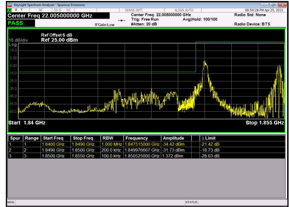
N2(20M)_DFT-s-OFDM_QPSK_Edge_1RB_Lef t_Low_CH
