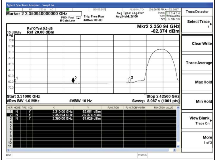
802.11b-Low channel(Average)
