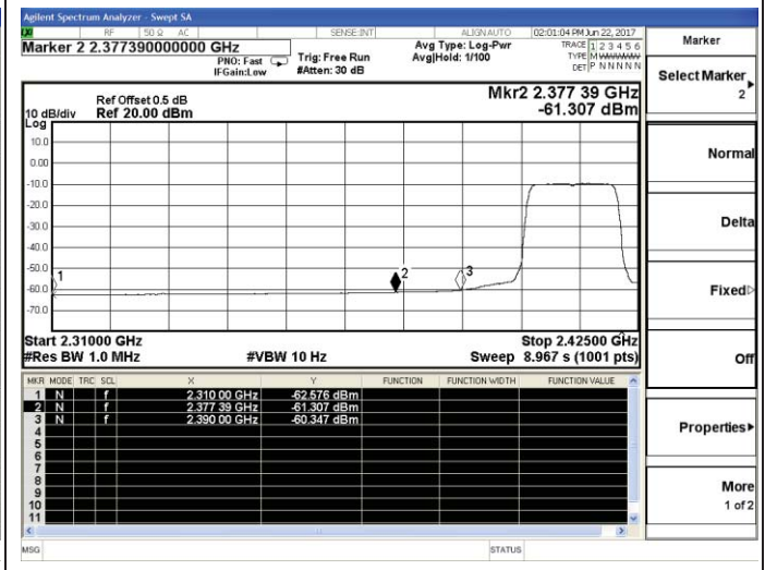
802.11g-Low channel(Average)
