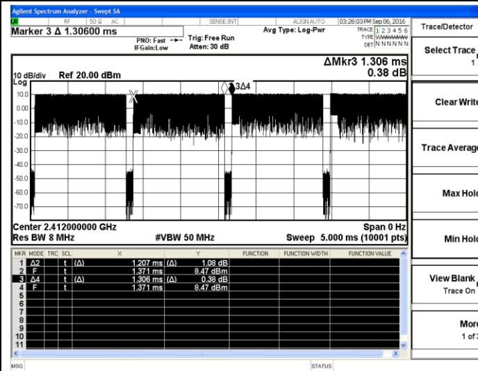
802.11b
