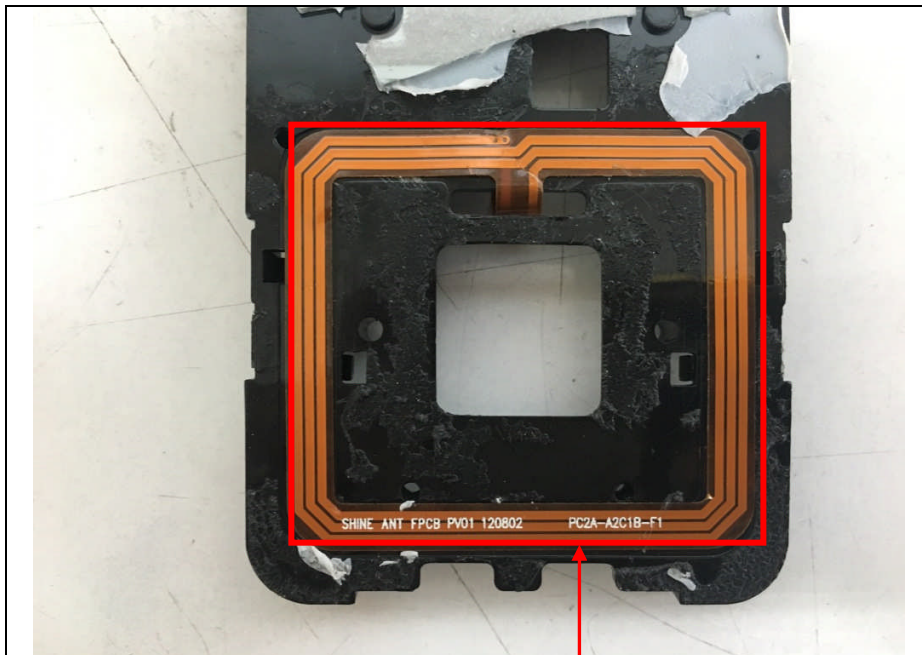
NFC Antenna
