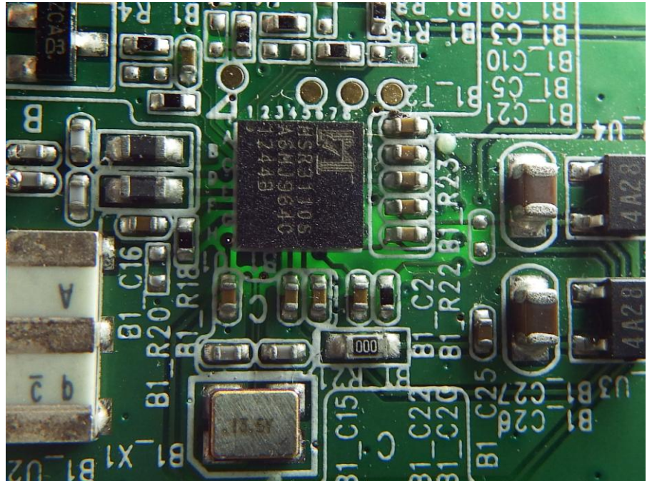
NFC Chip
