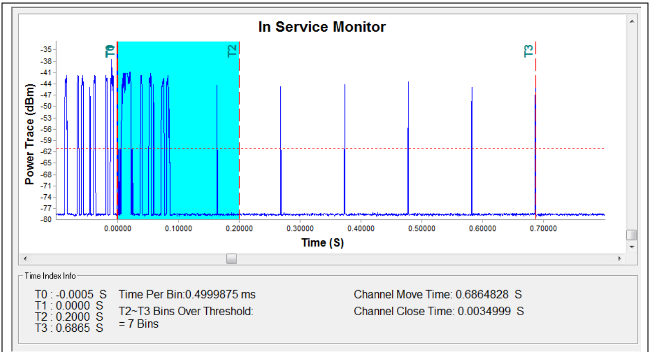
(5520MHz, 802.11a)
