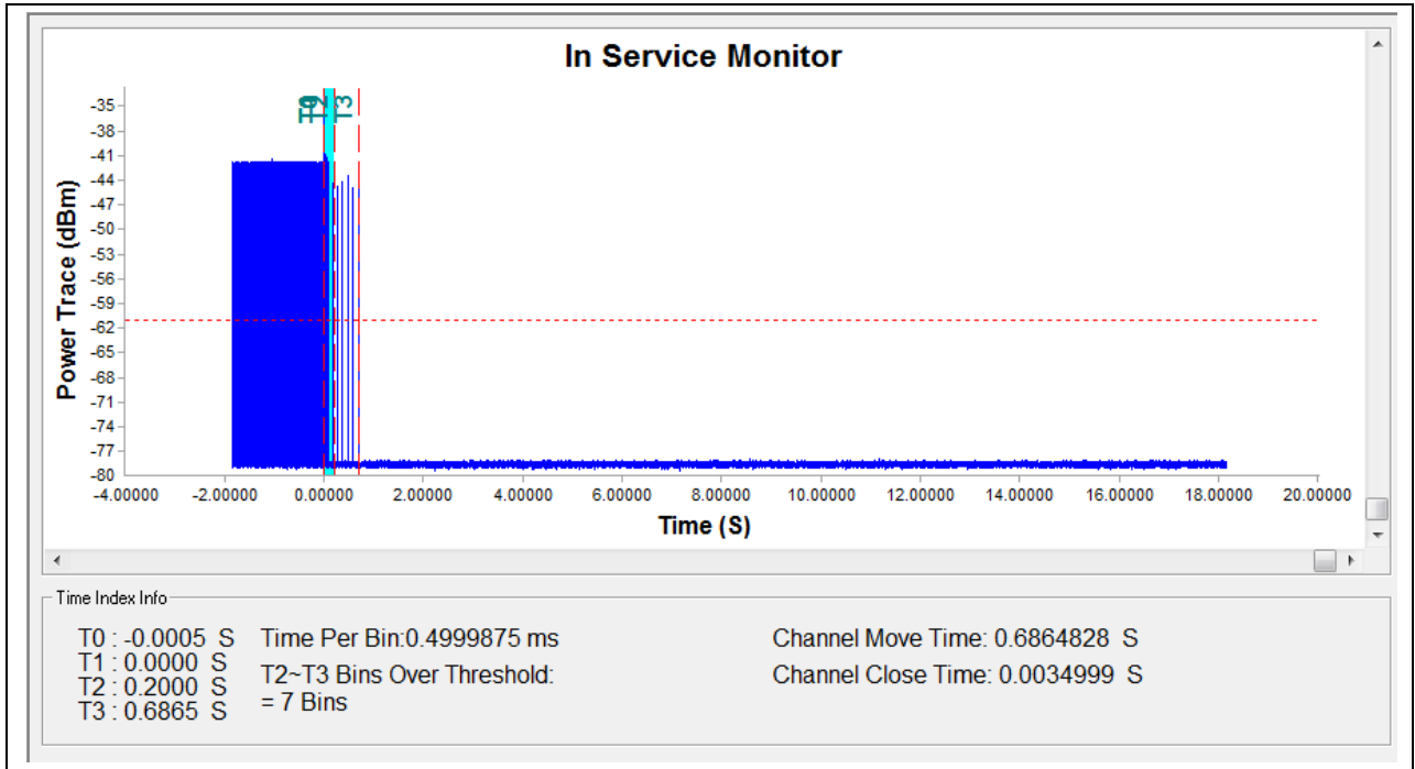
(5520MHz, 802.11a)
