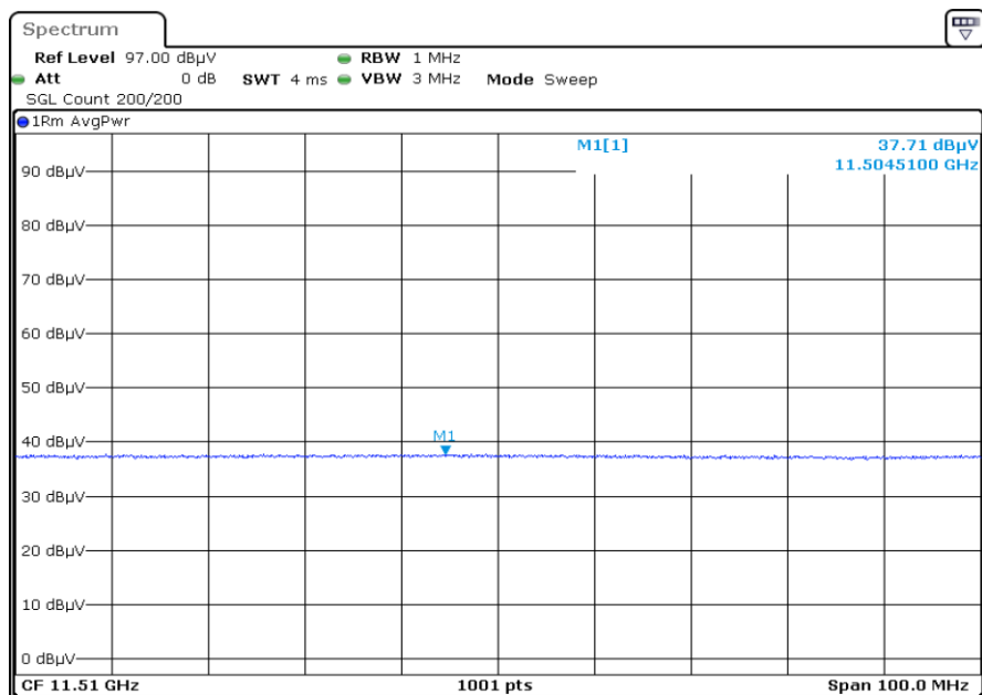
F1 X2 11510.0 Harmonic Vertical AVG
