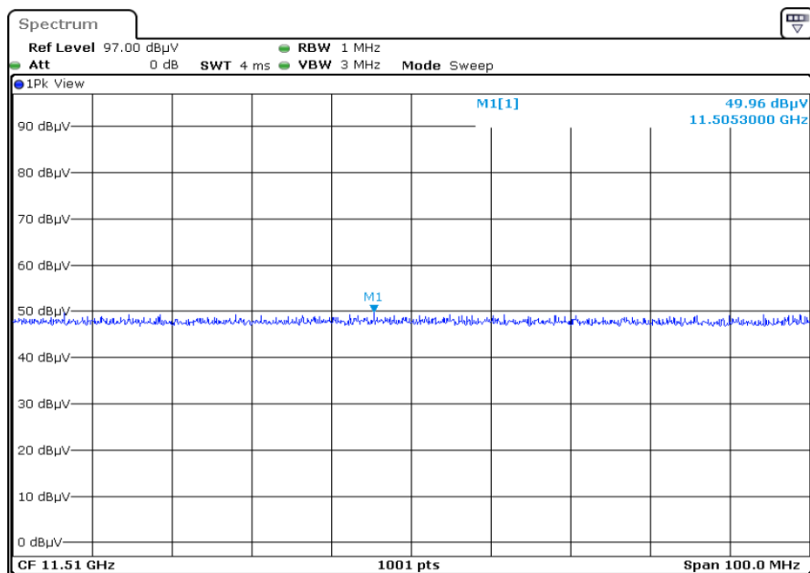
F1 X2 11510.0 Harmonic Vertical PEAK
