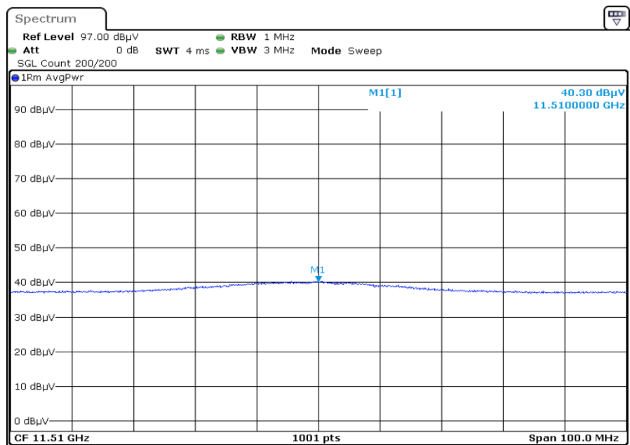
F1 X2 11510.0 Harmonic Horizontal AVG
