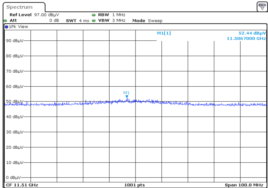
F1 X2 11510.0 Harmonic Horizontal PEAK
