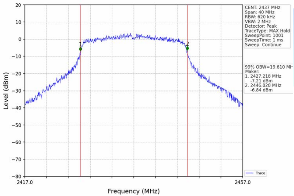
802.11ax(HEW20)_MCH_2437MHz_RU242_Left_Ant1 (SISO)_NTNV
