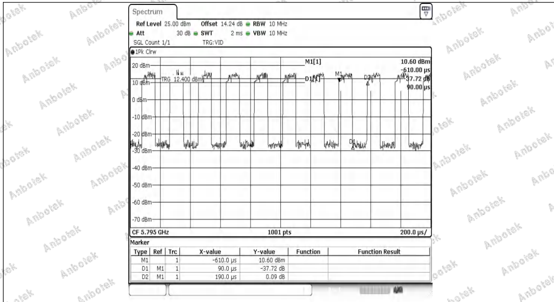
NTNV-11AX40MIMO-Ant1-5795
