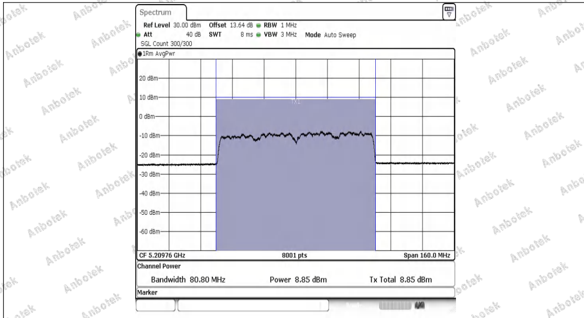
11AX80MIMO-Ant1-5210-PASS
