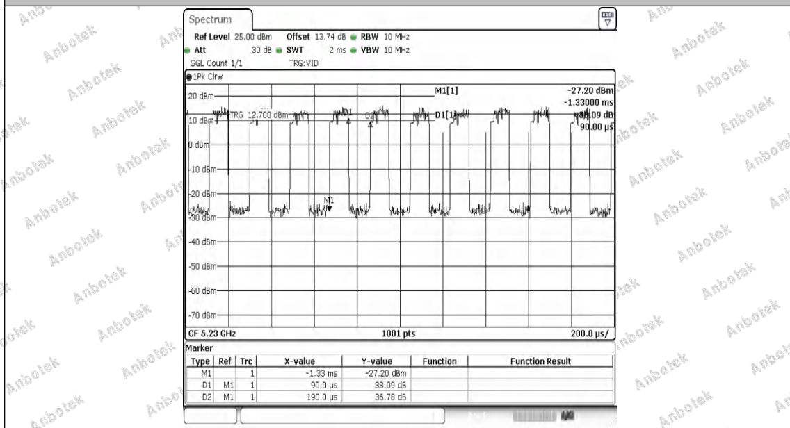
NTNV-11AX40MIMO-Ant2-5230
