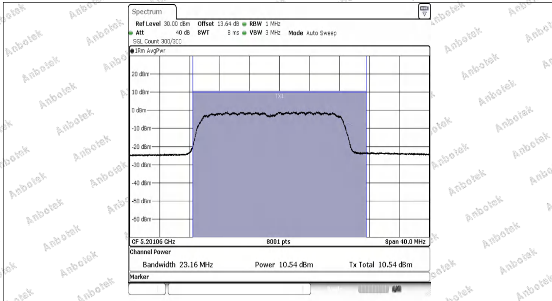
11AX20MIMO-Ant1-5200-PASS
