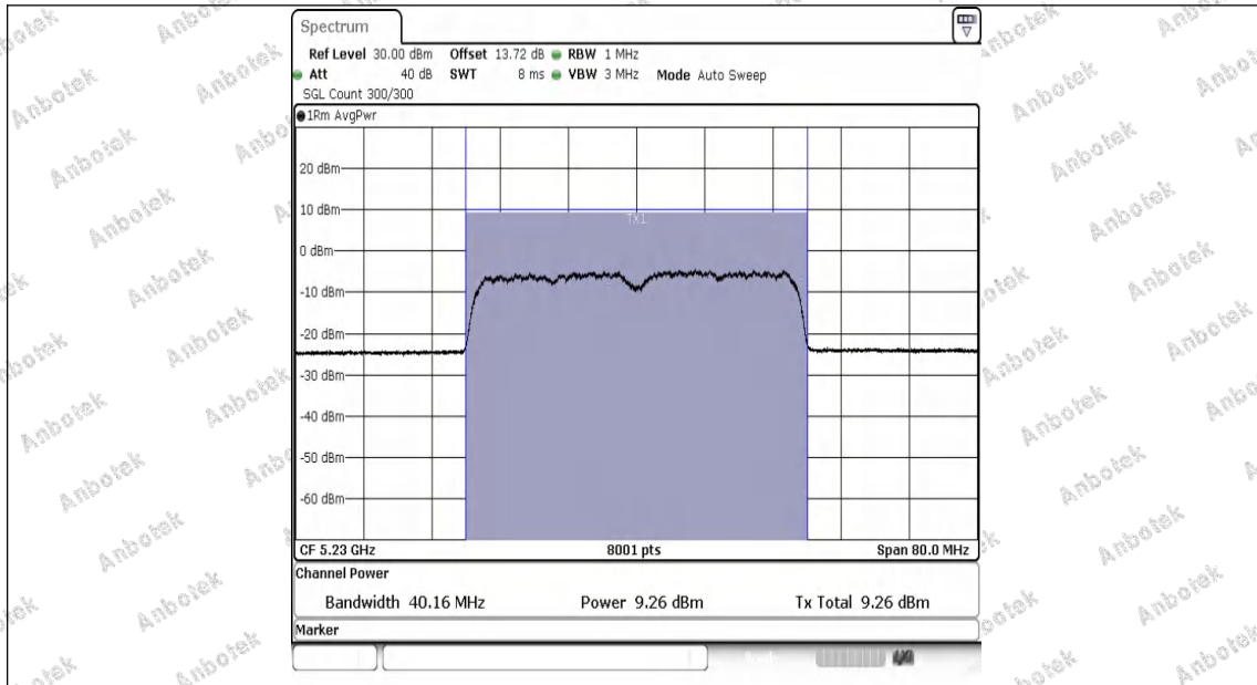
11AX40MIMO-Ant1-5230-PASS
