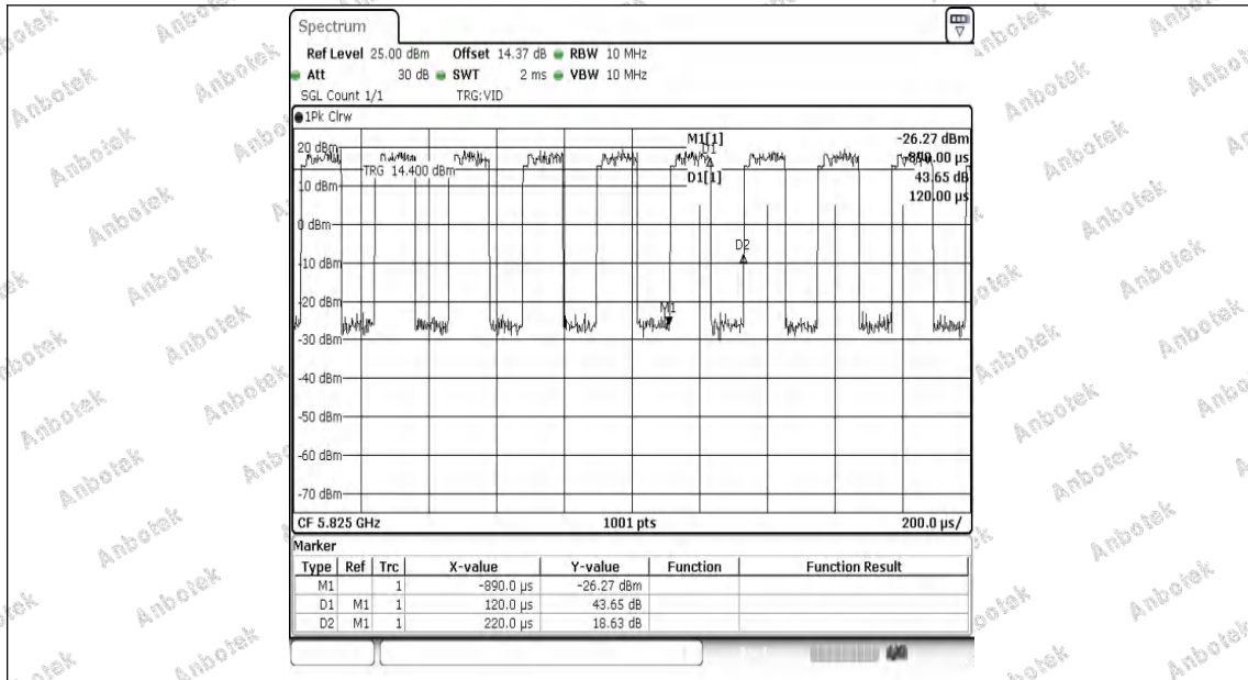
NTNV-11AX20MIMO-Ant1-5825
