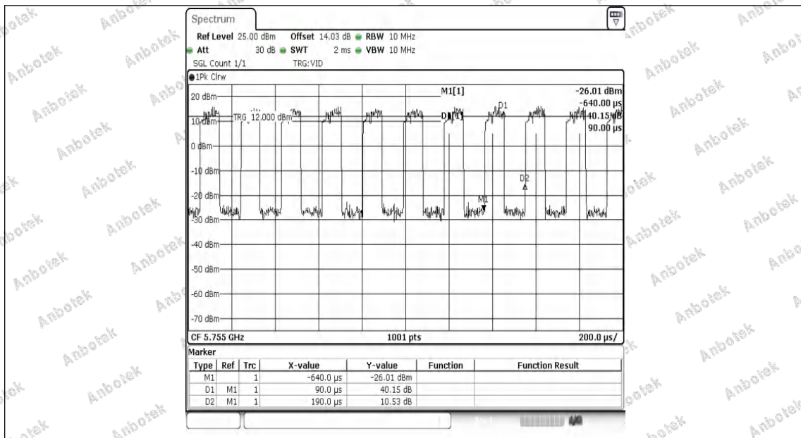
NTNV-11AX40MIMO-Ant1-5755
