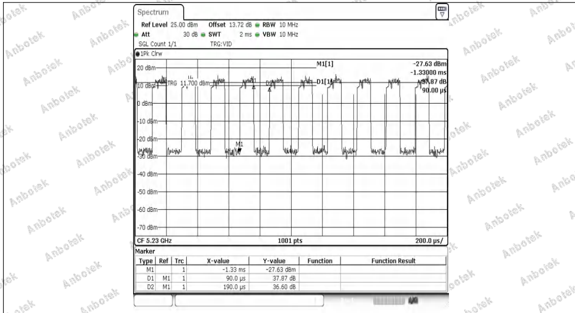
NTNV-11AX40MIMO-Ant1-5230
