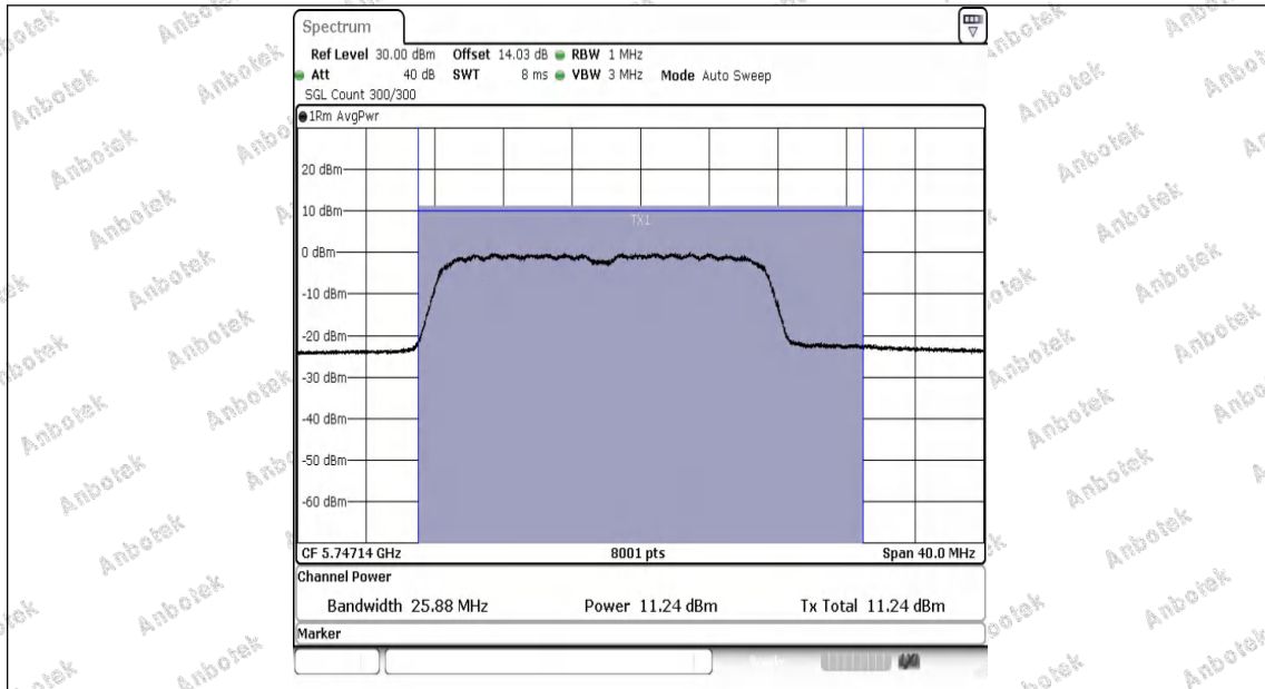
11AX20MIMO-Ant1-5745-PASS
