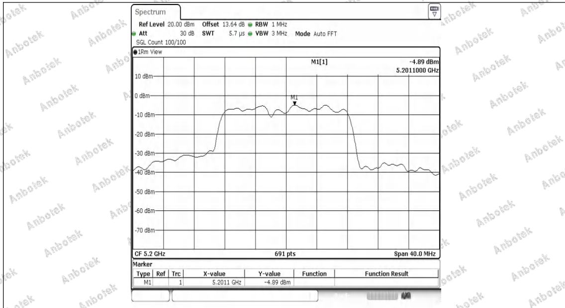
11N20MIMO-Ant1-5200-PASS
