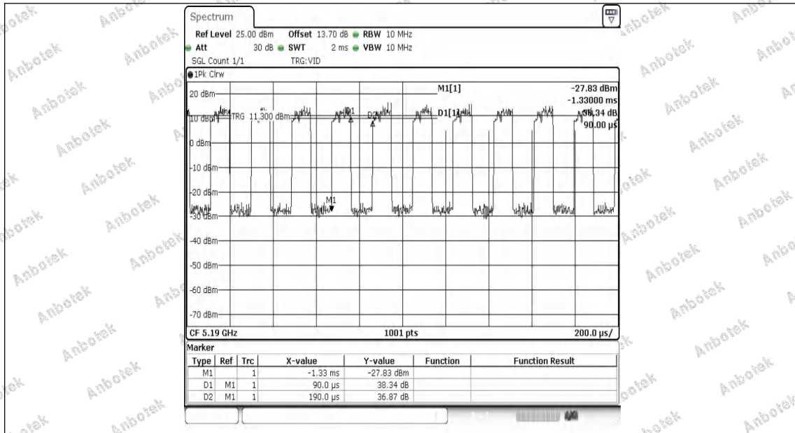
NTNV-11AX40MIMO-Ant1-5190
