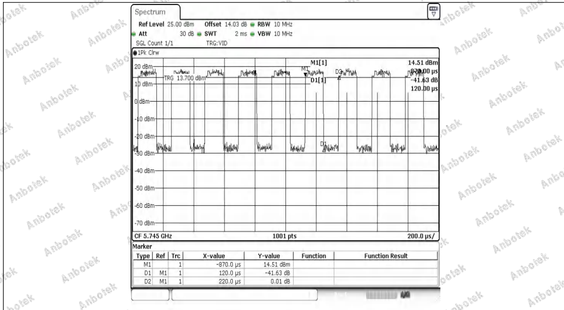
NTNV-11AX20MIMO-Ant1-5745
