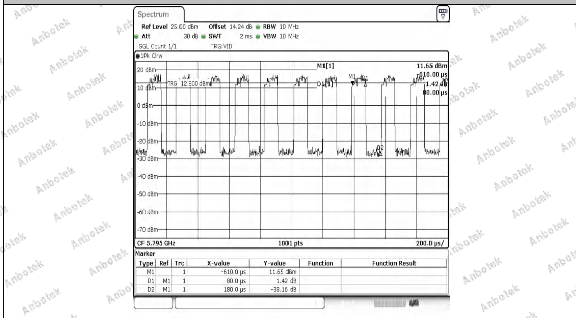
NTNV-11AX40MIMO-Ant2-5795
