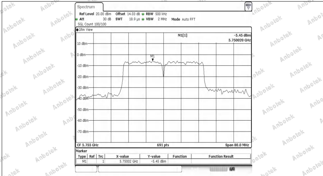
11N40MIMO-Ant1-5755-PASS
