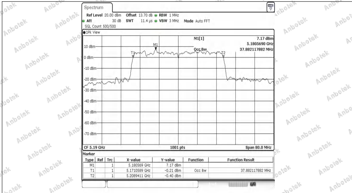
11AX40MIMO-Ant1-5190
