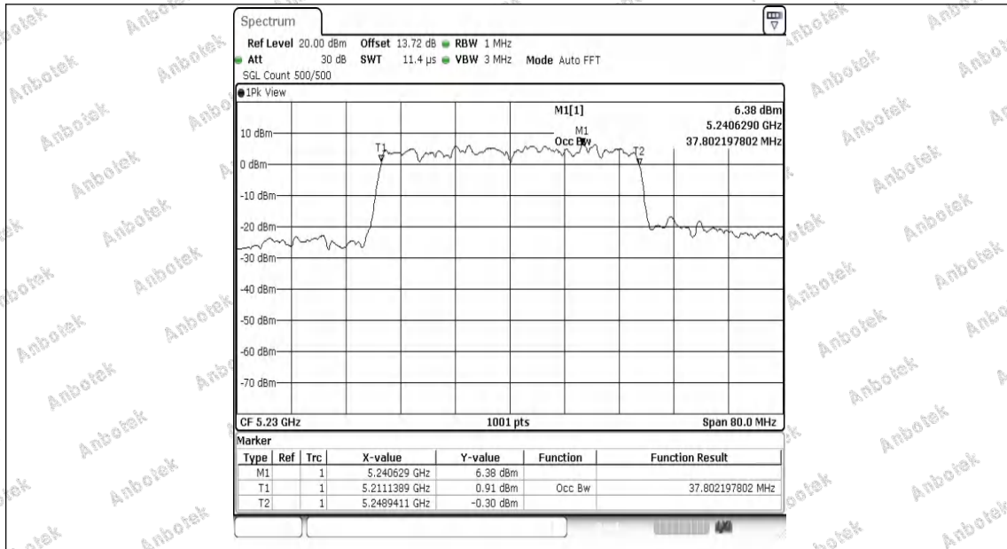
11AX40MIMO-Ant1-5230
