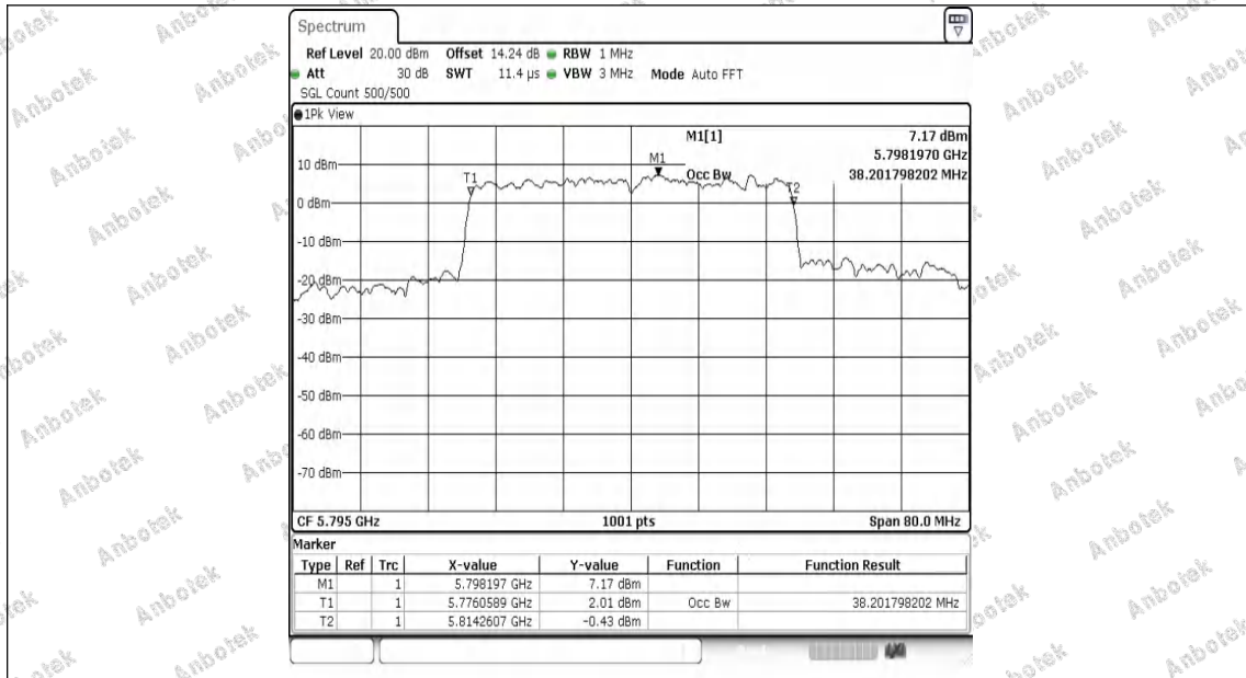
11AX40MIMO-Ant1-5795
