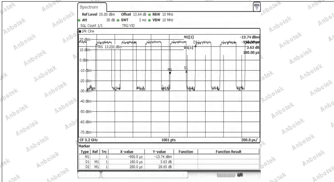
NTVN-11A-Ant1-5200
