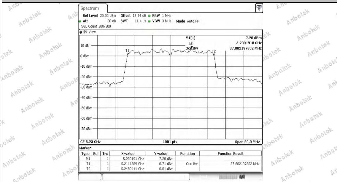
11AX40MIMO-Ant2-5230
