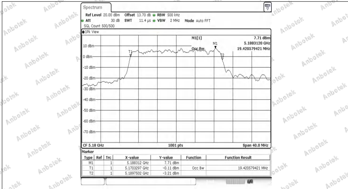
11AX20MIMO-Ant1-5180
