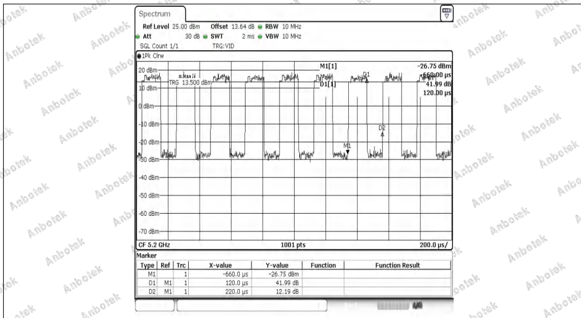
NTNV-11AX20MIMO-Ant1-5200
