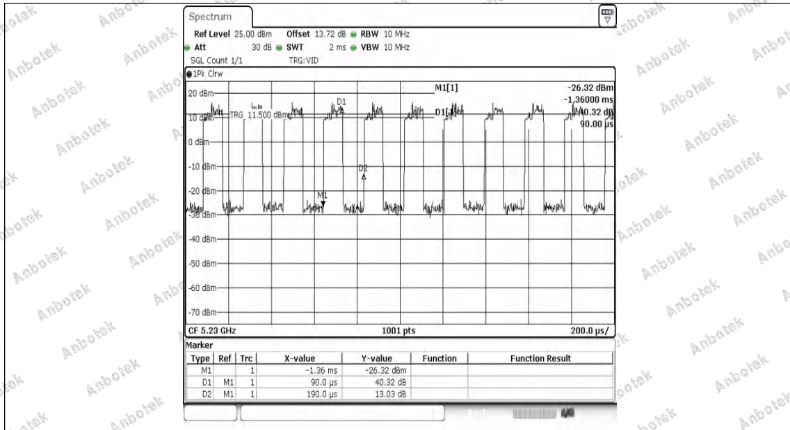
NTNV-11AC40MIMO-Ant1-5230
