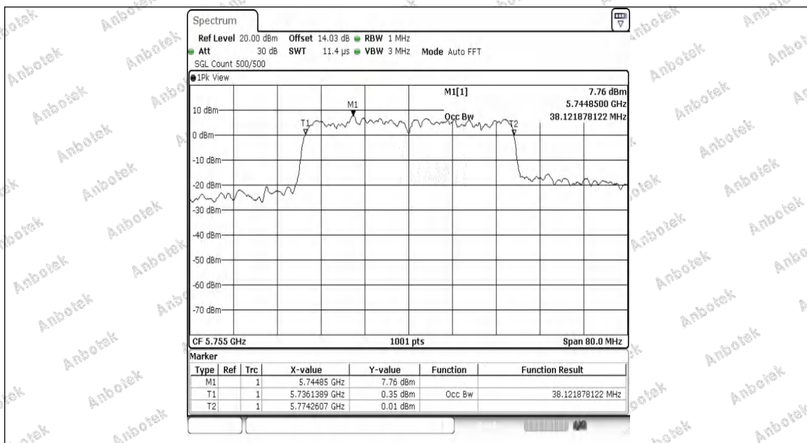
11AX40MIMO-Ant1-5755
