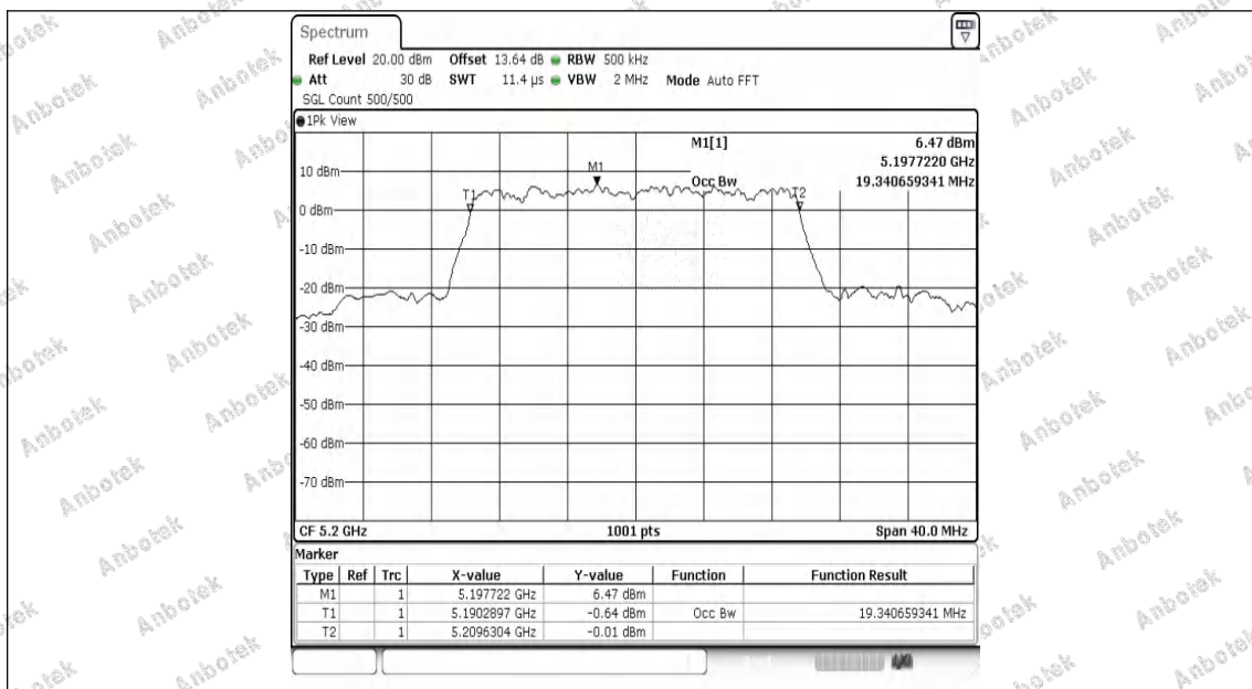
11AX20MIMO-Ant1-5200
