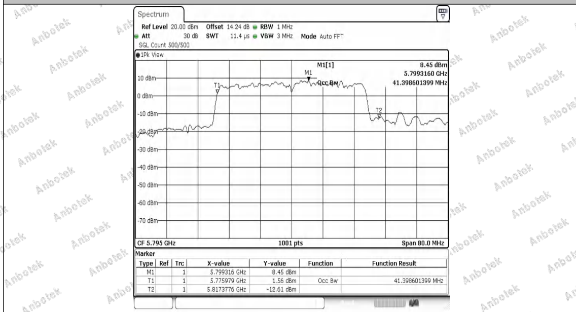
11AX40MIMO-Ant2-5795
