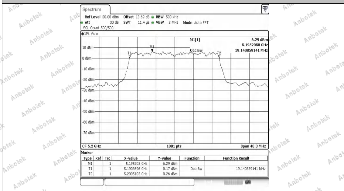
11AX20MIMO-Ant2-5200
