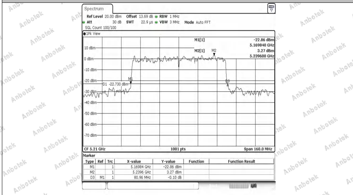
11AX80MIMO-Ant2-5210
