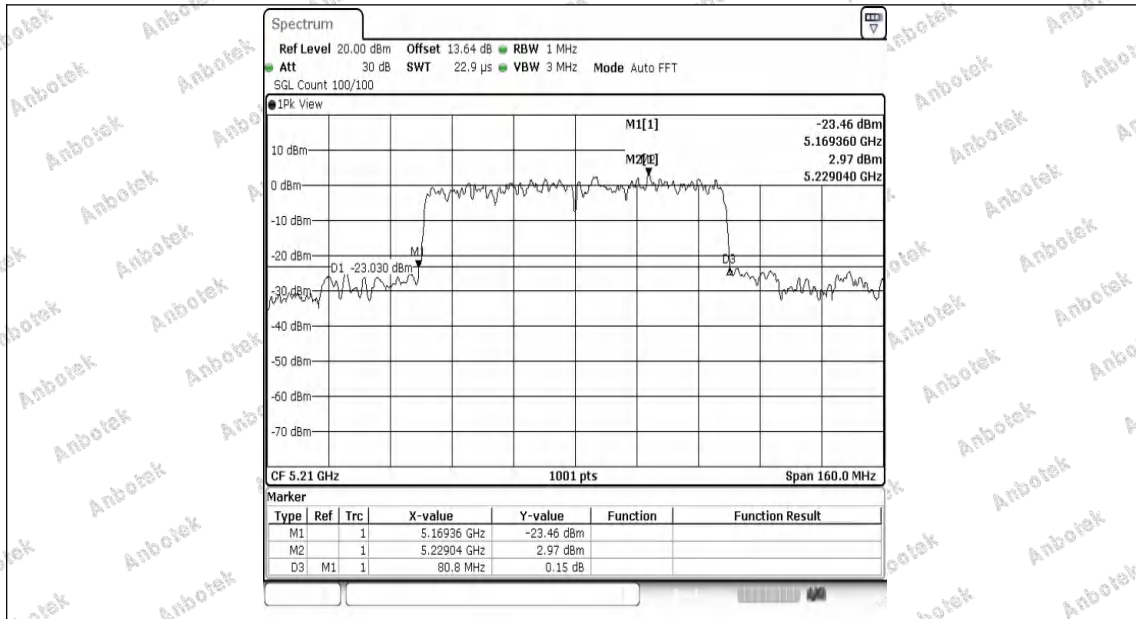
11AX80MIMO-Ant1-5210
