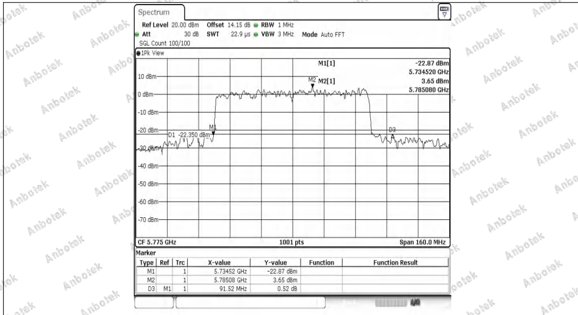
11AX80MIMO-Ant1-5775
