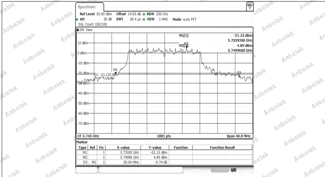
11A-Ant1-5745
