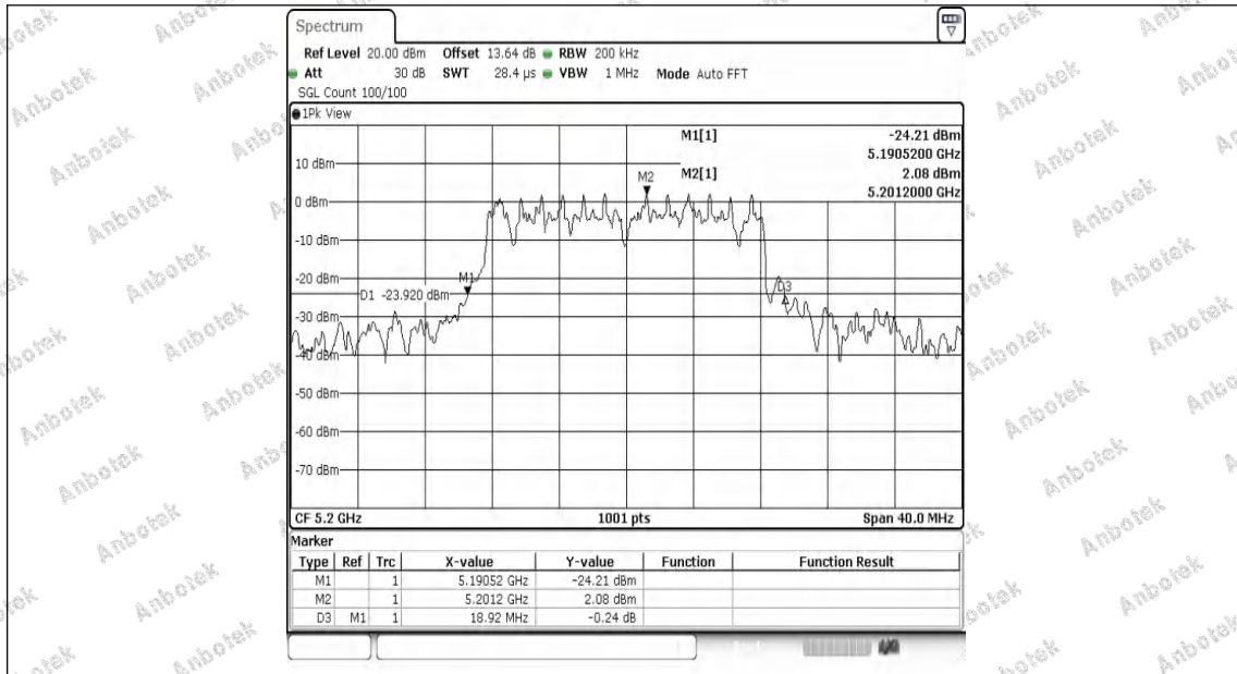
11AC20MIMO-Ant1-5200
