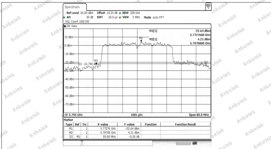
11AX40MIMO-Ant1-5795
