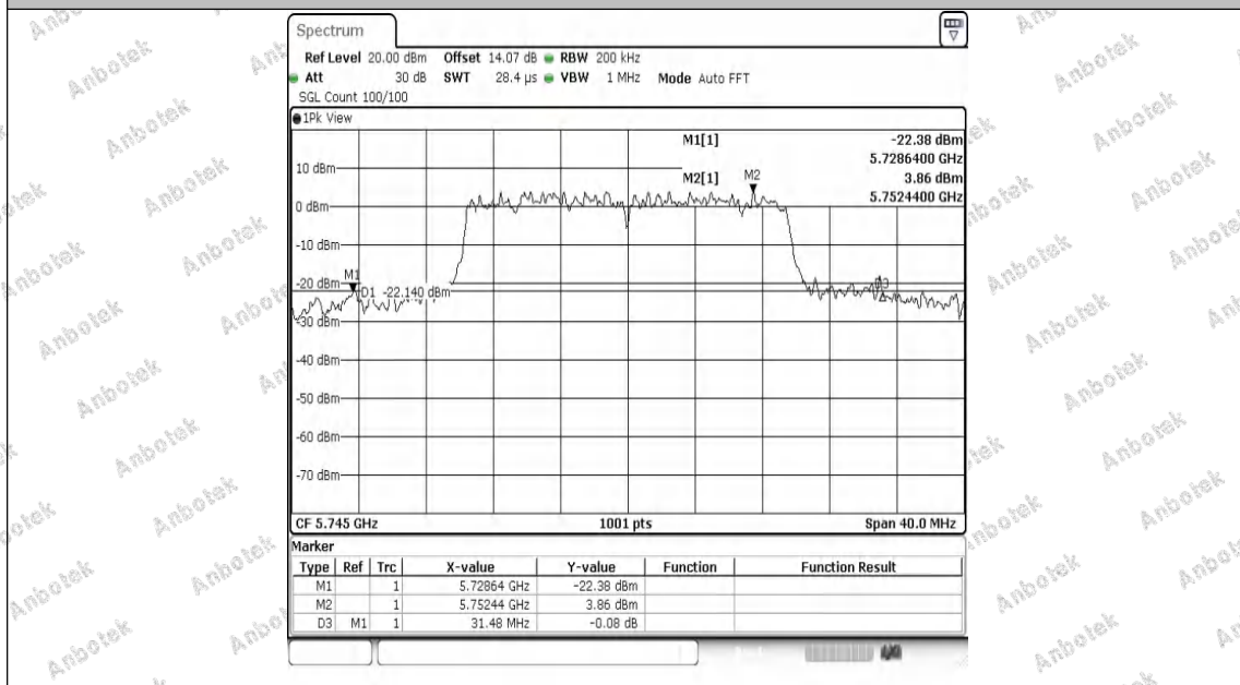
11AX20MIMO-Ant2-5745
