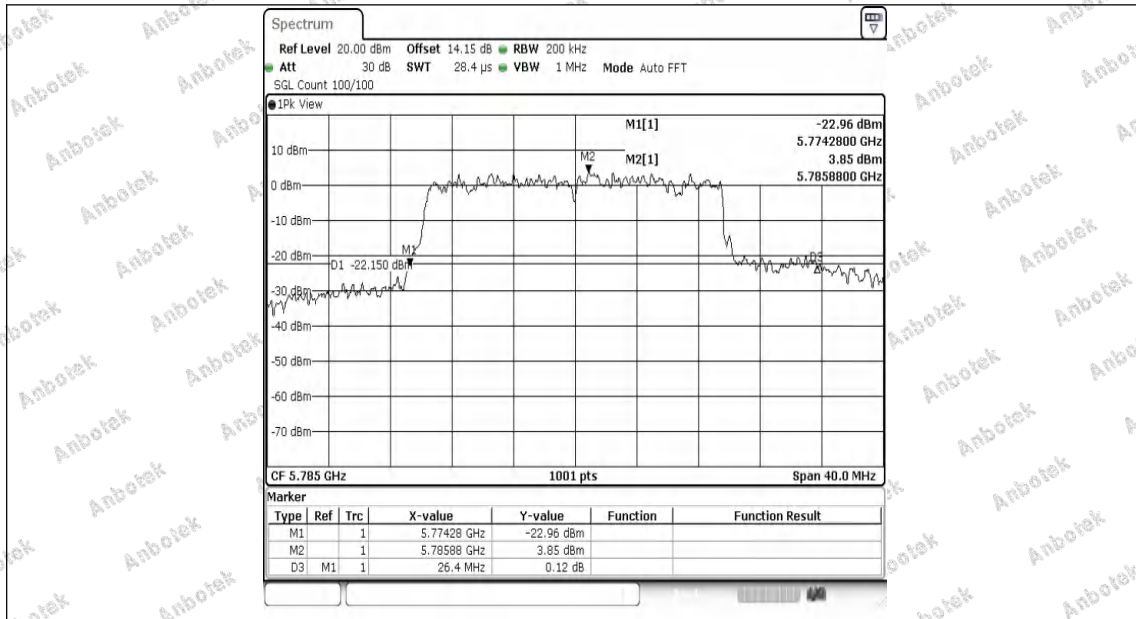
11AX20MIMO-Ant1-5785
