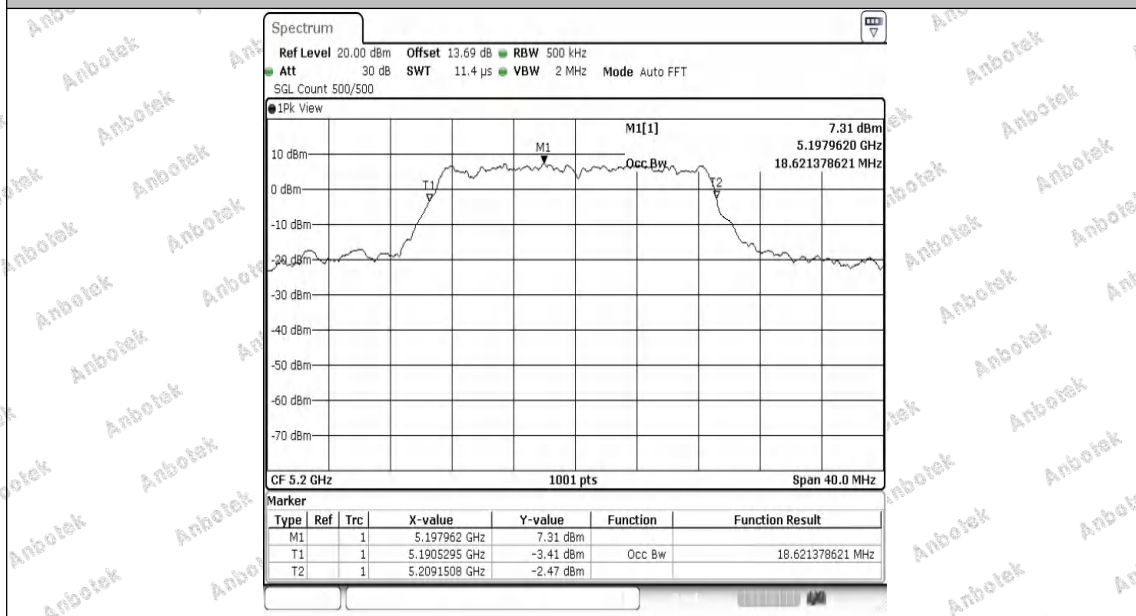
11N20MIMO-Ant2-5200
