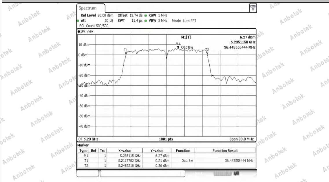
11N40MIMO-Ant2-5230
