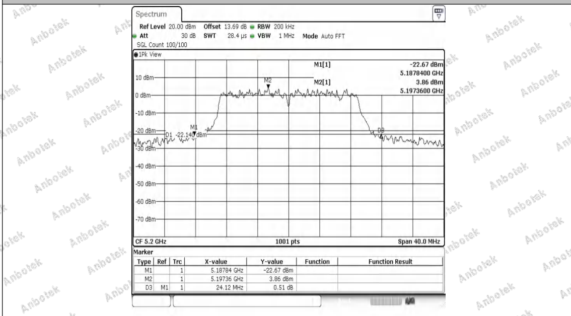
11N20MIMO-Ant2-5200
