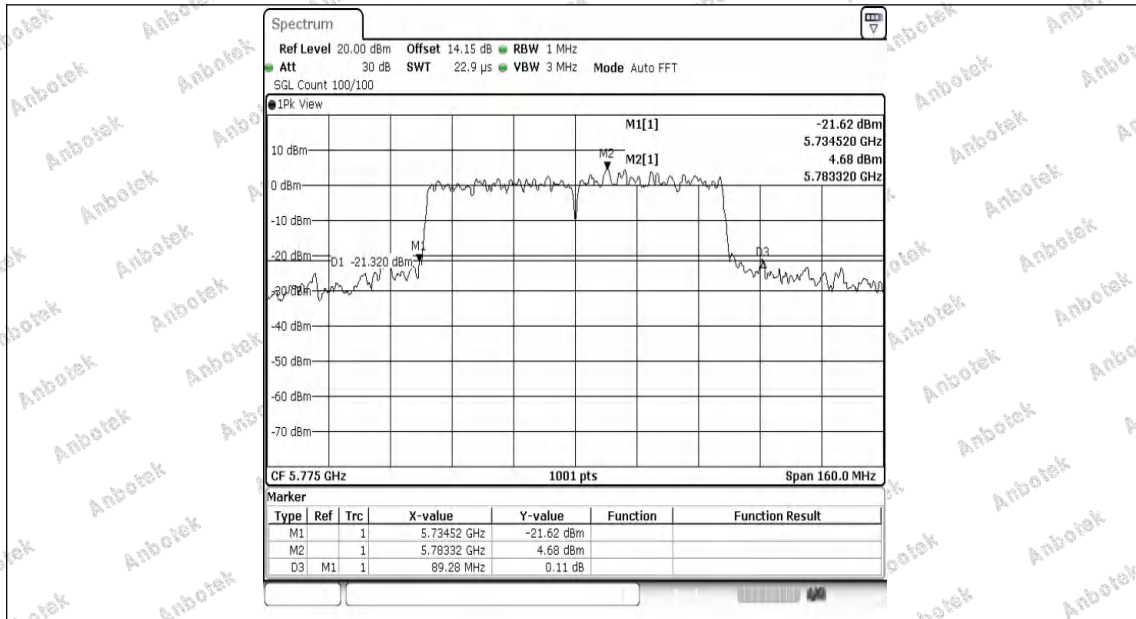
11AC80MIMO-Ant1-5775
