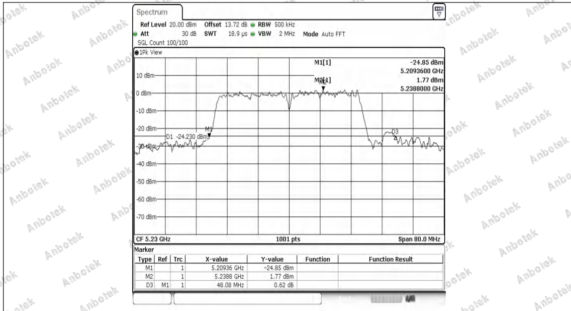
11AC40MIMO-Ant1-5230
