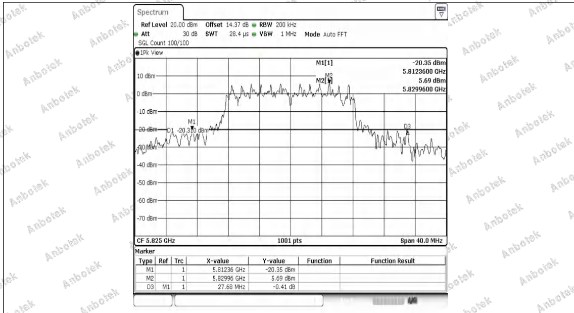
11N20MIMO-Ant1-5825
