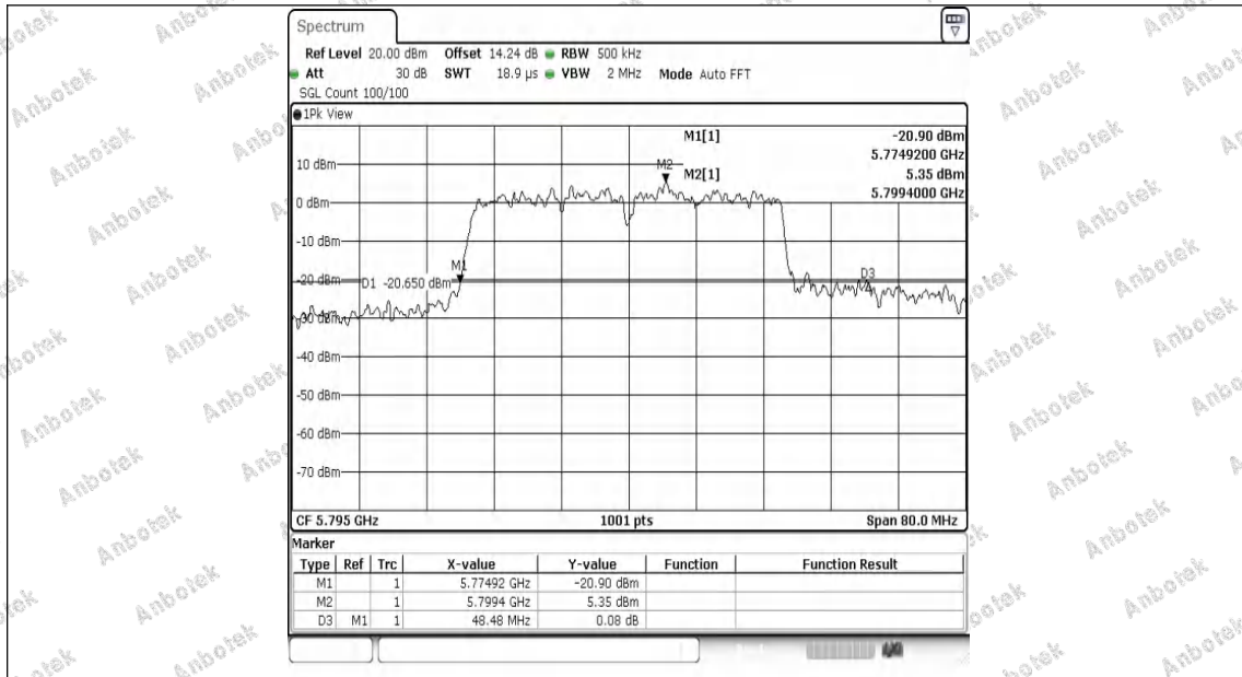
11AC40MIMO-Ant1-5795
