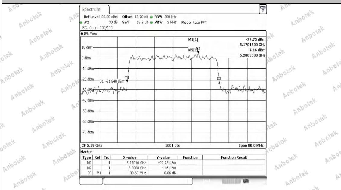
11AX40MIMO-Ant2-5190
