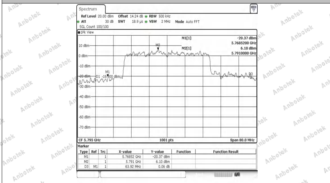
11AX40MIMO-Ant2-5795
