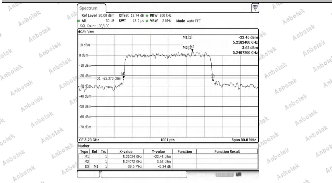
11AX40MIMO-Ant2-5230
