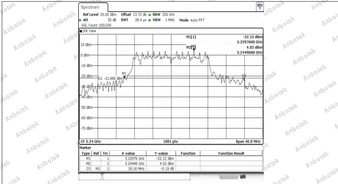
11N20MIMO-Ant1-5240
