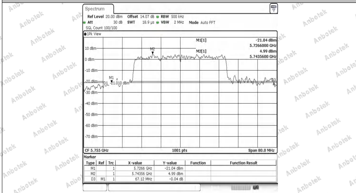
11AX40MIMO-Ant2-5755
