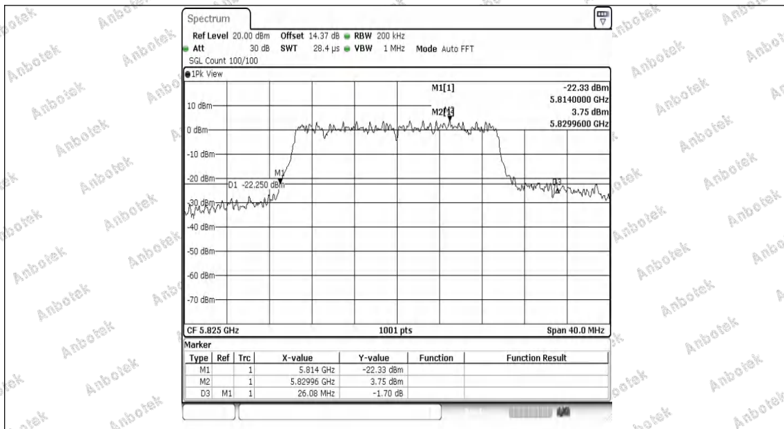
11AX20MIMO-Ant1-5825
