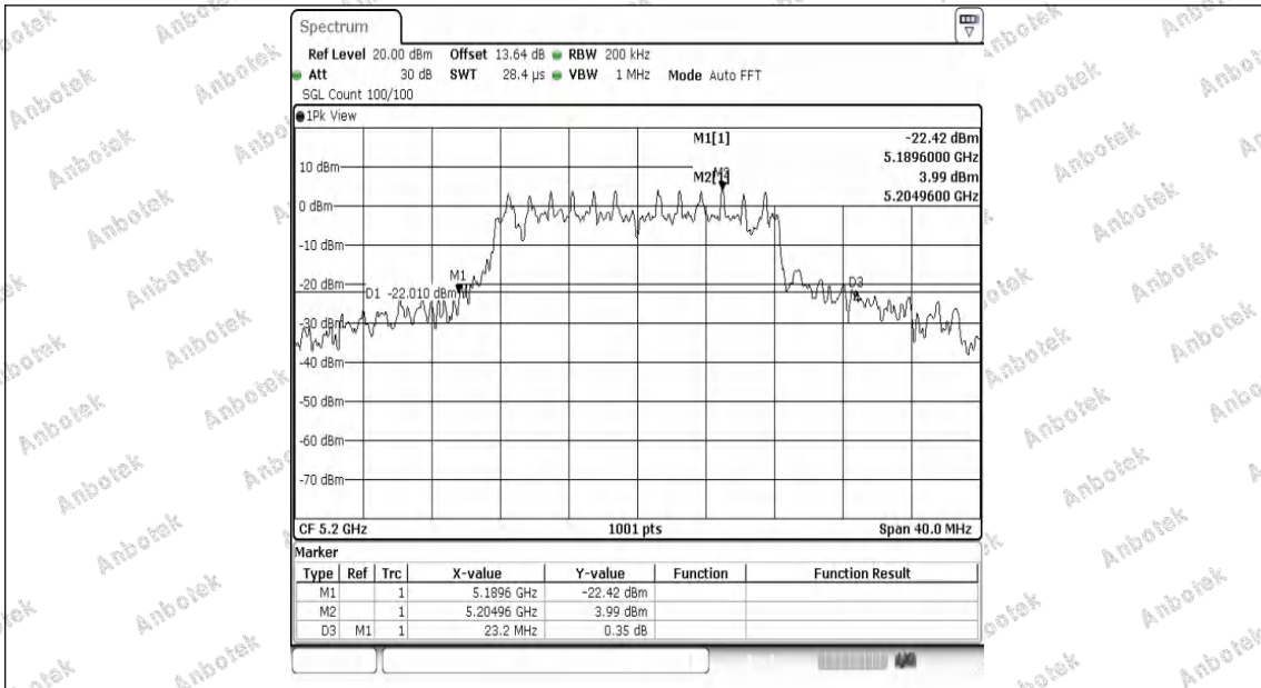
11N20MIMO-Ant1-5200
