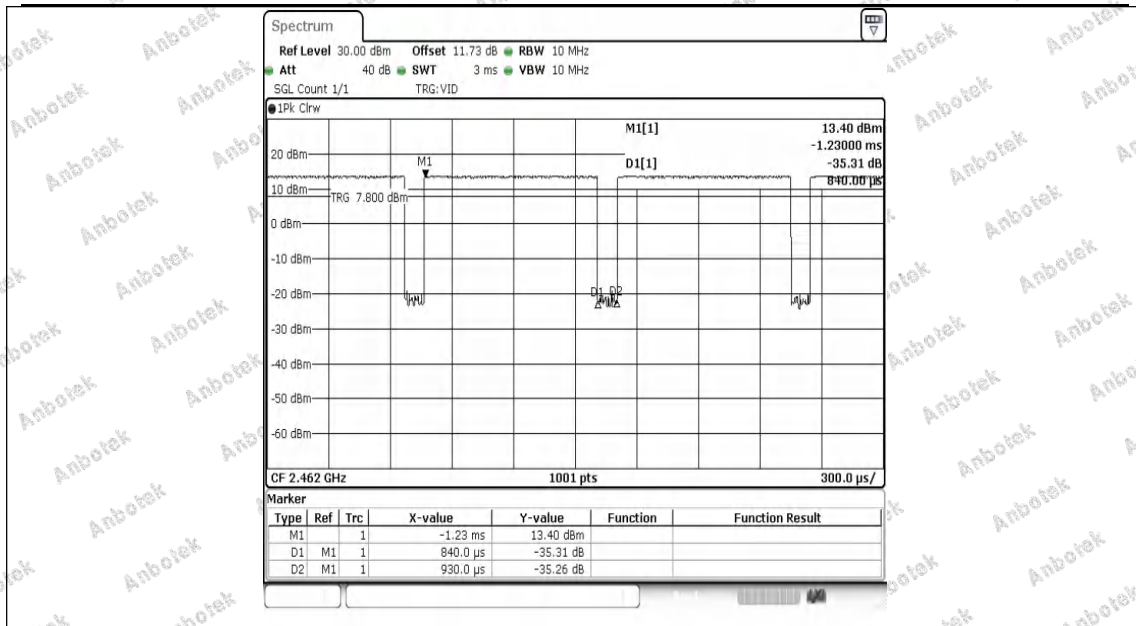
NTVN-11B-Ant1-2462
