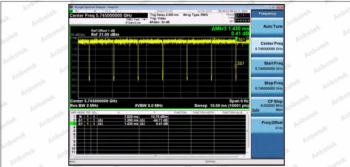
NTNV-11A-Ant1-5745
