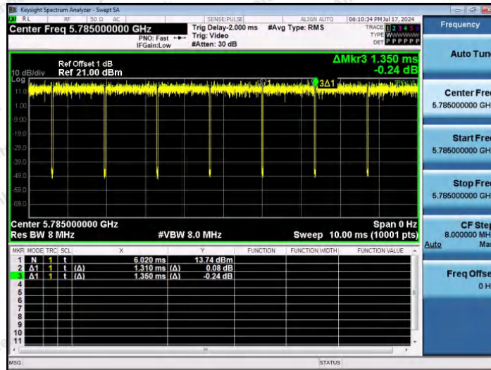
NTVN-11AC20SISO-Ant1-5785
