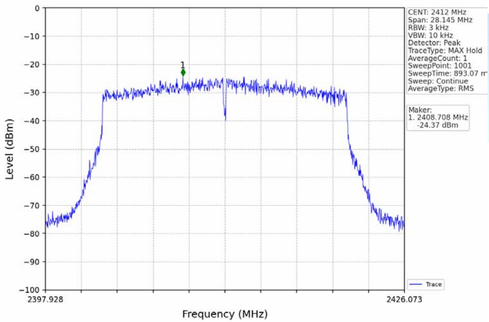
802.11ax(HEW20)_LCH_2412MHz_RU242_Left_Ant2 (MIMO)_NTNV
