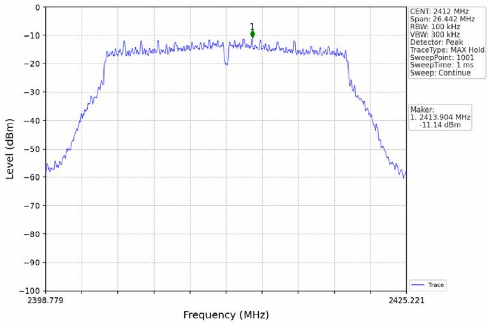
802.11n(HT20)_LCH_2412MHz_Ant2 (MIMO)_NTNV
