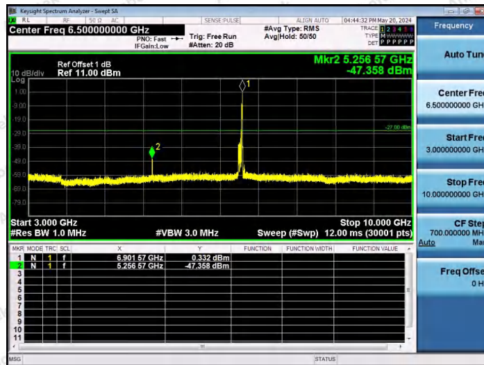
11AX80SISO-Ant1-6865-52Tone-RU52-3000~10000-PASS
