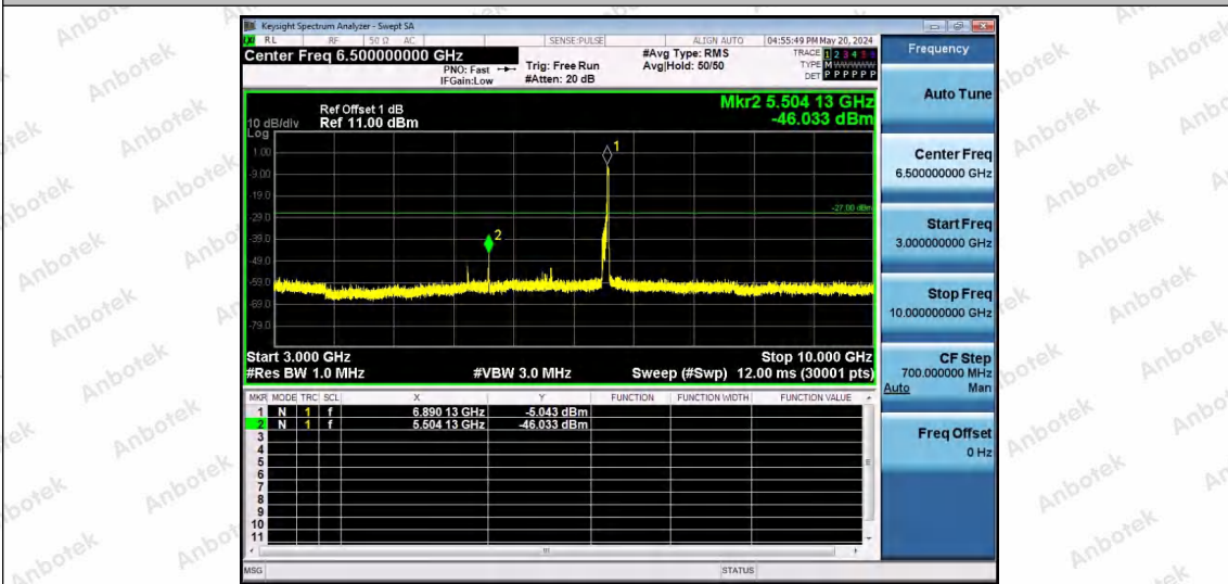
11AX80SISO-Ant1-6865-242Tone-RU64-3000~10000-PASS
