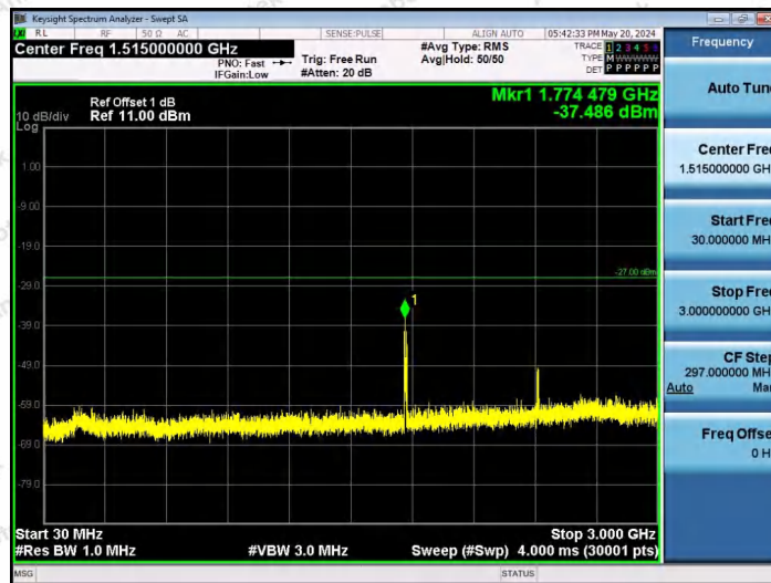
11AX80SISO-Ant1-7025-106Tone-RU60-30~3000-PASS
