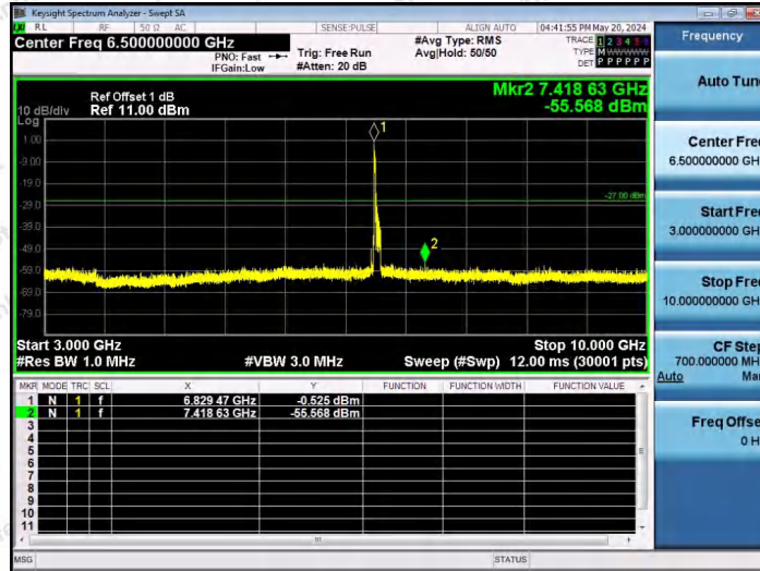
11AX80SISO-Ant1-6865-52Tone-RU37-3000~10000-PASS
