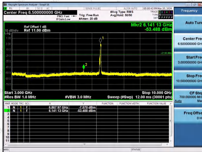
11AX80SISO-Ant1-6865-484Tone-RU66-3000~10000-PASS
