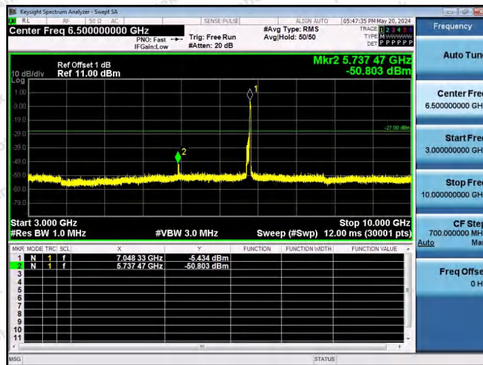
11AX80SISO-Ant1-7025-242Tone-RU64-3000~10000-PASS
