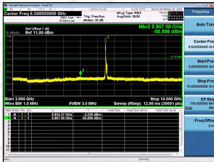
11AX80SISO-Ant1-6865-106Tone-RU53-3000~10000-PASS
