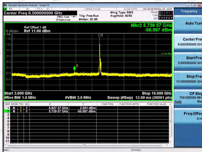
11AX80SISO-Ant1-6865-26Tone-RU0-3000~10000-PASS
