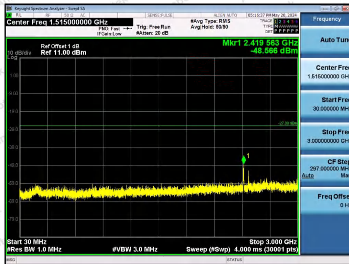
11AX80SISO-Ant1-6945-106Tone-RU60-30~3000-PASS
