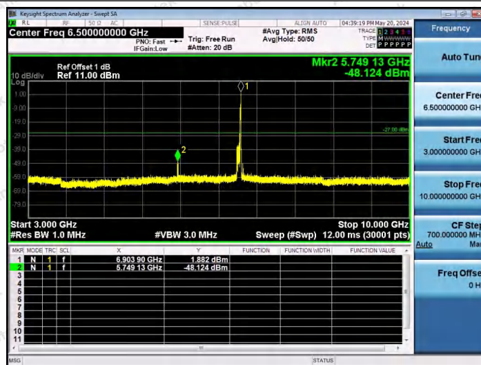
11AX80SISO-Ant1-6865-26Tone-RU36-3000~10000-PASS
