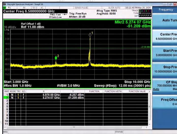
11AX80SISO-Ant1-6945-242Tone-RU64-3000~10000-PASS
