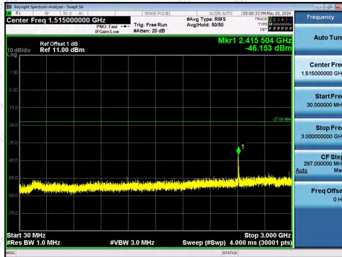
11AX80SISO-Ant1-6865-484Tone-RU66-30~3000-PASS
