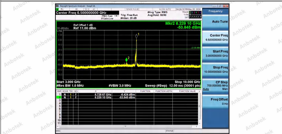
11AX80SISO-Ant1-6705-242Tone-RU64-3000~10000-PASS
