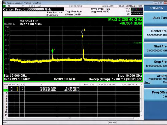
11AX80SISO-Ant1-6865-484Tone-RU65-3000~10000-PASS
