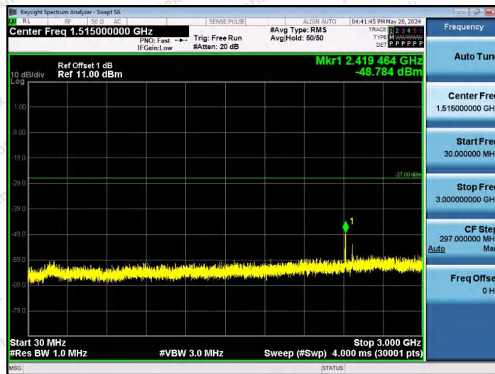
11AX80SISO-Ant1-6865-52Tone-RU37-30~3000-PASS
