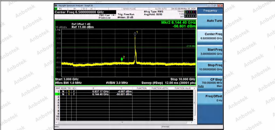
11AX80SISO-Ant1-6865-242Tone-RU61-3000~10000-PASS
