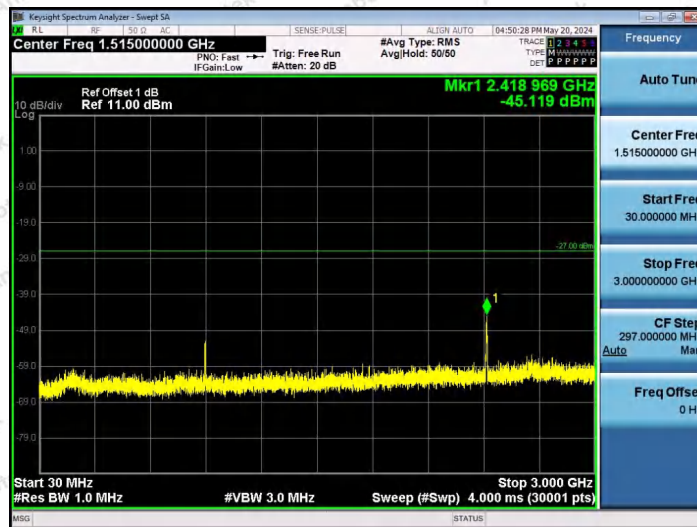
11AX80SISO-Ant1-6865-106Tone-RU60-30~3000-PASS
