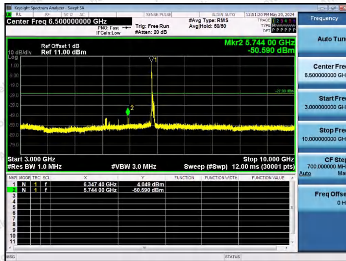
11AX80SISO-Ant1-6385-26Tone-RU0-3000~10000-PASS
