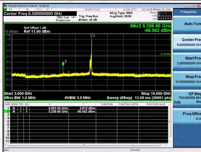
11AX80SISO-Ant1-6465-26Tone-RU36-3000~10000-PASS
