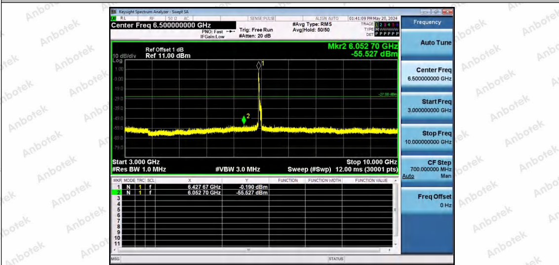
11AX80SISO-Ant1-6465-106Tone-RU53-3000~10000-PASS
