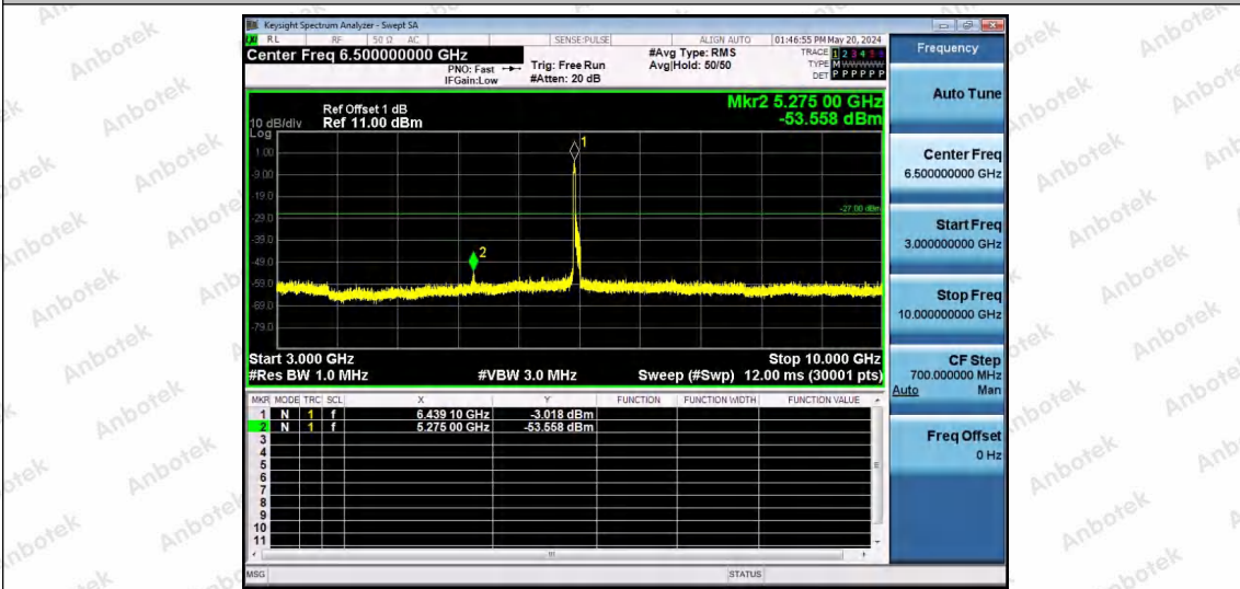
11AX80SISO-Ant1-6465-242Tone-RU61-3000~10000-PASS
