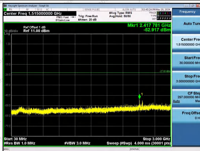
11AX80SISO-Ant1-6545-106Tone-RU60-30~3000-PASS
