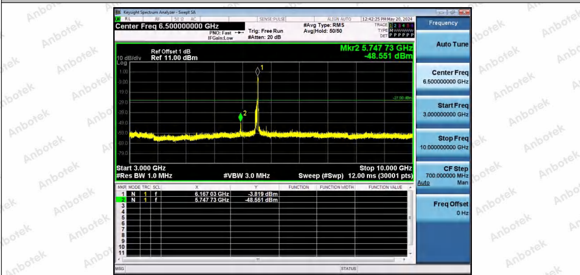
11AX80SISO-Ant1-6145-242Tone-RU64-3000~10000-PASS
