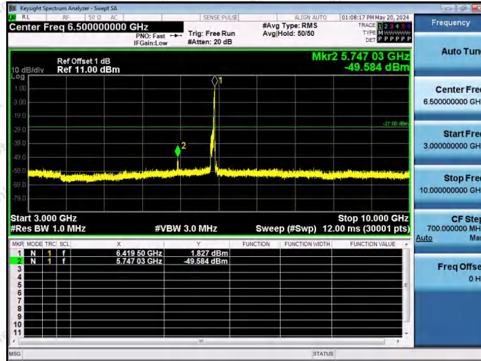
11AX80SISO-Ant1-6385-106Tone-RU60-3000~10000-PASS
