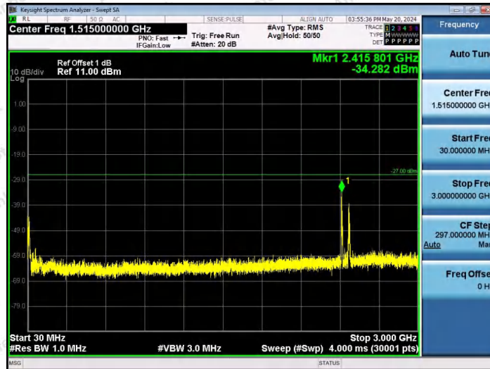
11AX80SISO-Ant1-6545-484Tone-RU66-30~3000-PASS
