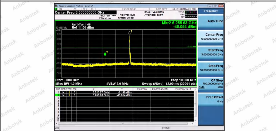
11AX80SISO-Ant1-6545-106Tone-RU53-3000~10000-PASS
