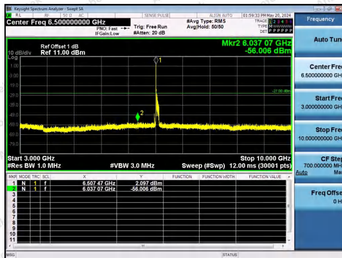
11AX80SISO-Ant1-6545-26Tone-RU0-3000~10000-PASS
