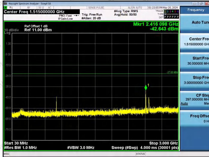
11AX80SISO-Ant1-6385-484Tone-RU66-30~3000-PASS
