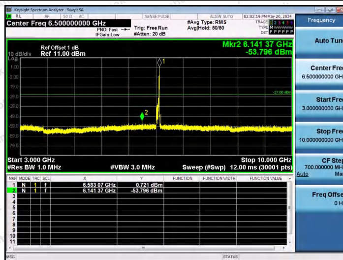
11AX80SISO-Ant1-6545-26Tone-RU36-3000~10000-PASS
