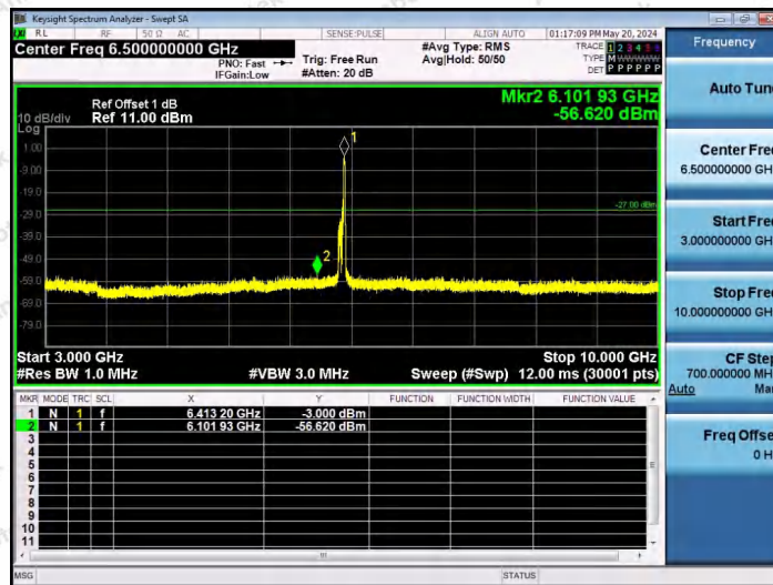
11AX80SISO-Ant1-6385-242Tone-RU64-3000~10000-PASS
