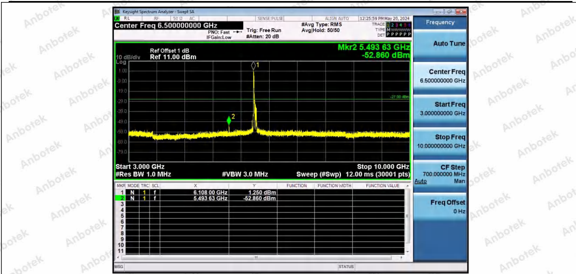
11AX80SISO-Ant1-6145-52Tone-RU37-3000~10000-PASS
