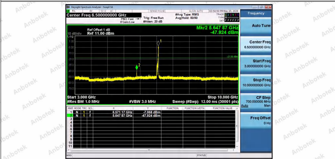
11AX80SISO-Ant1-6545-242Tone-RU64-3000~10000-PASS
