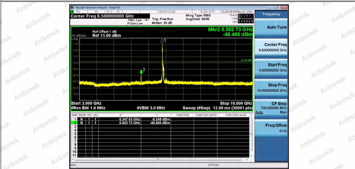
11AX80SISO-Ant1-6385-106Tone-RU53-3000~10000-PASS
