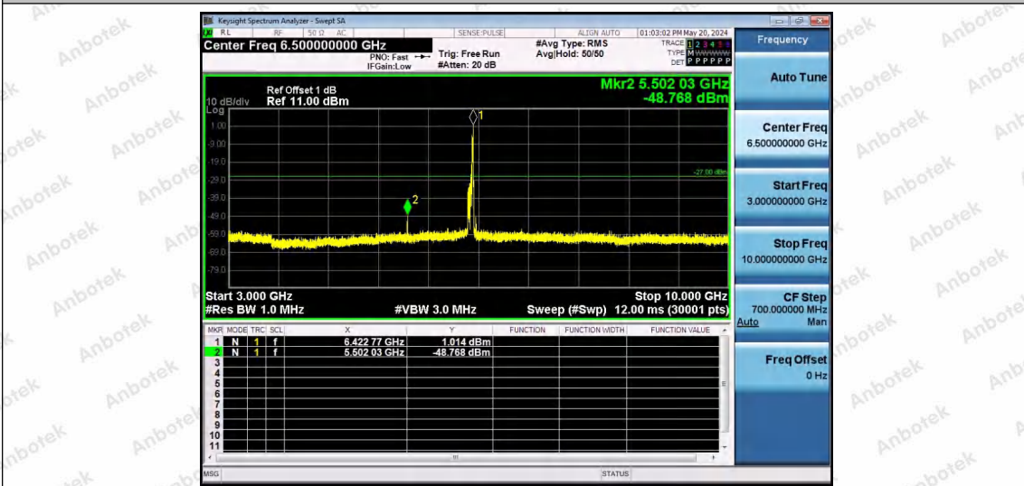
11AX80SISO-Ant1-6385-52Tone-RU52-3000~10000-PASS
