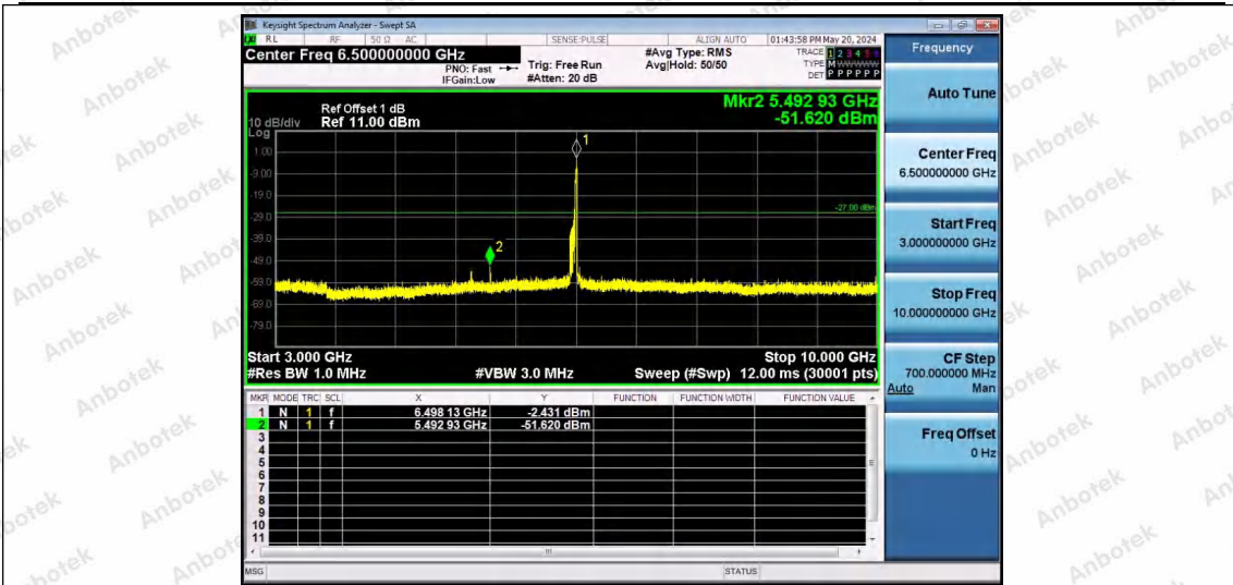
11AX80SISO-Ant1-6465-106Tone-RU60-3000~10000-PASS
