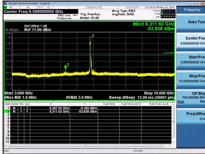
11AX80SISO-Ant1-6385-484Tone-RU65-3000~10000-PASS
