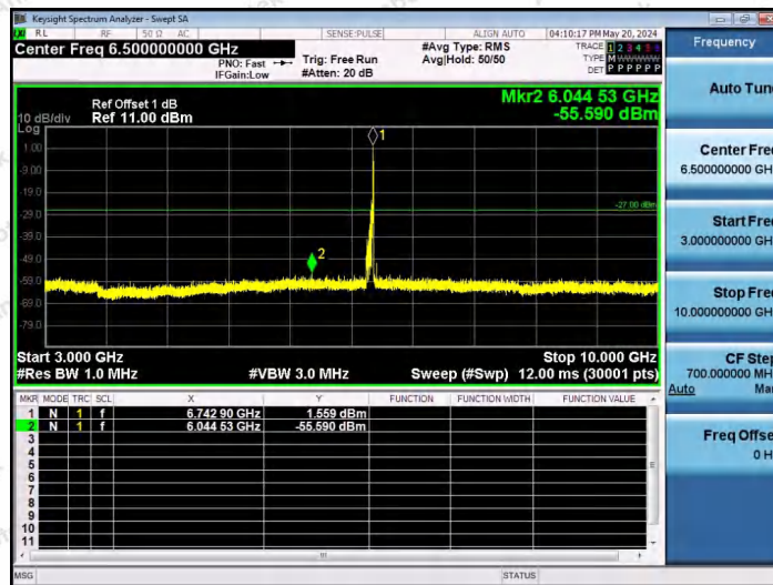
11AX80SISO-Ant1-6705-26Tone-RU36-3000~10000-PASS
