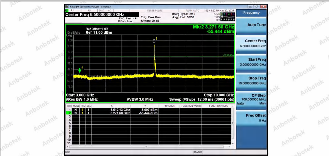
11AX80SISO-Ant1-6545-242Tone-RU61-3000~10000-PASS
