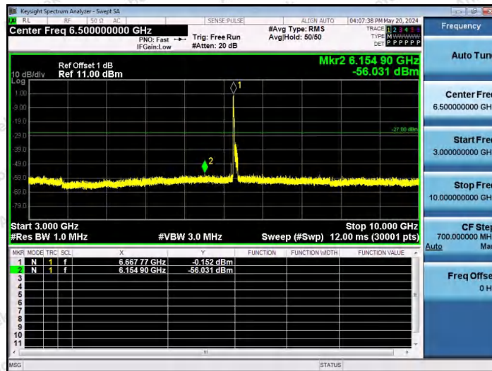
11AX80SISO-Ant1-6705-26Tone-RU0-3000~10000-PASS
