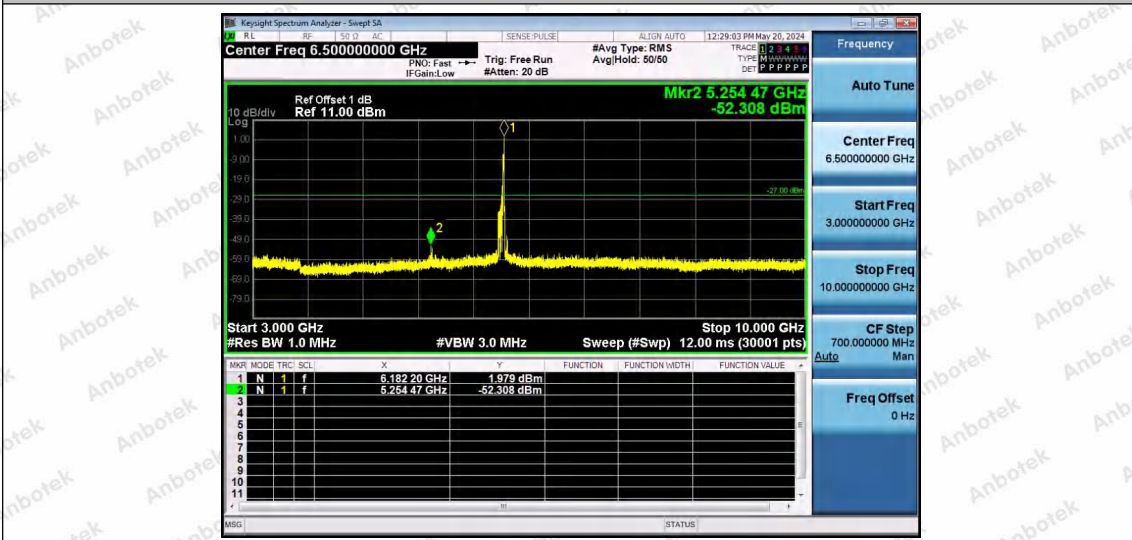
11AX80SISO-Ant1-6145-52Tone-RU52-3000~10000-PASS
