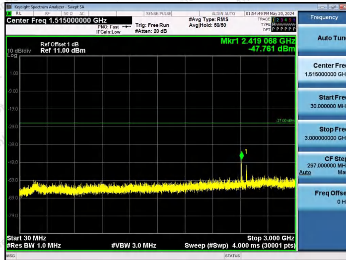
11AX80SISO-Ant1-6465-484Tone-RU66-30~3000-PASS
