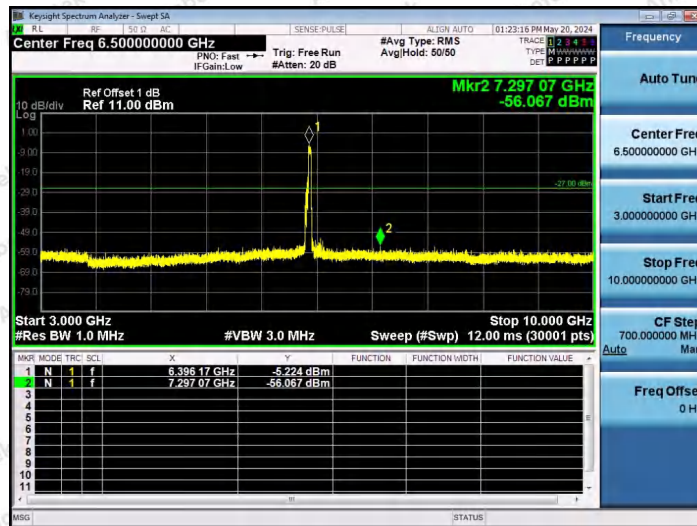
11AX80SISO-Ant1-6385-484Tone-RU66-3000~10000-PASS
