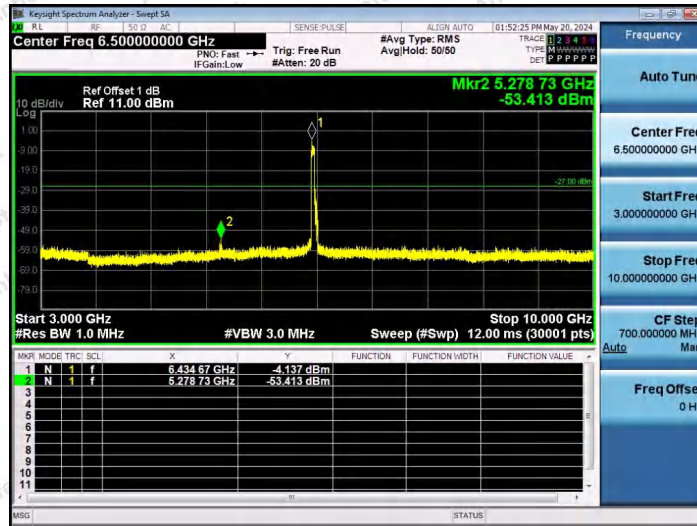
11AX80SISO-Ant1-6465-484Tone-RU65-3000~10000-PASS
