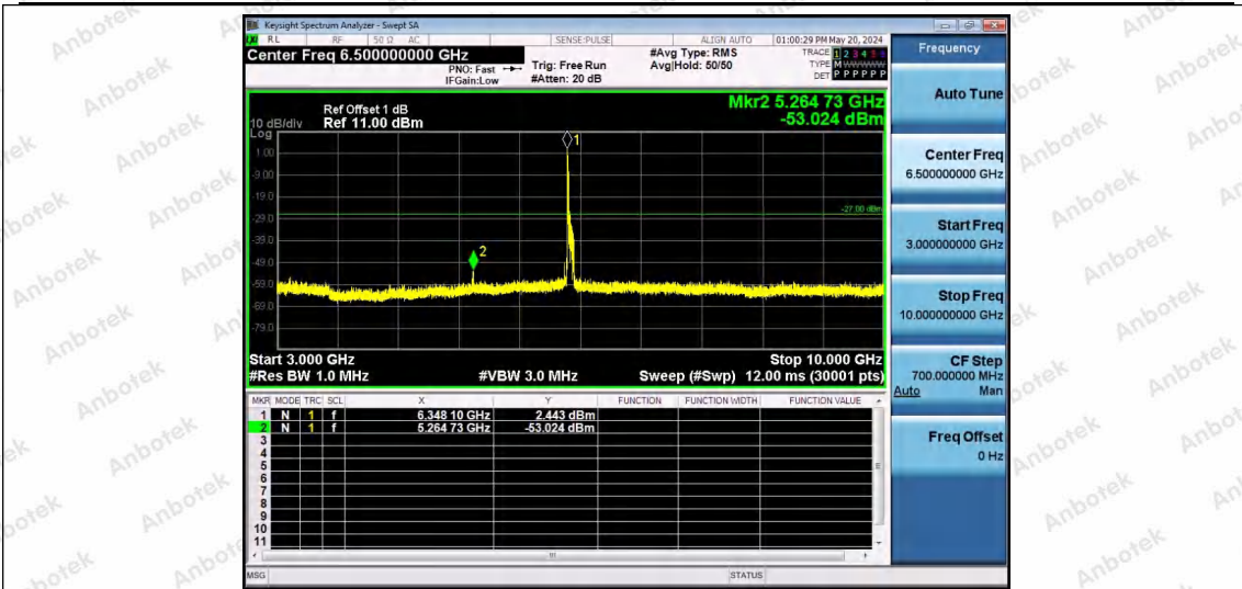
11AX80SISO-Ant1-6385-52Tone-RU37-3000~10000-PASS
