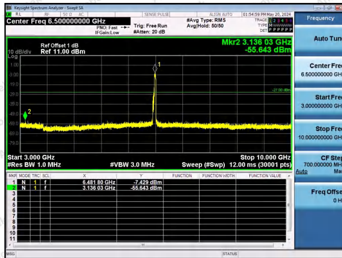
11AX80SISO-Ant1-6465-484Tone-RU66-3000~10000-PASS
