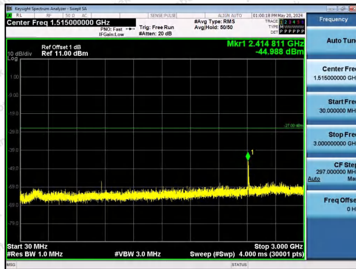
11AX80SISO-Ant1-6385-52Tone-RU37-30~3000-PASS
