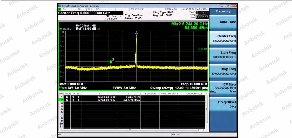
11AX80SISO-Ant1-6465-52Tone-RU52-3000~10000-PASS
