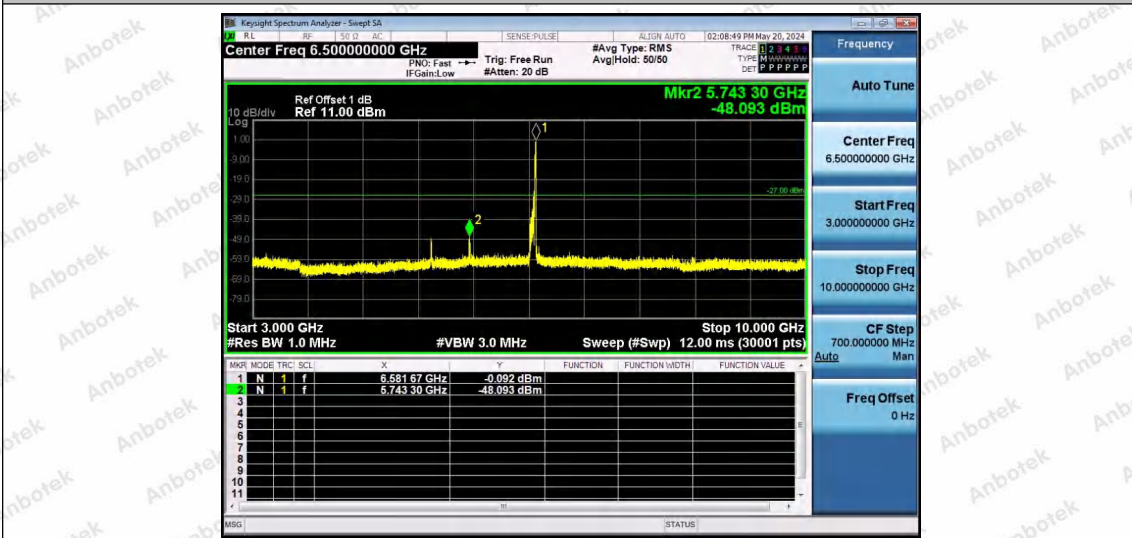
11AX80SISO-Ant1-6545-52Tone-RU52-3000~10000-PASS
