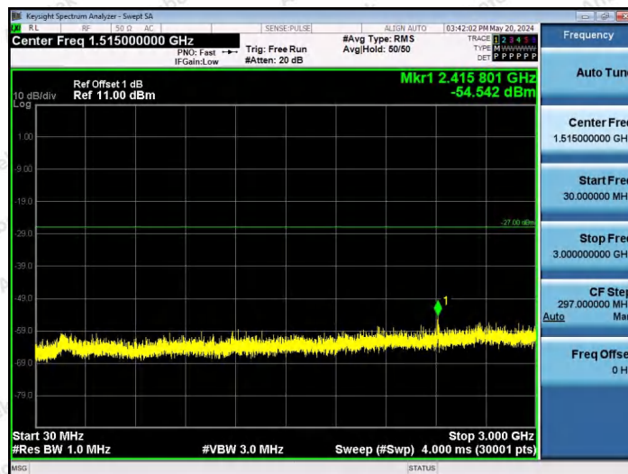
11AX80SISO-Ant1-6545-106Tone-RU53-30~3000-PASS
