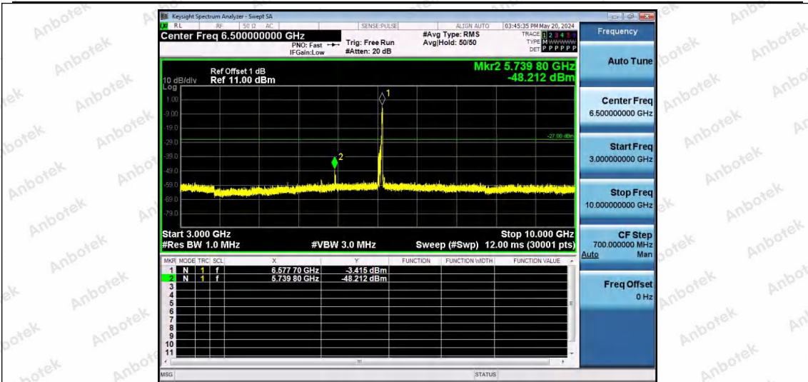
11AX80SISO-Ant1-6545-106Tone-RU60-3000~10000-PASS
