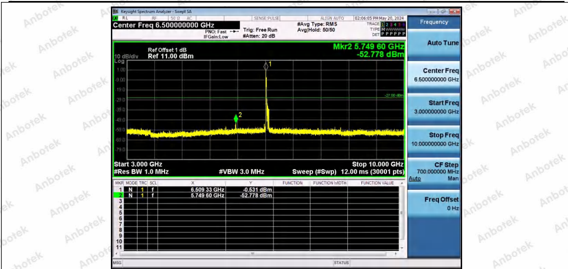
11AX80SISO-Ant1-6545-52Tone-RU37-3000~10000-PASS
