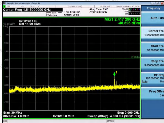
11AX80SISO-Ant1-6545-52Tone-RU52-30~3000-PASS
