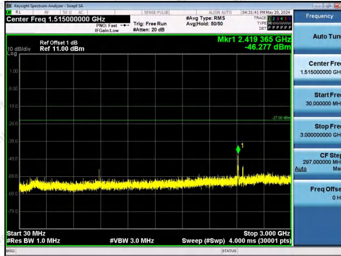
11AX80SISO-Ant1-6705-484Tone-RU66-30~3000-PASS
