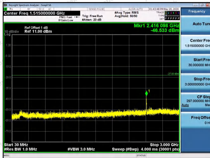
11AX80SISO-Ant1-6465-106Tone-RU60-30~3000-PASS
