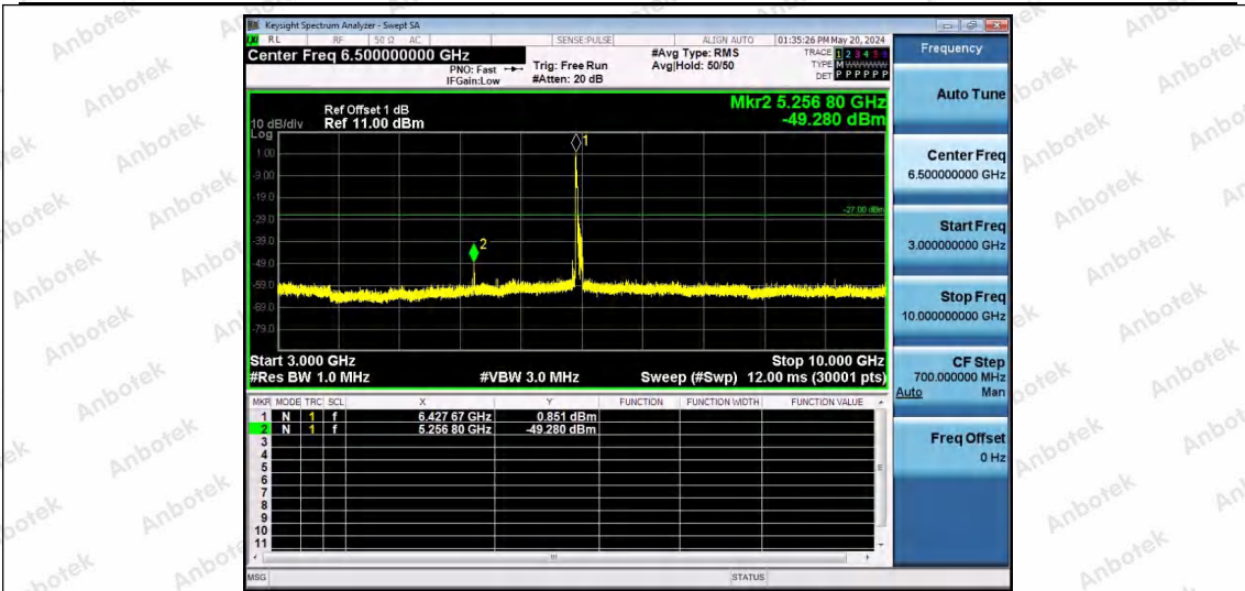
11AX80SISO-Ant1-6465-52Tone-RU37-3000~10000-PASS
