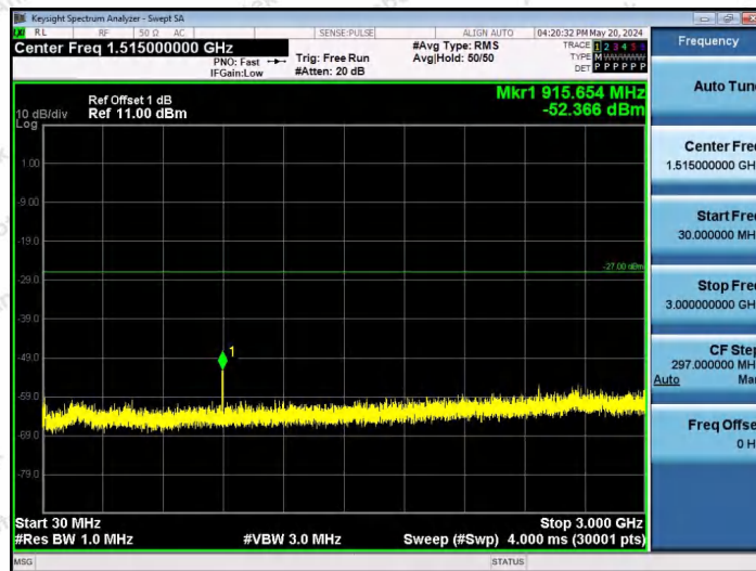
11AX80SISO-Ant1-6705-106Tone-RU60-30~3000-PASS
