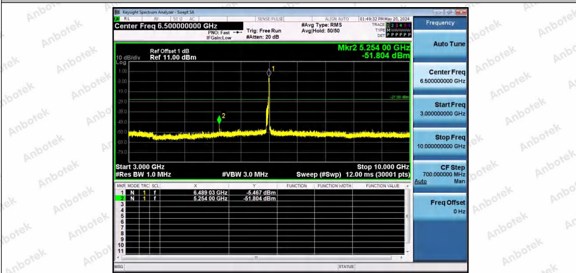
11AX80SISO-Ant1-6465-242Tone-RU64-3000~10000-PASS
