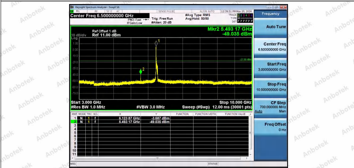
11AX80SISO-Ant1-6145-242Tone-RU61-3000~10000-PASS
