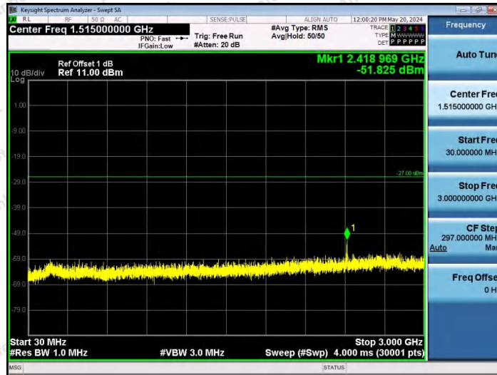
11AX80SISO-Ant1-5985-52Tone-RU52-30~3000-PASS
