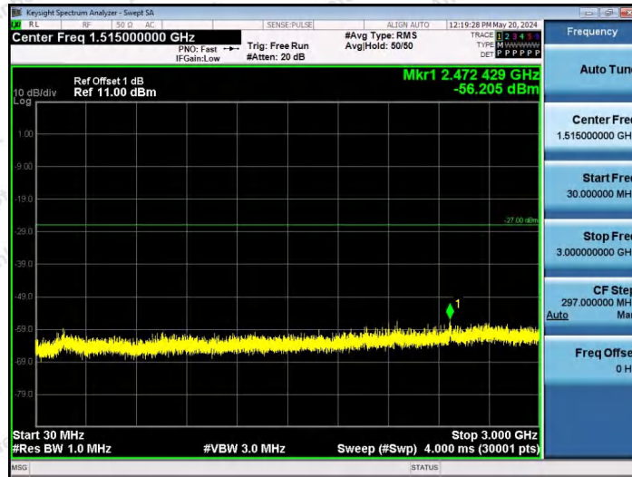
11AX80SISO-Ant1-6145-26Tone-RU0-30~3000-PASS
