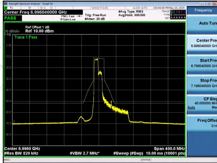
NTVN-11AX80SISO-Ant1-7025-106Tone-RU53-PASS
