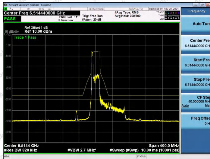
NTNV-11AX80SISO-Ant1-6545-26Tone-RU0-PASS
