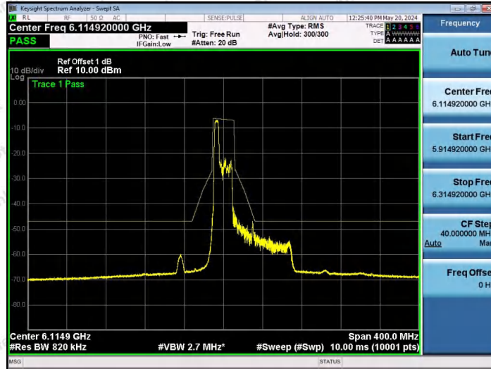
NTNV-11AX80SISO-Ant1-6145-52Tone-RU37-PASS
