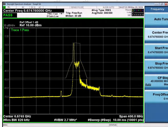
NTNV-11AX80SISO-Ant1-6705-26Tone-RU0-PASS
