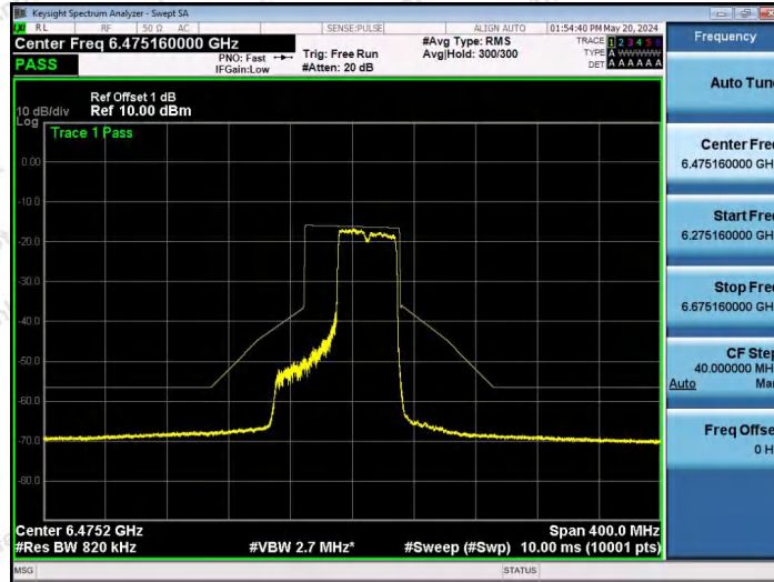
NTNV-11AX80SISO-Ant1-6465-484Tone-RU66-PASS
