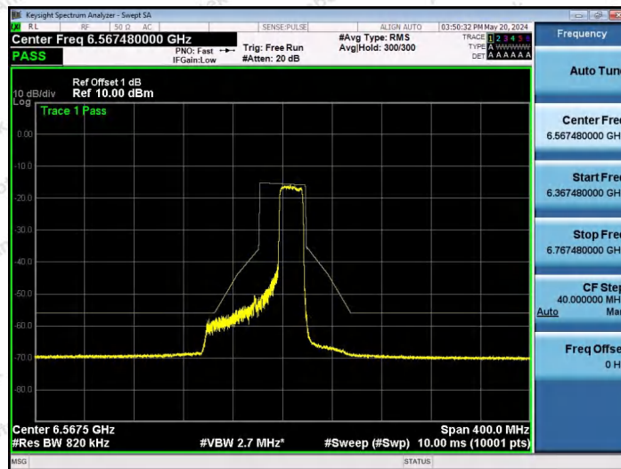
NTNV-11AX80SISO-Ant1-6545-242Tone-RU64-PASS
