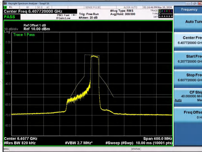
NTVN-11AX80SISO-Ant1-6385-242Tone-RU64-PASS
