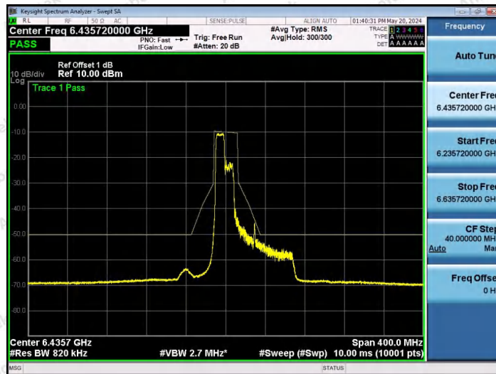
NTNV-11AX80SISO-Ant1-6465-106Tone-RU53-PASS
