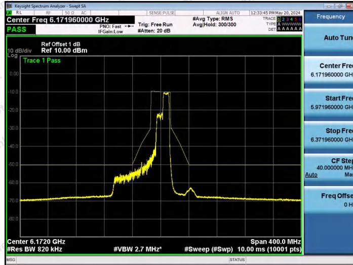
NTNV-11AX80SISO-Ant1-6145-106Tone-RU60-PASS
