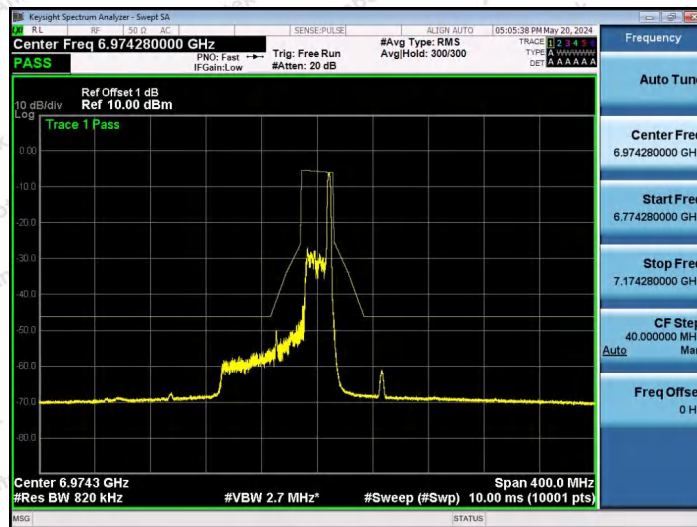
NTNV-11AX80SISO-Ant1-6945-26Tone-RU36-PASS
