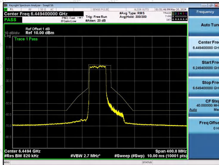
NTVN-11AX80SISO-Ant1-6465-484Tone-RU65-PASS
