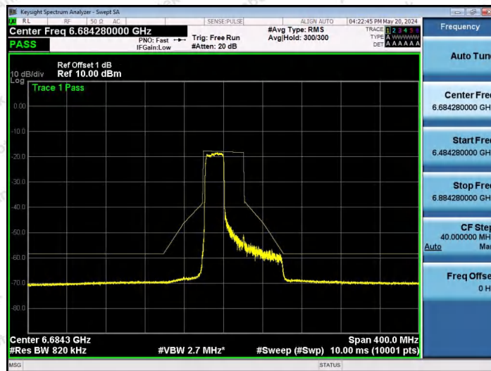
NTNV-11AX80SISO-Ant1-6705-242Tone-RU61-PASS
