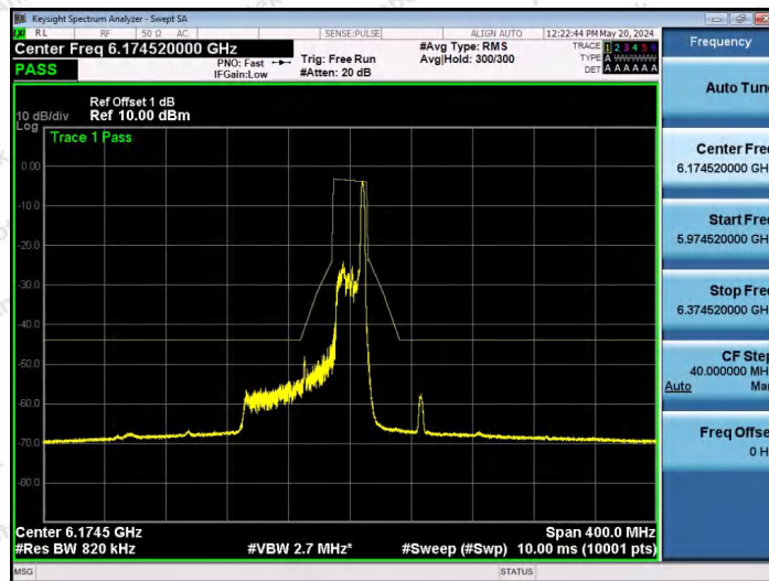
NTNV-11AX80SISO-Ant1-6145-26Tone-RU36-PASS
