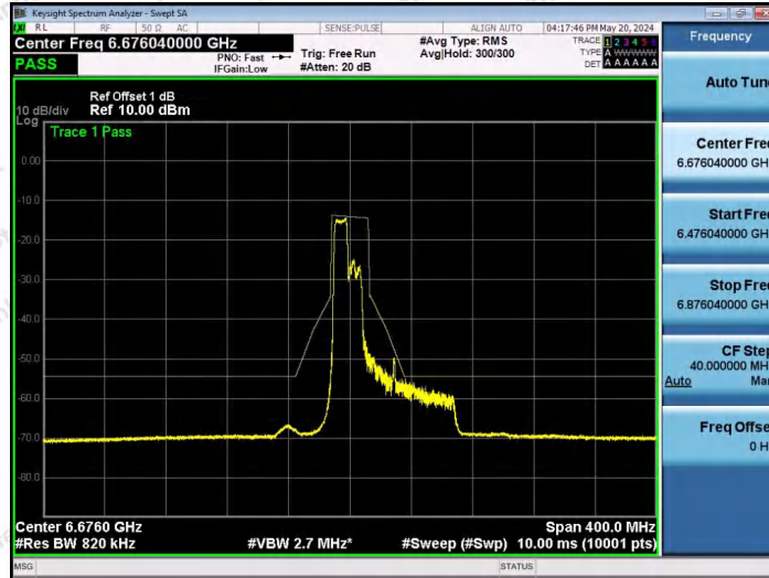
NTNV-11AX80SISO-Ant1-6705-106Tone-RU53-PASS
