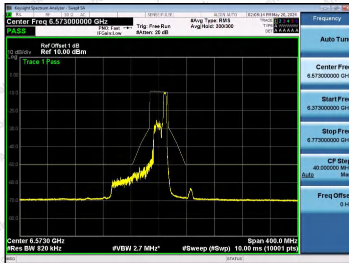
NTNV-11AX80SISO-Ant1-6545-52Tone-RU52-PASS
