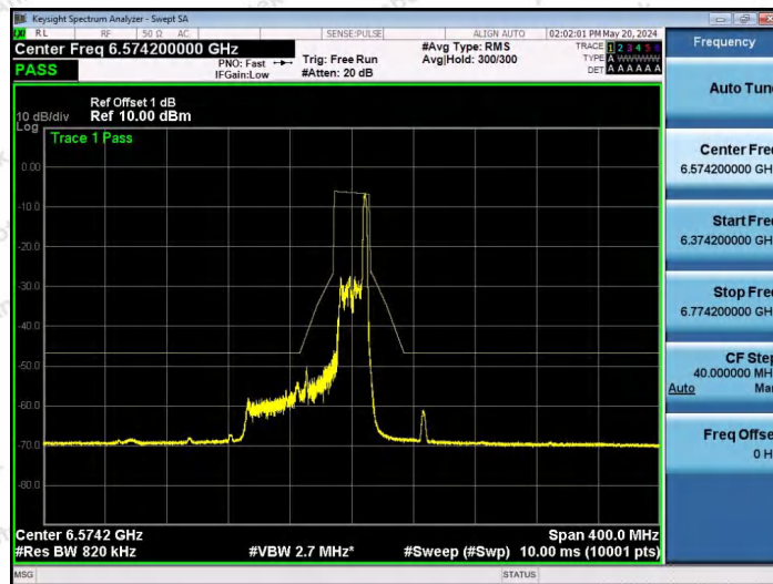
NTNV-11AX80SISO-Ant1-6545-26Tone-RU36-PASS
