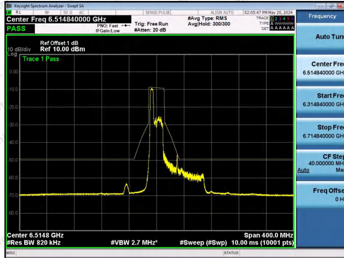
NTNV-11AX80SISO-Ant1-6545-52Tone-RU37-PASS
