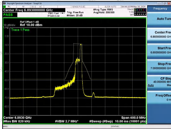
NTNV-11AX80SISO-Ant1-6865-52Tone-RU52-PASS
