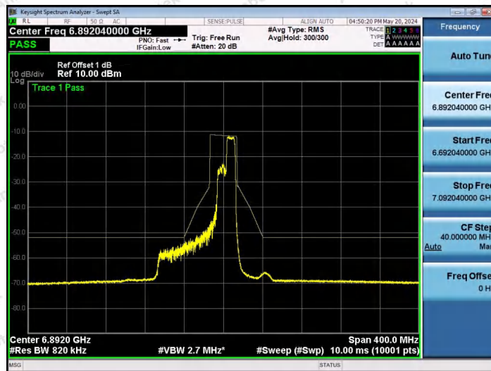
NTNV-11AX80SISO-Ant1-6865-106Tone-RU60-PASS
