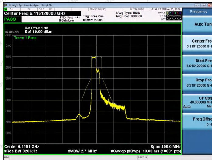
NTNV-11AX80SISO-Ant1-6145-106Tone-RU53-PASS
