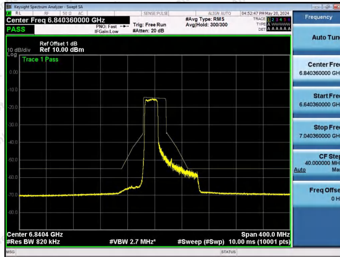
NTNV-11AX80SISO-Ant1-6865-242Tone-RU61-PASS
