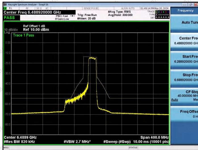
NTVN-11AX80SISO-Ant1-6465-242Tone-RU64-PASS
