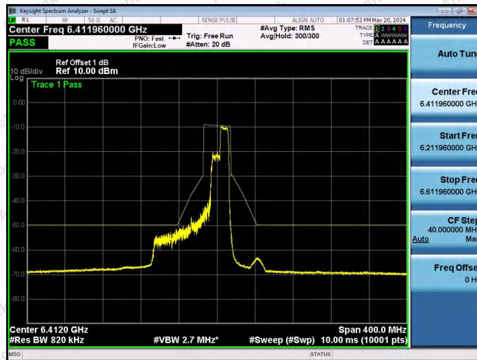
NTVN-11AX80SISO-Ant1-6385-106Tone-RU60-PASS
