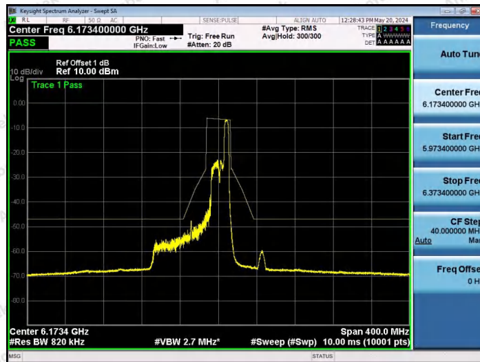
NTNV-11AX80SISO-Ant1-6145-52Tone-RU52-PASS
