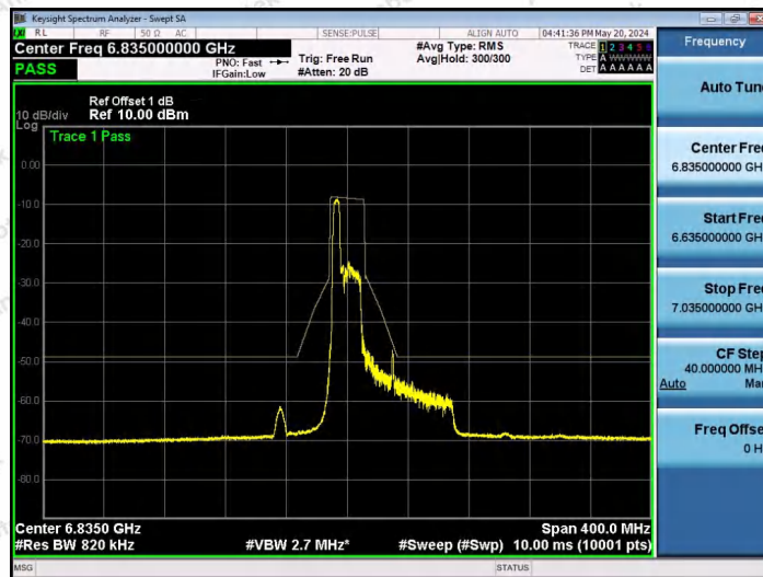
NTNV-11AX80SISO-Ant1-6865-52Tone-RU37-PASS
