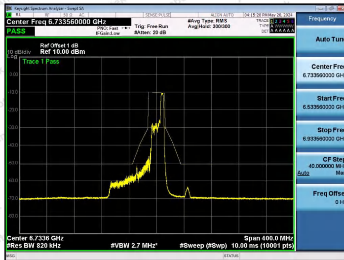
NTNV-11AX80SISO-Ant1-6705-52Tone-RU52-PASS
