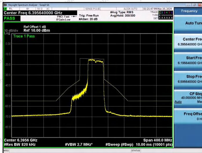
NTVN-11AX80SISO-Ant1-6385-484Tone-RU66-PASS
