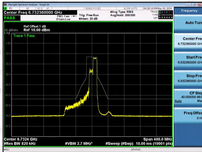
NTNV-11AX80SISO-Ant1-6705-106Tone-RU60-PASS
