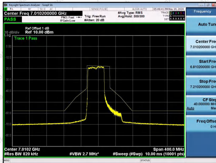
NTNV-11AX80SISO-Ant1-7025-484Tone-RU65-PASS
