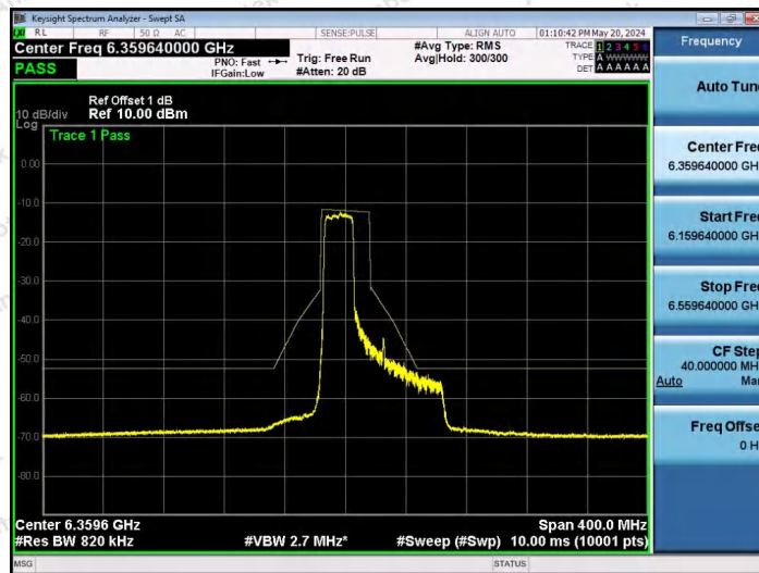
NTVN-11AX80SISO-Ant1-6385-242Tone-RU61-PASS
