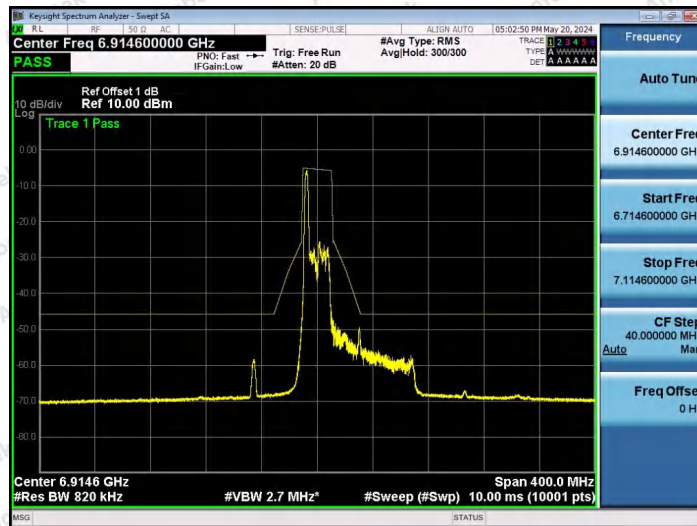
NTNV-11AX80SISO-Ant1-6945-26Tone-RU0-PASS
