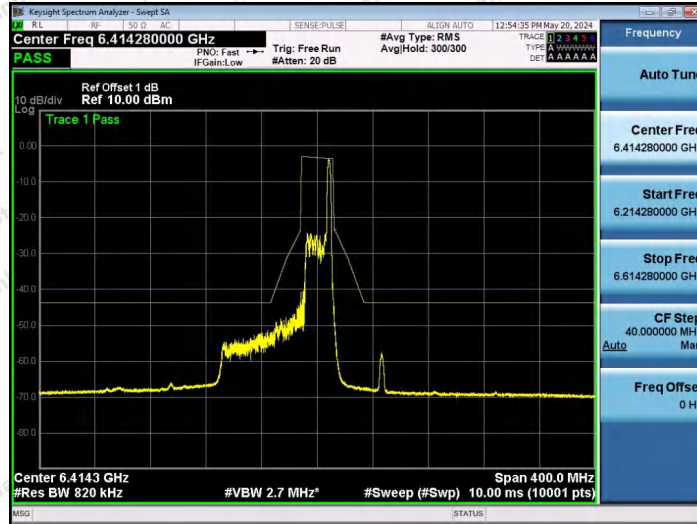
NTNV-11AX80SISO-Ant1-6385-26Tone-RU36-PASS
