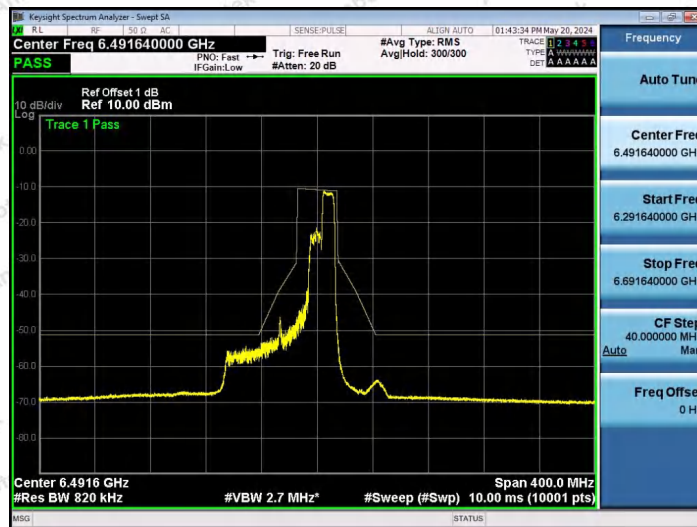
NTNV-11AX80SISO-Ant1-6465-106Tone-RU60-PASS
