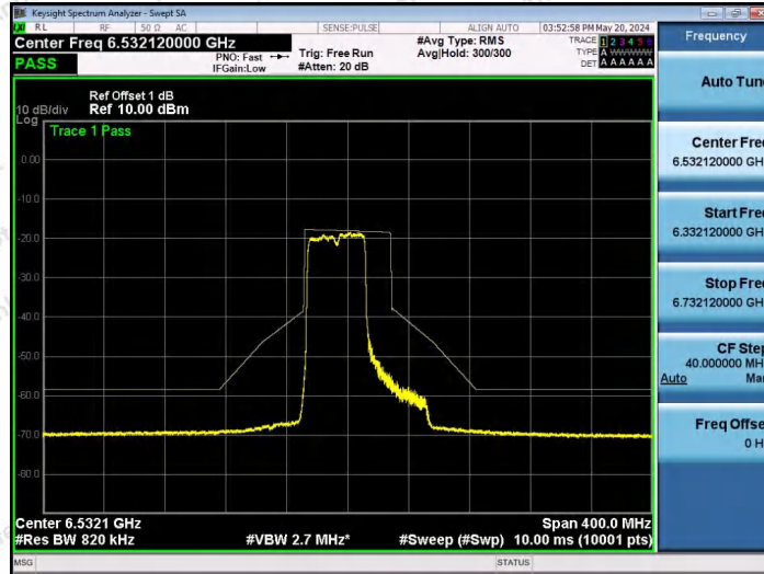
NTNV-11AX80SISO-Ant1-6545-484Tone-RU65-PASS
