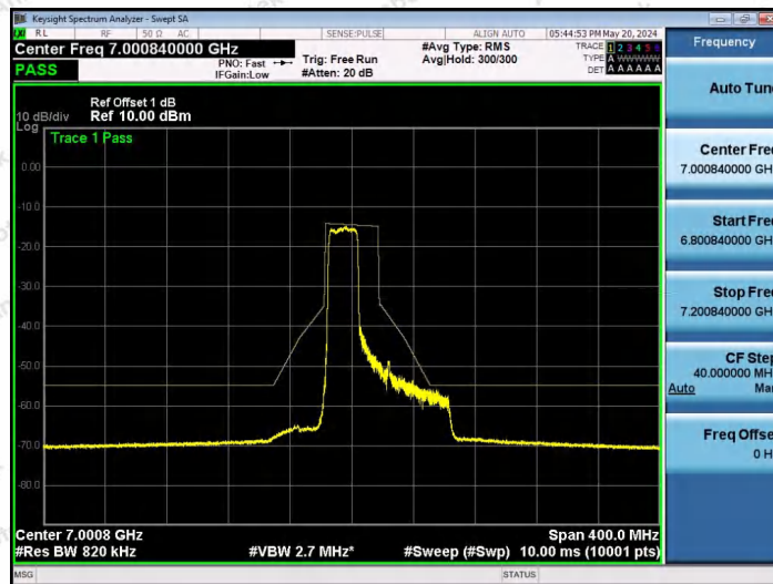
NTVN-11AX80SISO-Ant1-7025-242Tone-RU61-PASS
