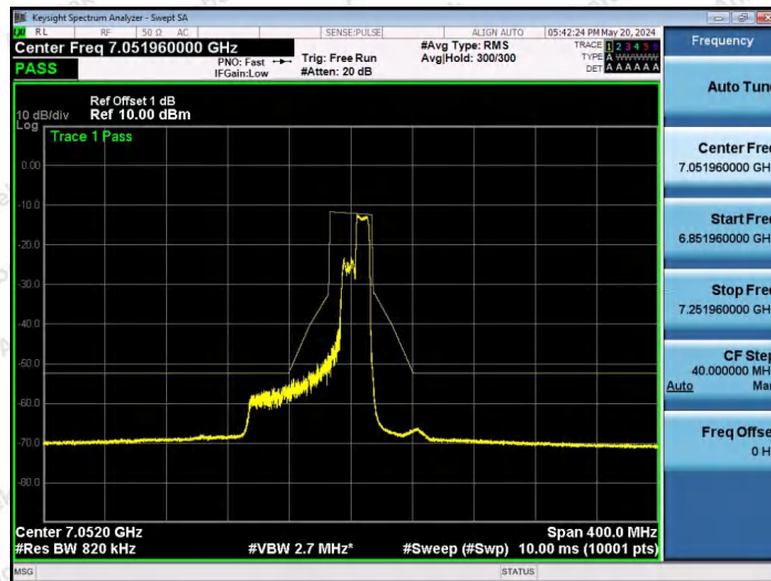
NTVN-11AX80SISO-Ant1-7025-106Tone-RU60-PASS
