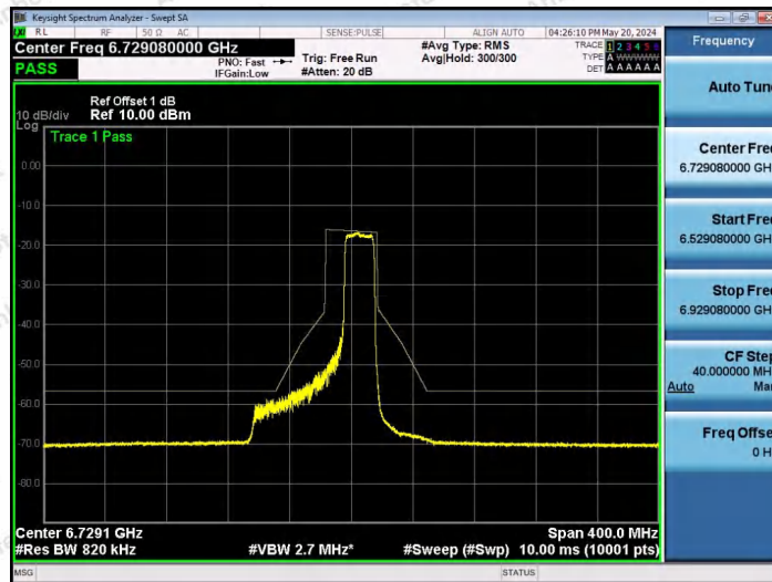
NTNV-11AX80SISO-Ant1-6705-242Tone-RU64-PASS
