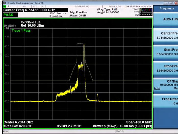
NTNV-11AX80SISO-Ant1-6705-26Tone-RU36-PASS
