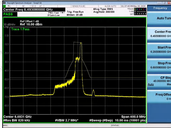
NTNV-11AX80SISO-Ant1-6465-52Tone-RU52-PASS
