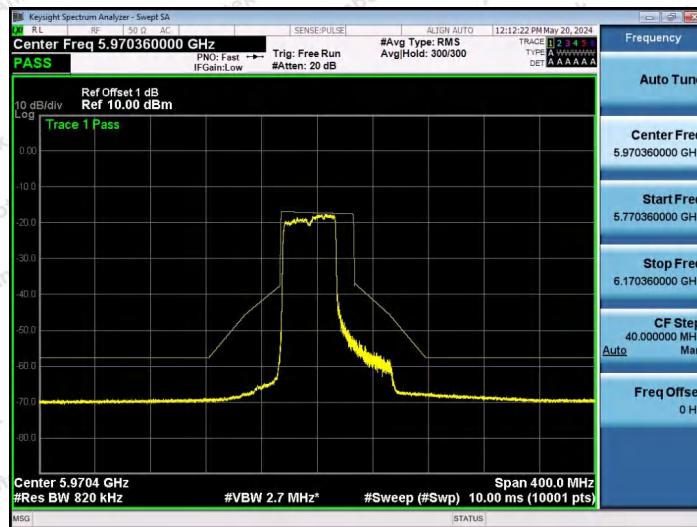
NTVN-11AX80SISO-Ant1-5985-484Tone-RU65-PASS
