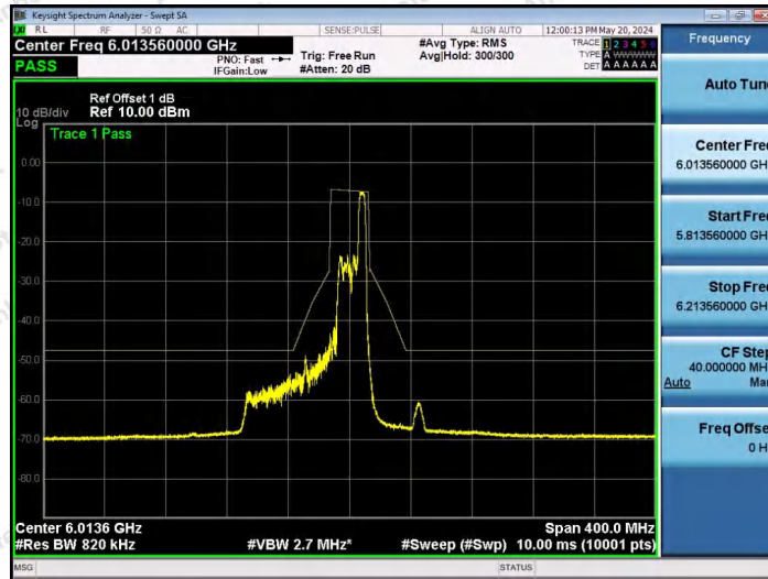
NTNV-11AX80SISO-Ant1-5985-52Tone-RU52-PASS
