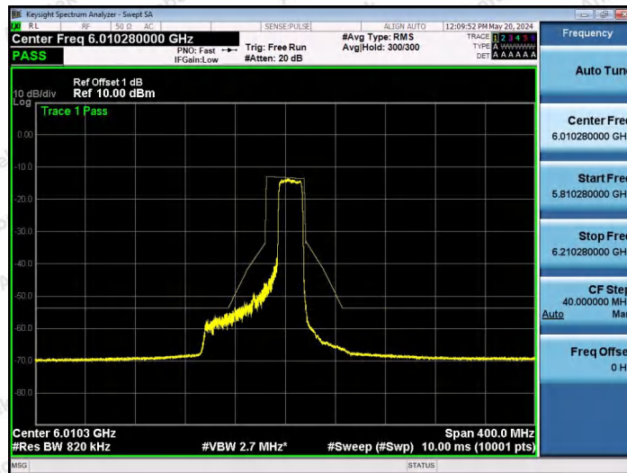
NTVN-11AX80SISO-Ant1-5985-242Tone-RU64-PASS
