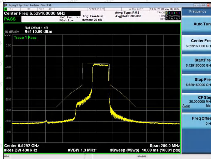
NTNV-11AX40SISO-Ant1-6525-242Tone-RU62-PASS
