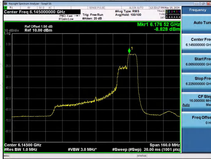
11AX80SISO-Ant1-6145-106Tone-RU60-PASS
