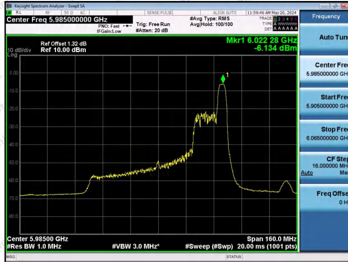
11AX80SISO-Ant1-5985-52Tone-RU52-PASS
