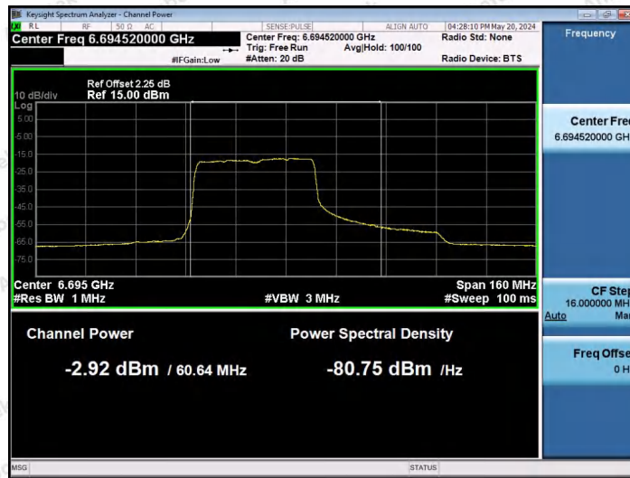
11AX80SISO-Ant1-6705-484Tone-RU65-PASS
