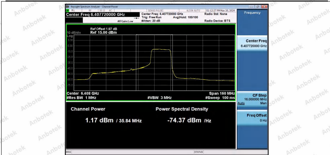
11AX80SISO-Ant1-6385-242Tone-RU64-PASS
