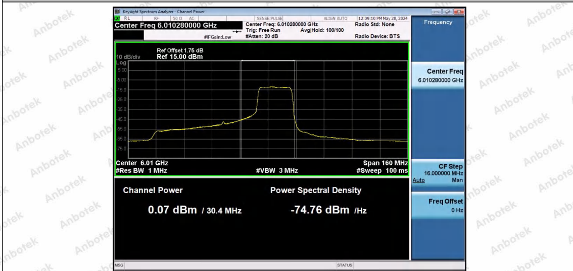
11AX80SISO-Ant1-5985-242Tone-RU64-PASS
