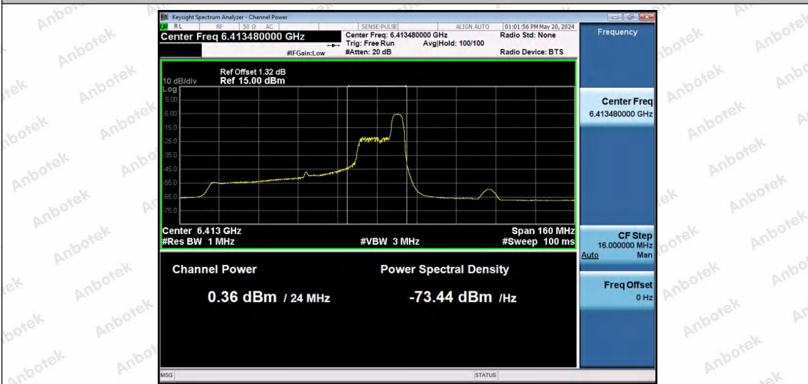
11AX80SISO-Ant1-6385-52Tone-RU52-PASS
