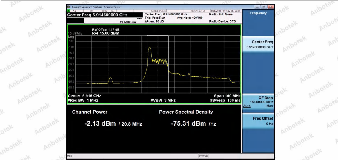
11AX80SISO-Ant1-6945-26Tone-RU0-PASS
