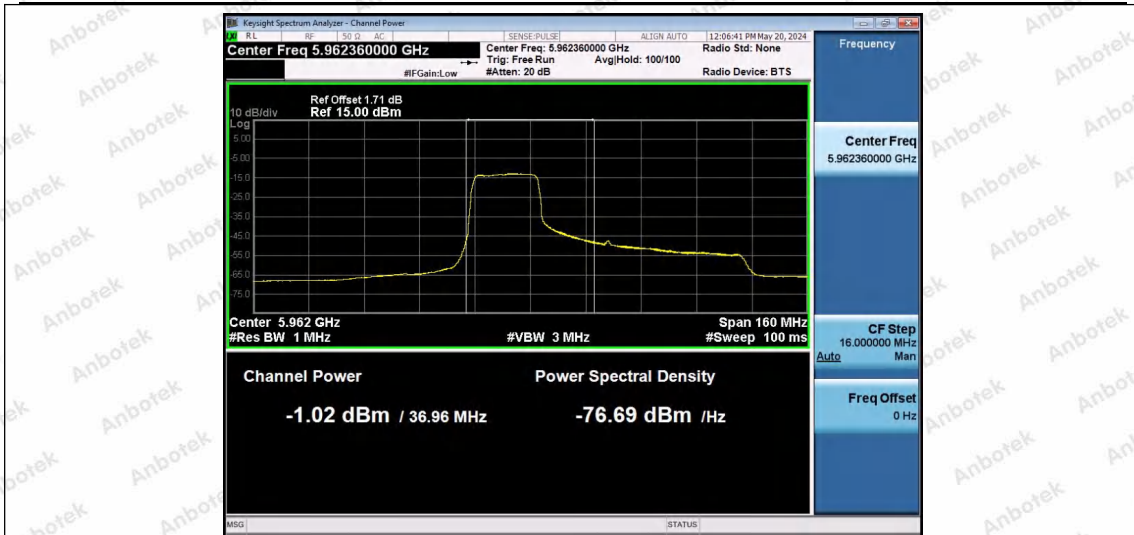
11AX80SISO-Ant1-5985-242Tone-RU61-PASS
