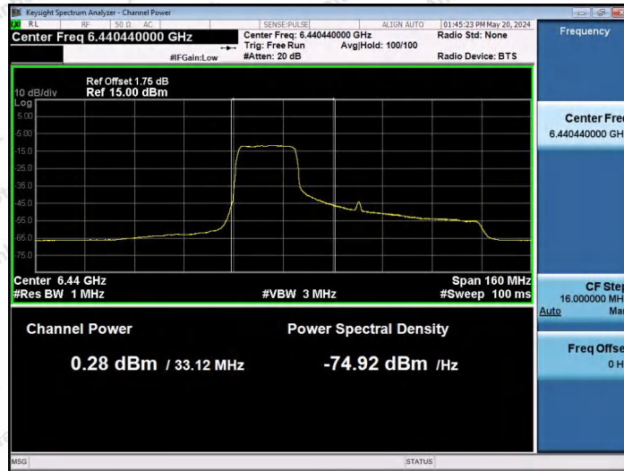
11AX80SISO-Ant1-6465-242Tone-RU61-PASS
