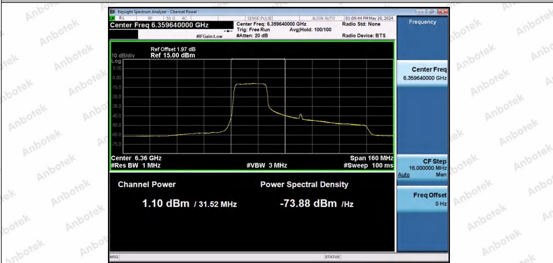
11AX80SISO-Ant1-6385-242Tone-RU61-PASS
