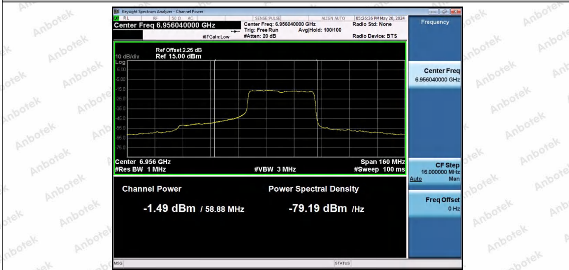
11AX80SISO-Ant1-6945-484Tone-RU66-PASS
