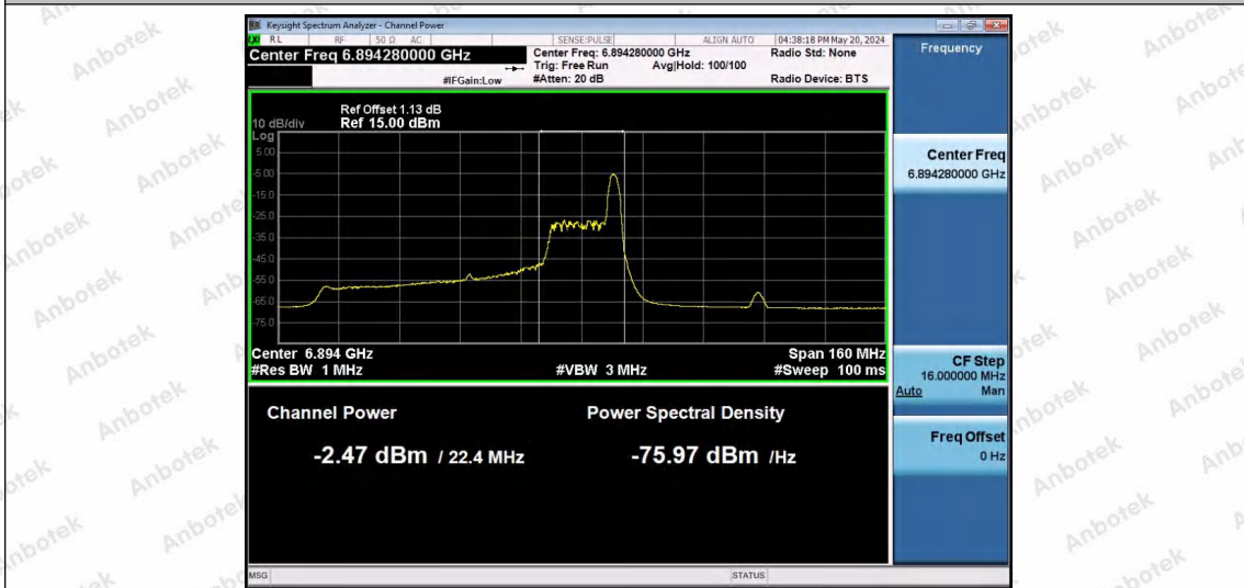
11AX80SISO-Ant1-6865-26Tone-RU36-PASS
