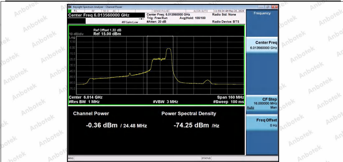
11AX80SISO-Ant1-5985-52Tone-RU52-PASS
