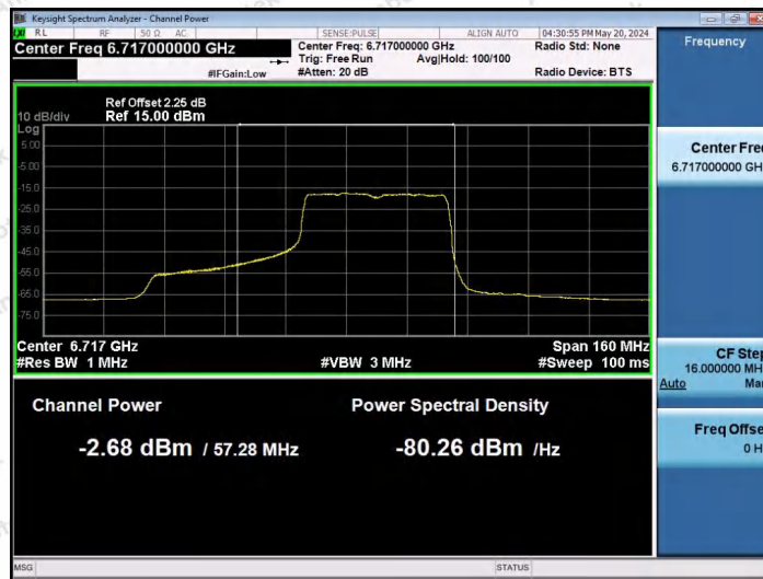
11AX80SISO-Ant1-6705-484Tone-RU66-PASS
