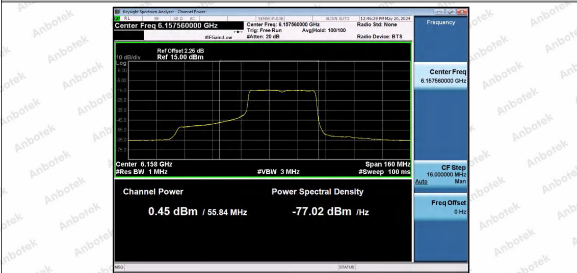
11AX80SISO-Ant1-6145-484Tone-RU66-PASS
