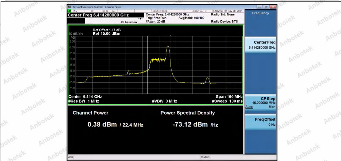
11AX80SISO-Ant1-6385-26Tone-RU36-PASS
