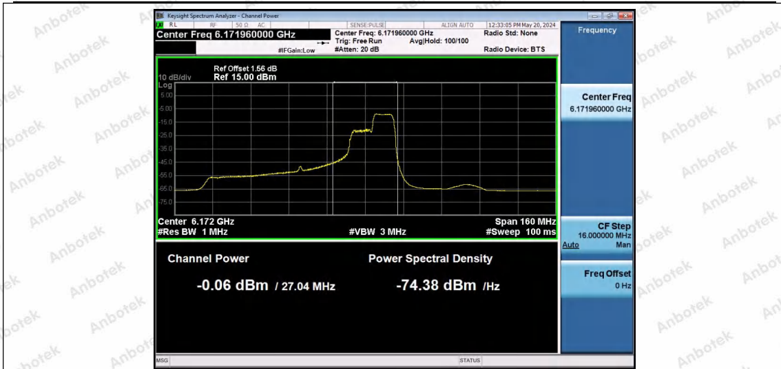
11AX80SISO-Ant1-6145-106Tone-RU60-PASS
