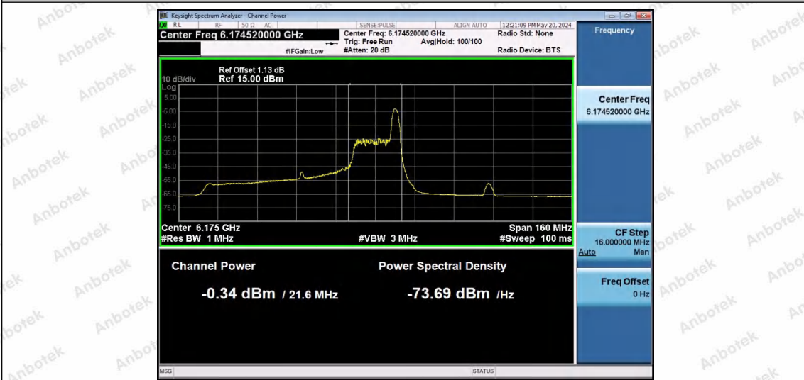
11AX80SISO-Ant1-6145-26Tone-RU36-PASS
