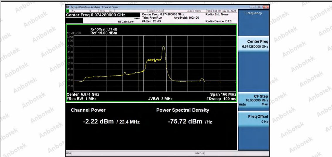
11AX80SISO-Ant1-6945-26Tone-RU36-PASS
