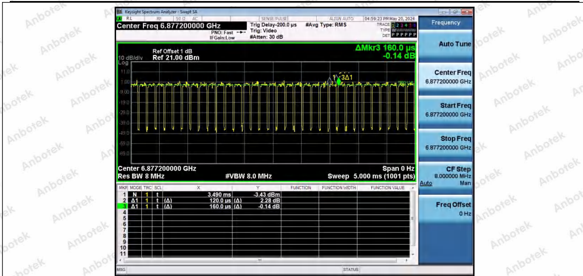
NTNV-11AX80SISO-Ant1-6865-484Tone-RU66
