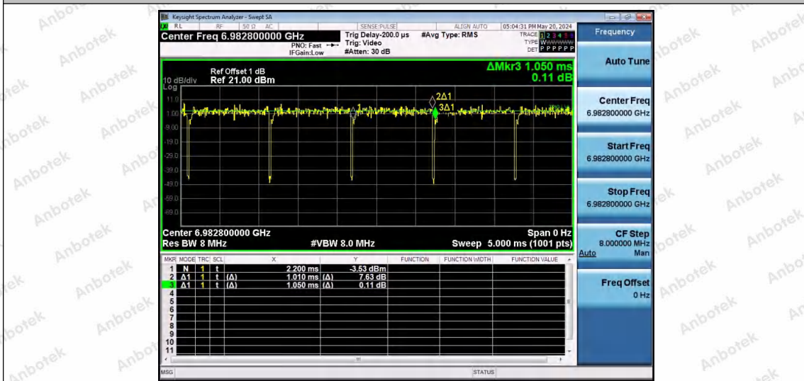
NTNV-11AX80SISO-Ant1-6945-26Tone-RU36
