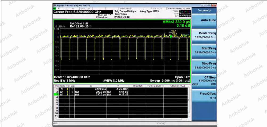
NTNV-11AX80SISO-Ant1-6865-106Tone-RU53
