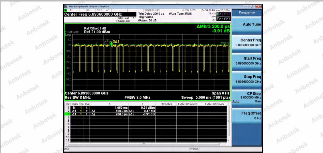
NTNV-11AX80SISO-Ant1-6865-242Tone-RU64
