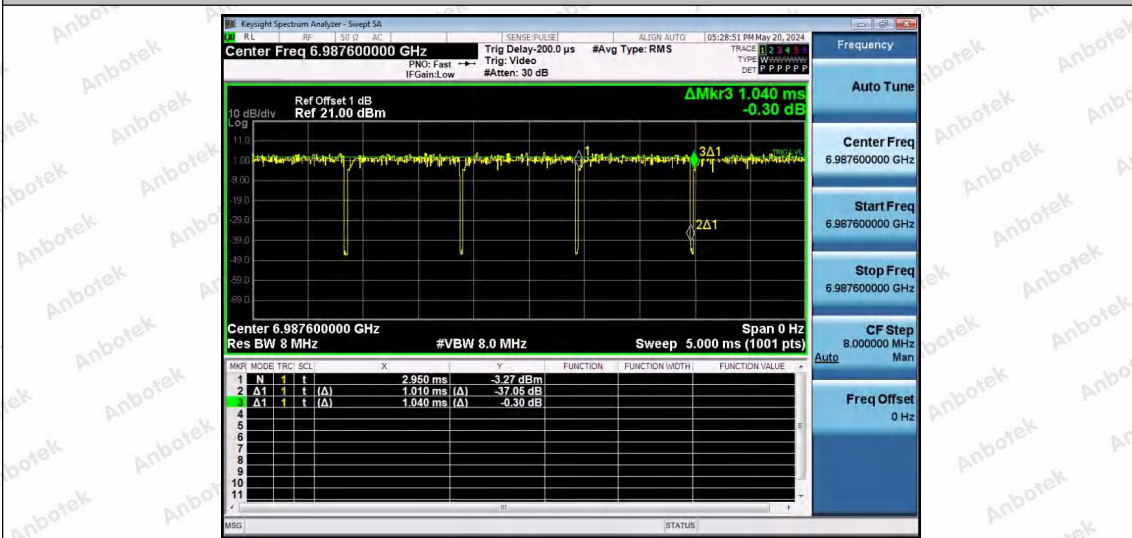
NTNV-11AX80SISO-Ant1-7025-26Tone-RU0
