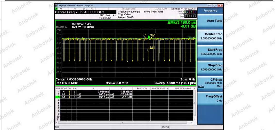
NTNV-11AX80SISO-Ant1-7025-242Tone-RU64
