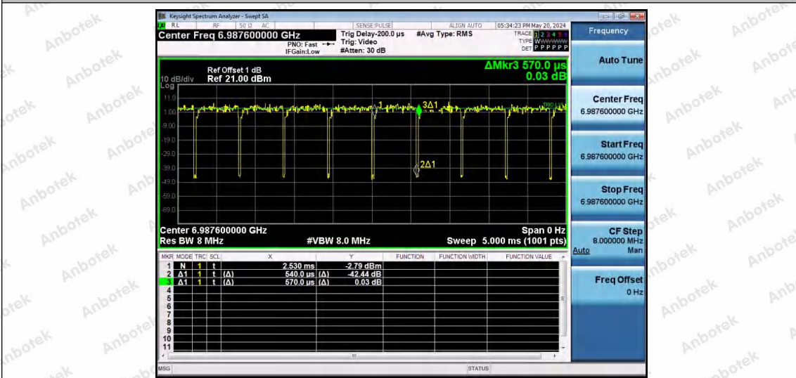
NTNV-11AX80SISO-Ant1-7025-52Tone-RU37
