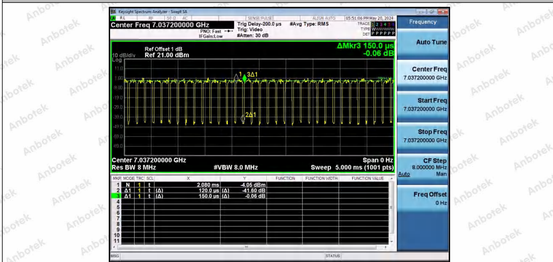
NTNV-11AX80SISO-Ant1-7025-484Tone-RU66
