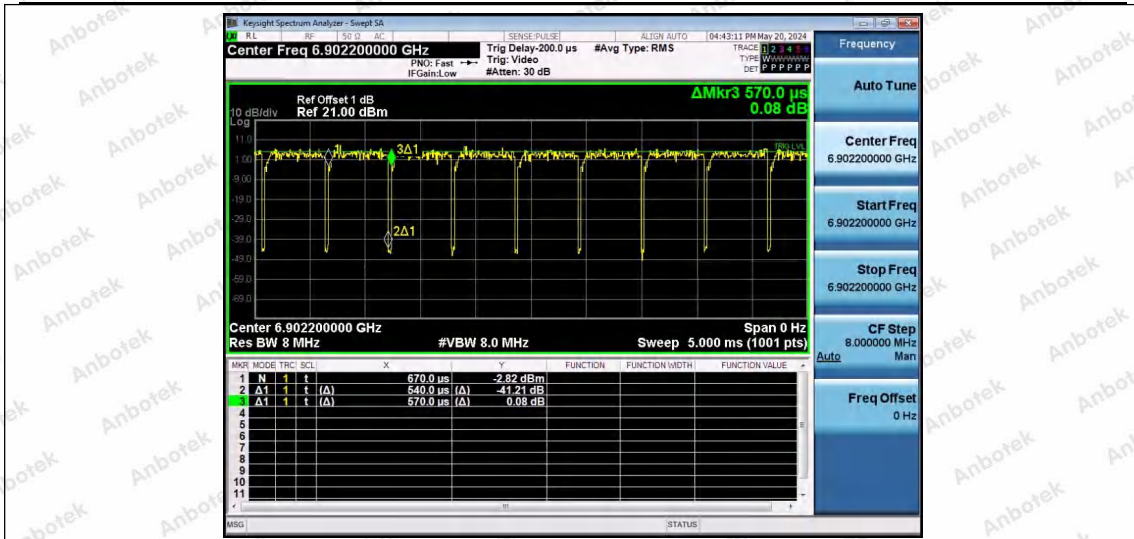
NTNV-11AX80SISO-Ant1-6865-52Tone-RU52
