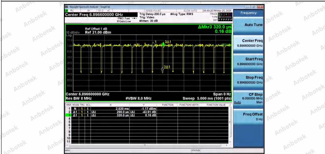
NTNV-11AX80SISO-Ant1-6865-106Tone-RU60
