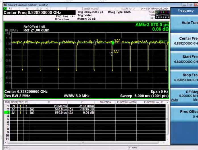
NTNV-11AX80SISO-Ant1-6865-52Tone-RU37
