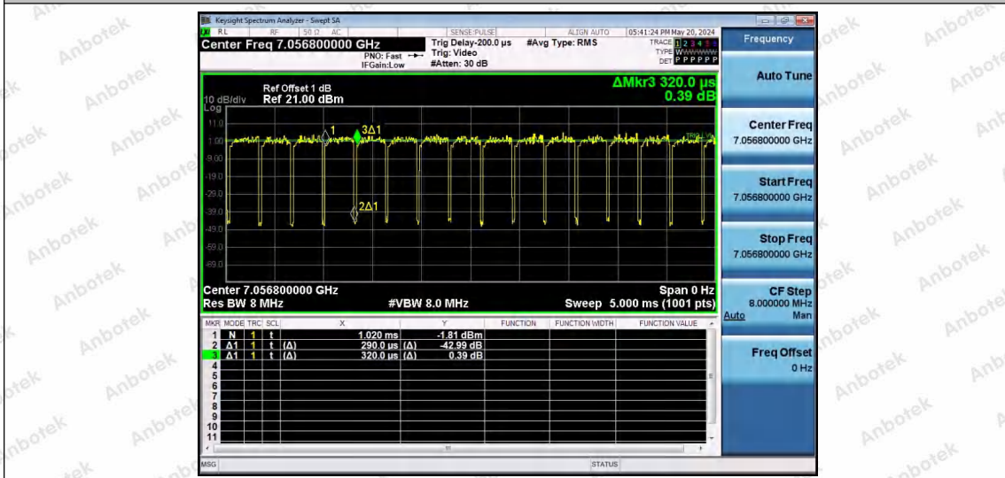
NTNV-11AX80SISO-Ant1-7025-106Tone-RU60
