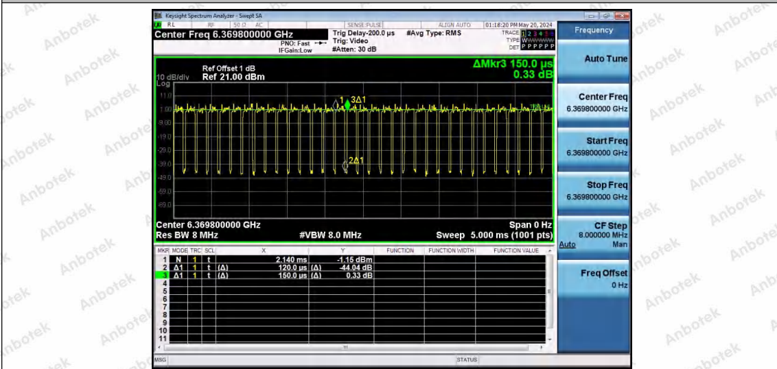
NTNV-11AX80SISO-Ant1-6385-484Tone-RU65
