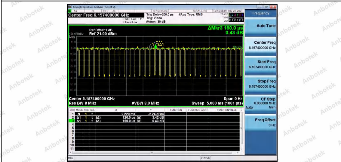
NTNV-11AX80SISO-Ant1-6145-484Tone-RU66
