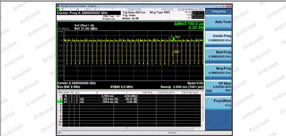
NTNV-11AX80SISO-Ant1-6385-484Tone-RU66
