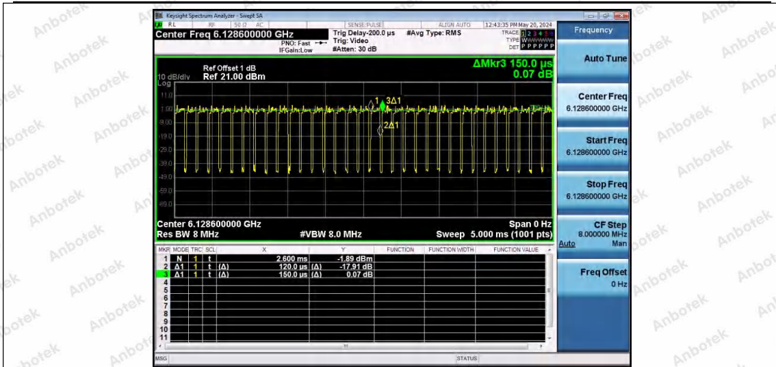
NTNV-11AX80SISO-Ant1-6145-484Tone-RU65
