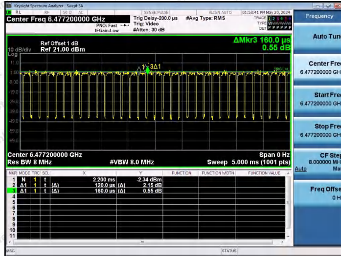
NTNV-11AX80SISO-Ant1-6465-484Tone-RU66
