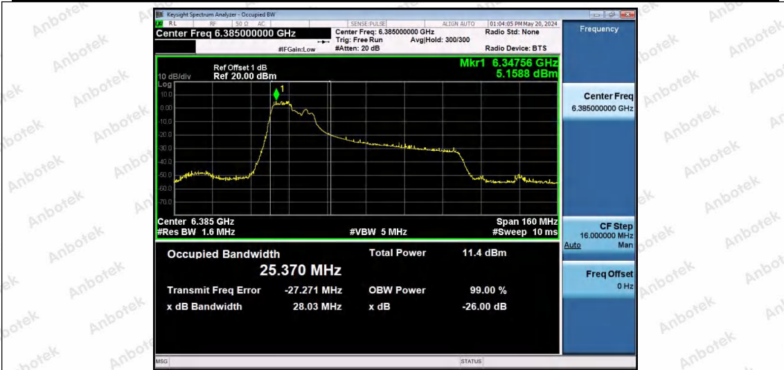
11AX80SISO-Ant1-6385-106Tone-RU53-PASS
