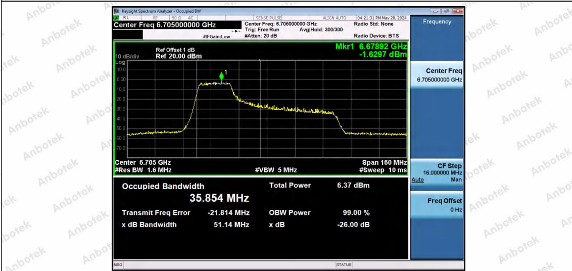
11AX80SISO-Ant1-6705-242Tone-RU61-PASS
