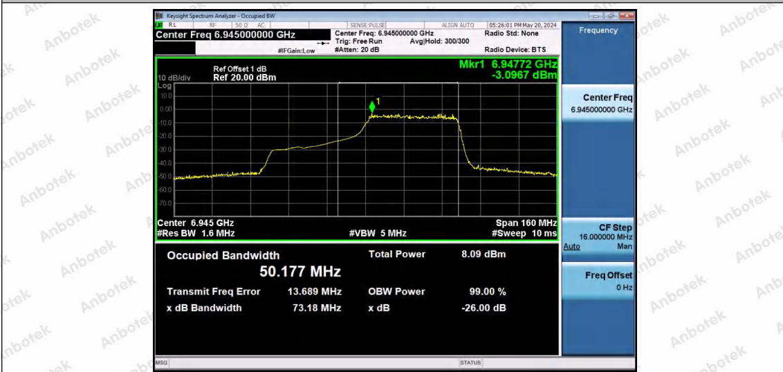
11AX80SISO-Ant1-6945-484Tone-RU66-PASS
