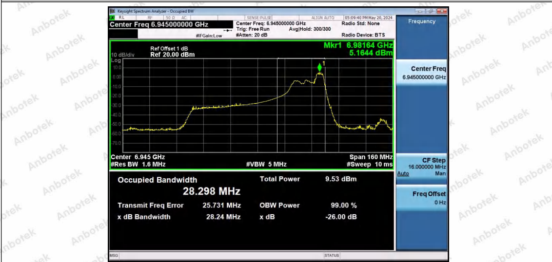
11AX80SISO-Ant1-6945-52Tone-RU52-PASS
