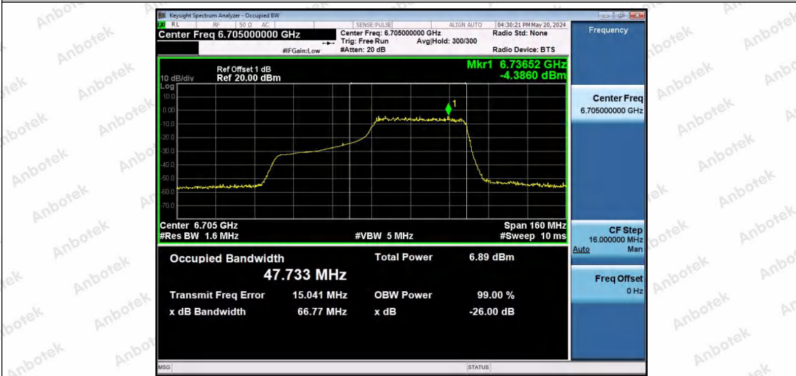
11AX80SISO-Ant1-6705-484Tone-RU66-PASS
