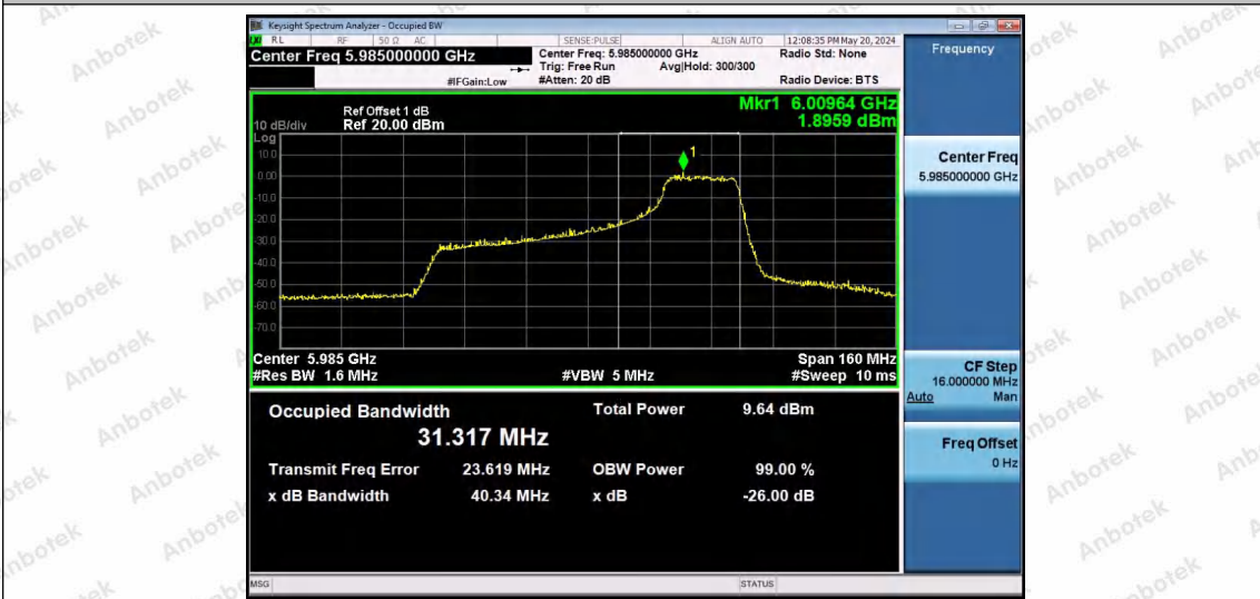
11AX80SISO-Ant1-5985-242Tone-RU64-PASS
