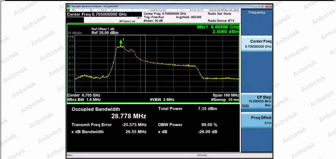
11AX80SISO-Ant1-6705-106Tone-RU53-PASS
