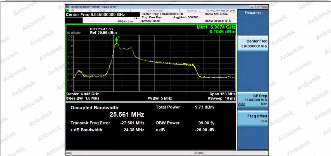
11AX80SISO-Ant1-6945-52Tone-RU37-PASS
