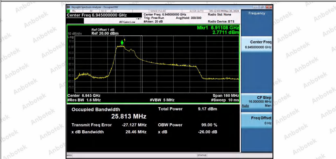
11AX80SISO-Ant1-6945-106Tone-RU53-PASS
